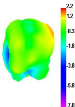
2450.000MHz H
