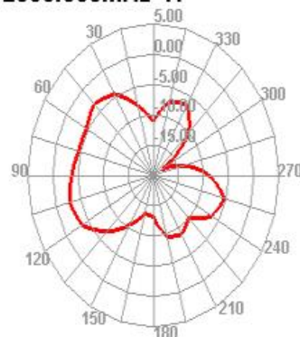
2500.000MHz H
