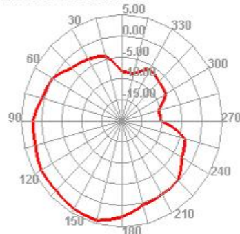
5850.000MHz H
