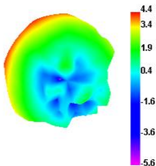
5500.000MHz H
