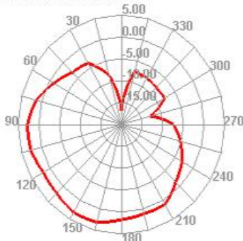
5150.000MHz H
