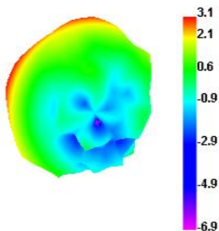
5150.000MHz H
