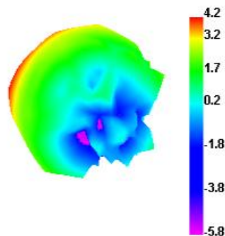
5850.000MHz H
