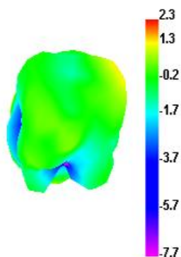
2400.000MHz H
