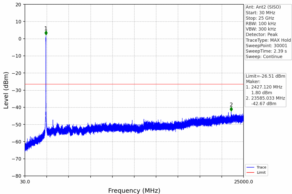
802.11n(HT40)_LCH_2422MHz_Ant2 (SISO)_NTNV
