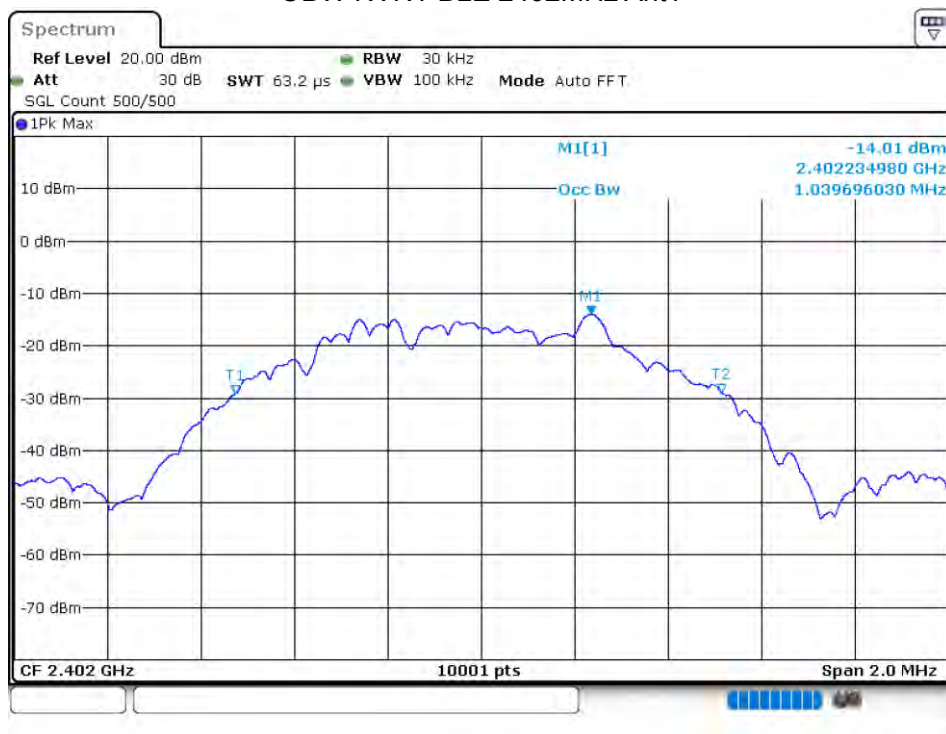
OBW NVNT BLE 2402MHz Ant1
