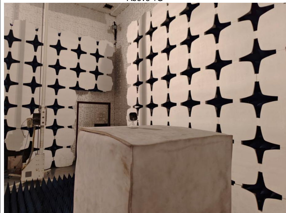
Above 1G
