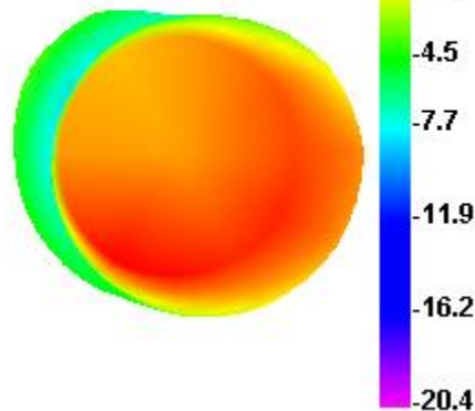
2450.000MHz E1
