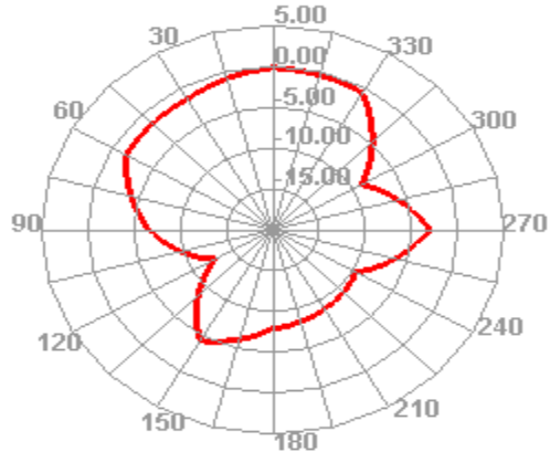
2400.000MHz E1
