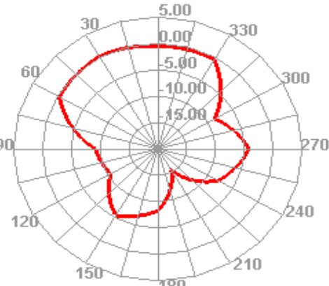
2450.000MHz E1
