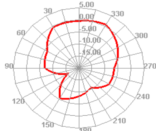
2450.000MHz E2
