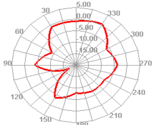
2400.000MHz E2
