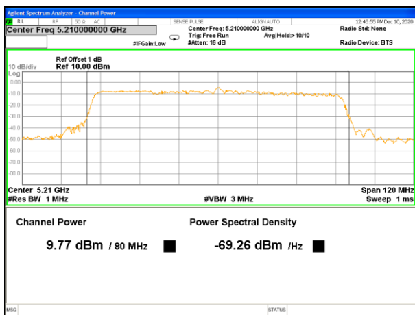
5210MHz_ANT 4
