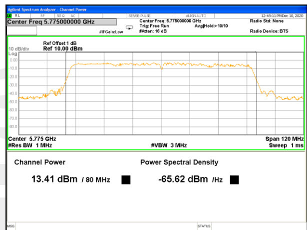
5775MHz_ANT 4
