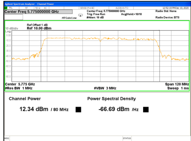
5775MHz_ANT 3
