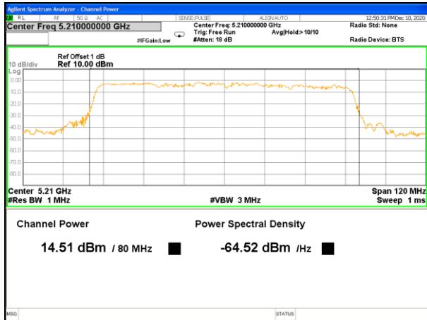
5210MHz_ANT 3
