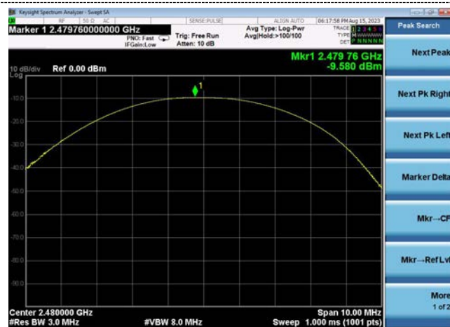
GFSK(CH78)
