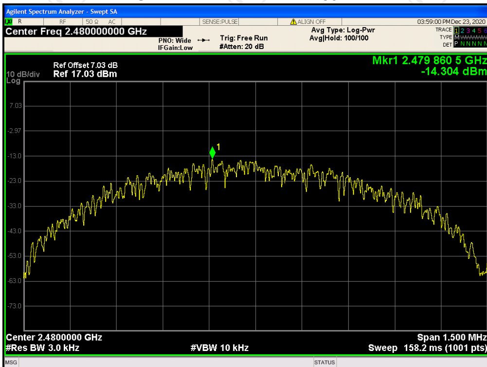
PSD NVNT BLE 1M PHY 2480MHz
