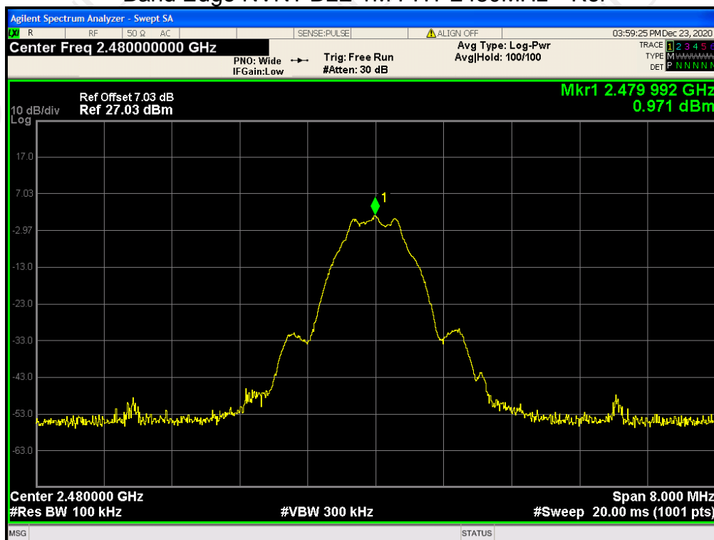
Band Edge NVNT BLE 1M PHY 2480MHz Emission
