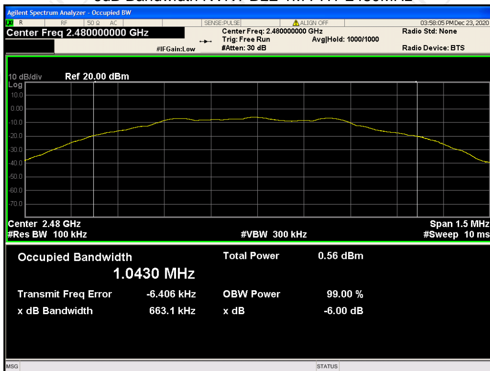
-6dB Bandwidth NVNT BLE 1M PHY 2480MHz
