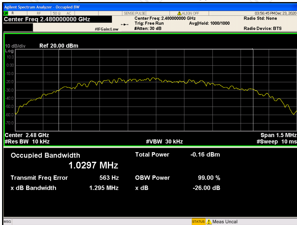
OBW NVNT BLE 1M PHY 2480MHz
