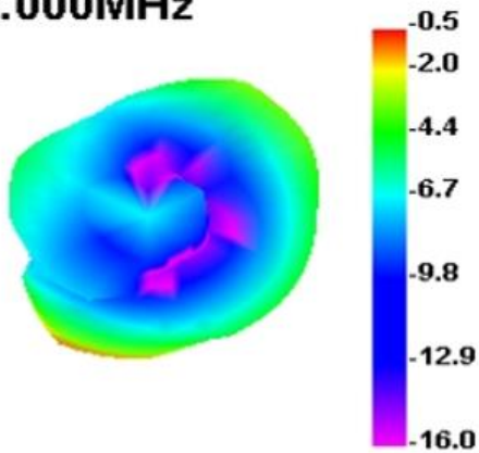
2450.000MHz
