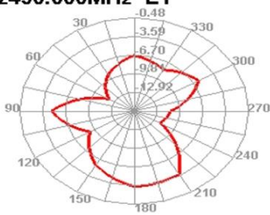
2450.000MHz E1
