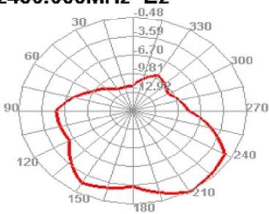
2450.000MHz E2
