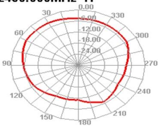
2450.000MHz H
