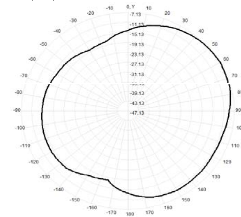
Total(H-XY), Max=-7.13dBi, CirD=11.37
