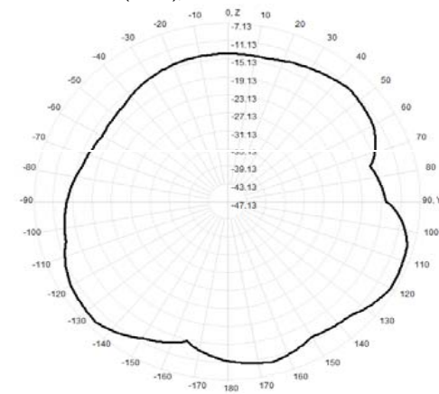
928.0MHz Total(E2-YZ), Max=-8.19dBi
