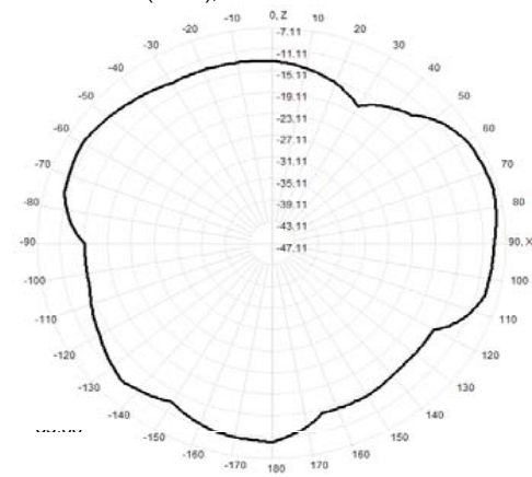
929.0MHz Total(E1-XZ), Max=-8.10dBi
