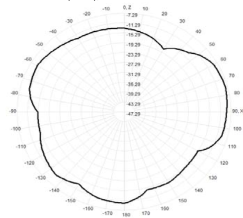
927.0MHz Total(E1-XZ), Max=-8.29dBi
