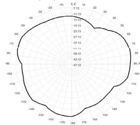
928.0MHz Total(E1-XZ), Max=-8.14dBi
