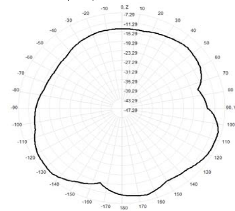
927.0MHz Total(E2-YZ), Max=-8.77dBi
