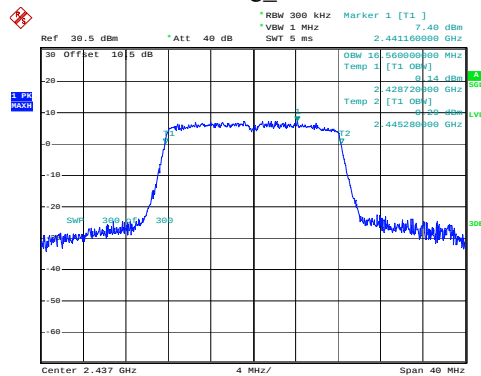
802.11g_2437MHz
