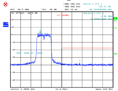
802.11n20_2462MHz
