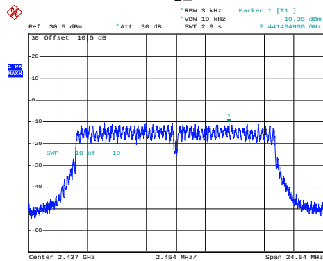
802.11g_2437MHz
