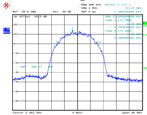
802.11b_2462MHz
