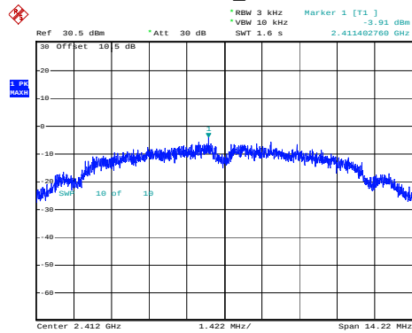
802.11b_2412MHz
