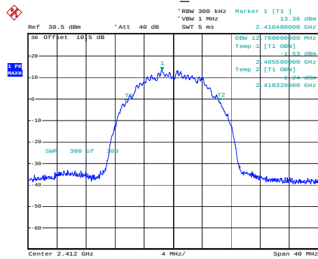
802.11b_2412MHz
