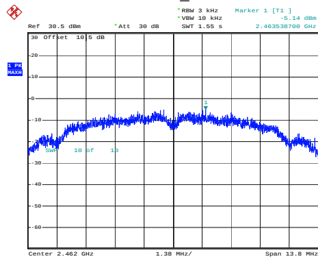
802.11b_2462MHz
