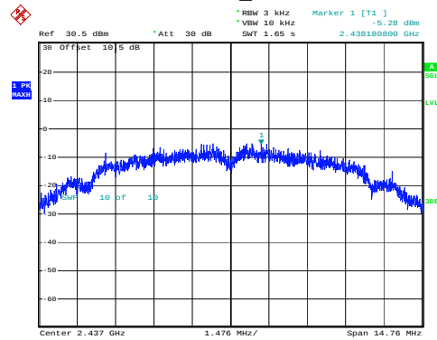
802.11b_2437MHz
