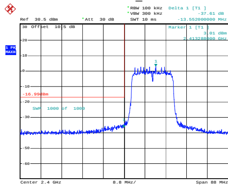
802.11n20_2412MHz
