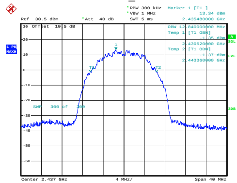
802.11b_2437MHz
