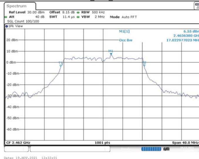
11G_Ant2_2462
