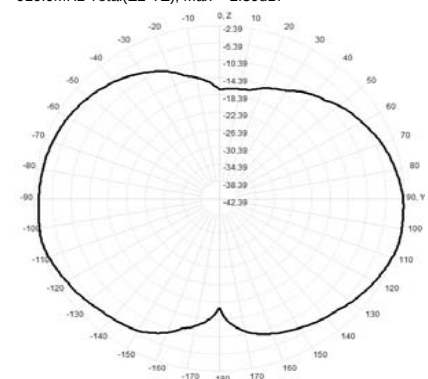
910.0MHz Total(E2-YZ), Max= -2.39dBi
