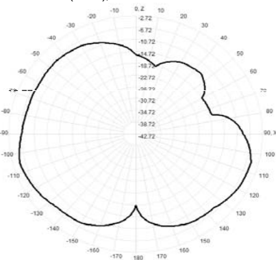
915.0MHz Total(E1-XZ), Max= -4.95dBi
