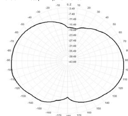
926.0MHz Total(E2-YZ), Max= -3.49dBi
