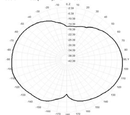
908.0MHz Total(E2-YZ), Max= -2.39dBi
