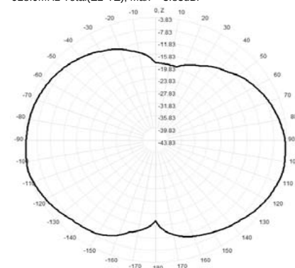
928.0MHz Total(E2-YZ), Max= -3.83dBi
