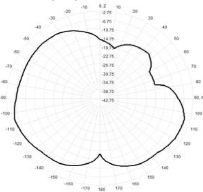
916.0MHz Total(E1-XZ), Max= -5.08dBi
