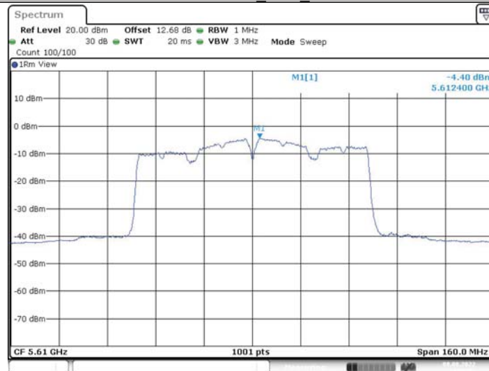
11AC80SISO_Ant1_5610
