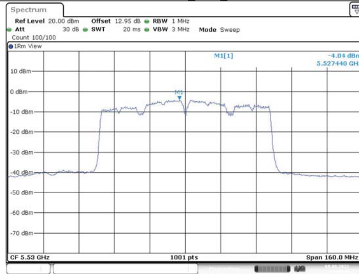
11AC80SISO_Ant1_5530
