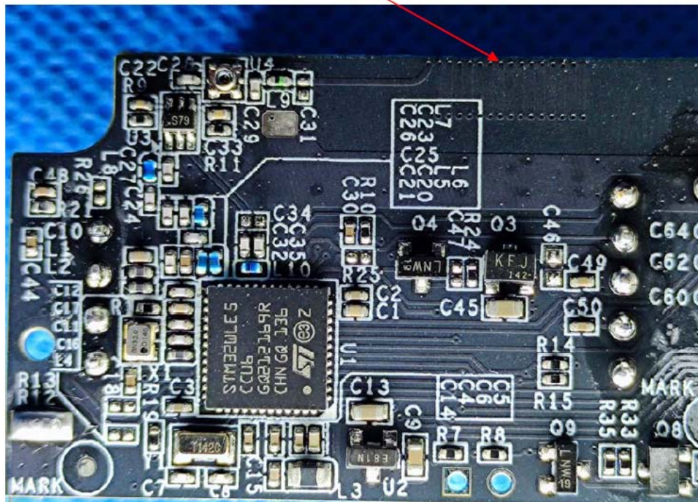
NFC Passive Antenna
