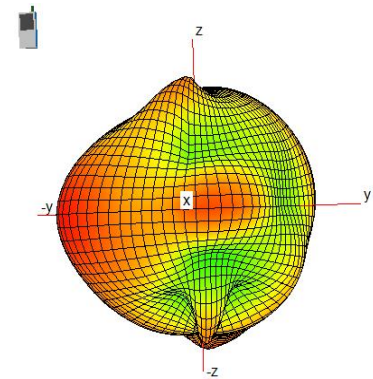
5800MHz
