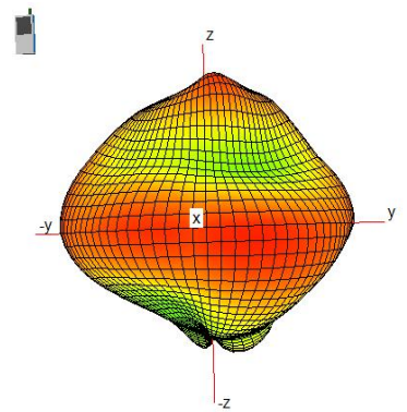
2500MHz
