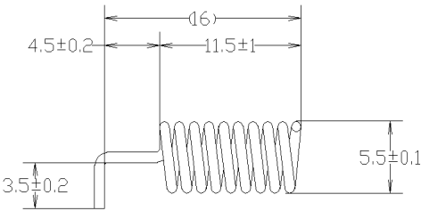
GBT-915-3.5-01 弹簧天线，线径0.8mm，圈数9，材质磷铜
