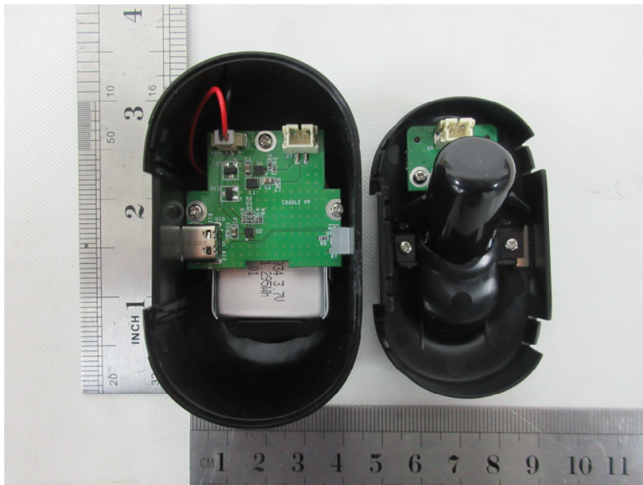
Cradle_Internal photo
