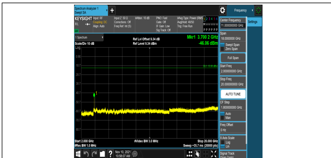
Band2-3MHz-QPSK-18615-1RB#0-Range5:2000~20000MHz
