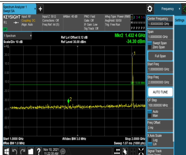
Band2-5MHz-QPSK-19175-1RB#0-Range4:1000~2000MHz
