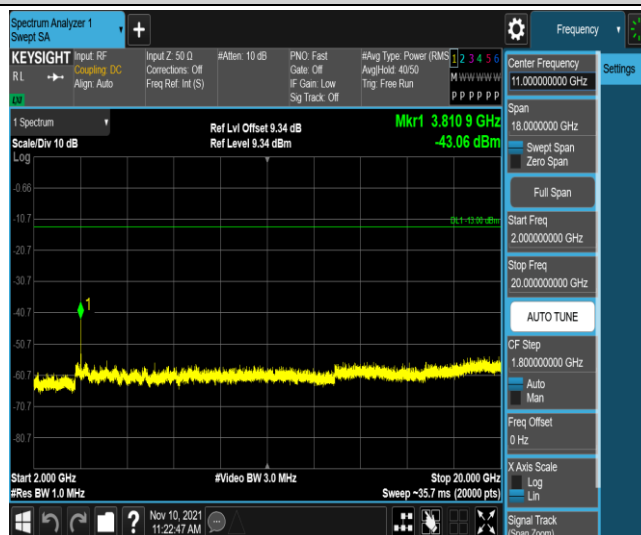
Band2-5MHz-QPSK-19175-1RB#0-Range5:2000~20000MHz
