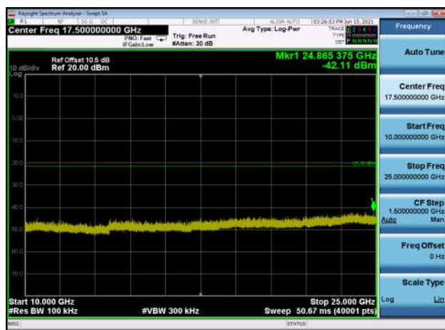
,Plot 5,10000MHz~25000MHz-802.11g ,2437MHz
