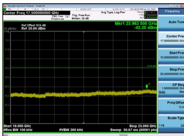
,Plot 5,10000MHz~25000MHz-802.11n(HT2 0),2437MHz
