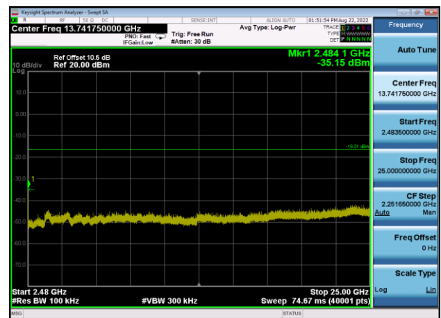
,Plot 4,2483.5MHz~25000MHz-802.11n(HT20),2462MHz,Ant0
