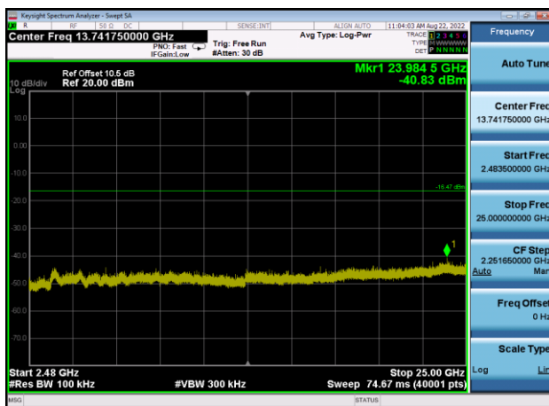
,Plot 4,2483.5MHz~25000MHz-802.11n(HT20),2437MHz,Ant0
