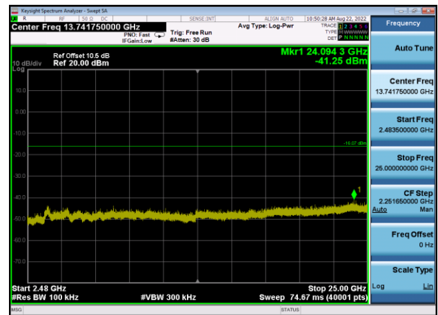
,Plot 4,2483.5MHz~25000MHz-802.11n(HT20),2462MHz,Ant0
