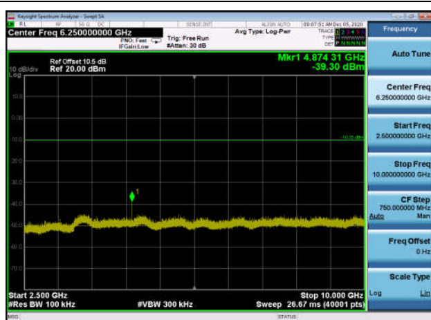
,Plot 4,2500MHz~10000MHz-802.11b
