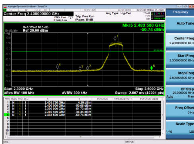
,Plot 2,Band Edge-802.11n(HT20) ,2437MHz,Ant0
