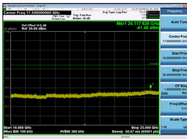
,Plot 5,10000MHz~25000MHz-802.11g ,2462MHz,Ant0
