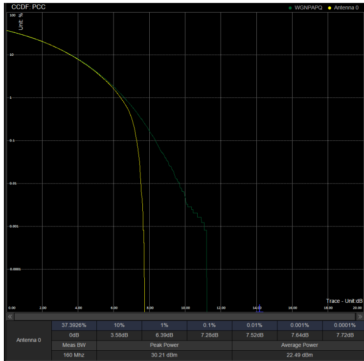
PAPR/PC2\N78(3450-3550)\90M CP 633000 100%RB 16QAM
