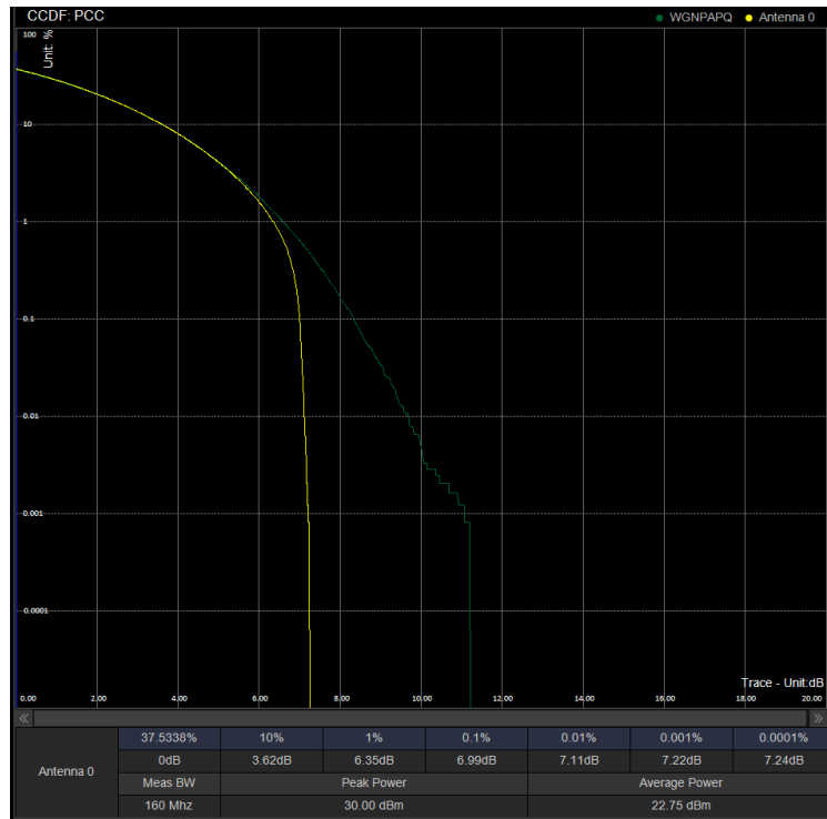
PAPR/PC2\N78(3450-3550)\60M CP 632000 100%RB 256QAM
