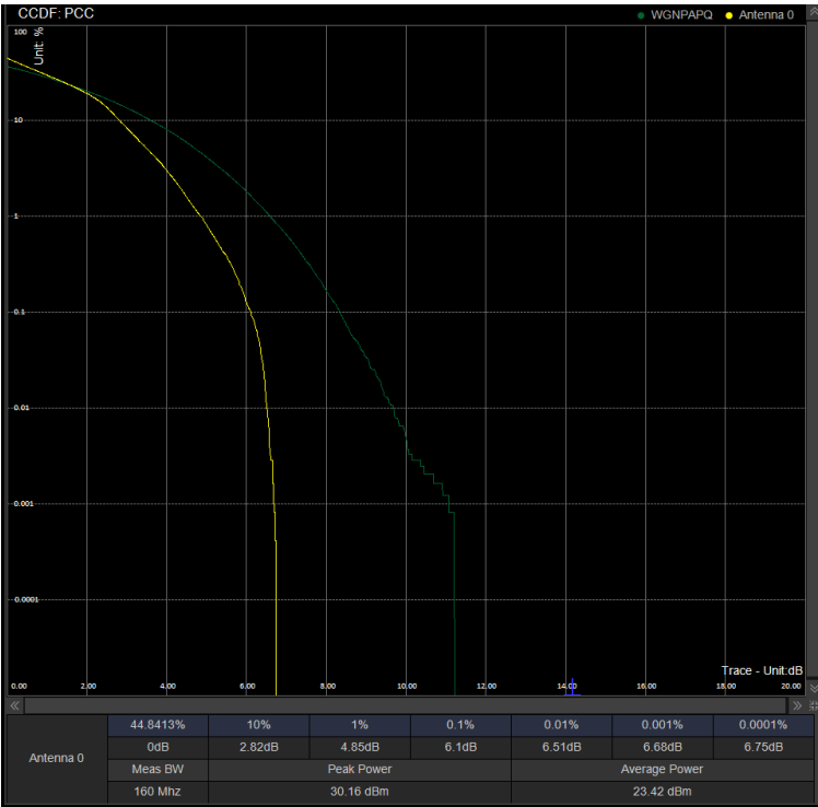
PAPR/PC2\N78(3450-3550)\70M DFT 634332 100%RB 16QAM
