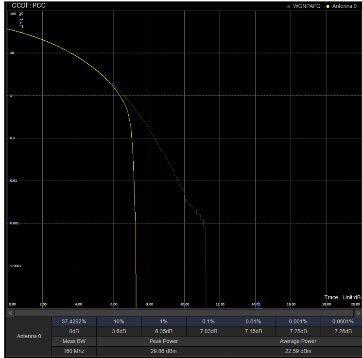
PAPR/PC2\N78(3450-3550)\60M CP 634666 100%RB 64QAM
