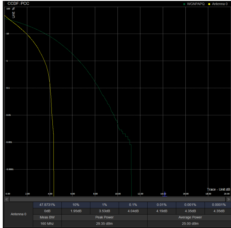
PAPR/PC2\N78(3450-3550)\70M DFT 634332 100%RB BPSK
