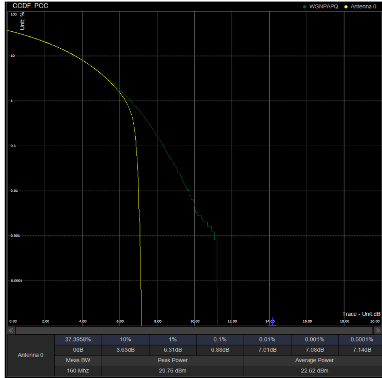
PAPR/PC2\N78(3450-3550)\60M CP 634666 100%RB 16QAM
