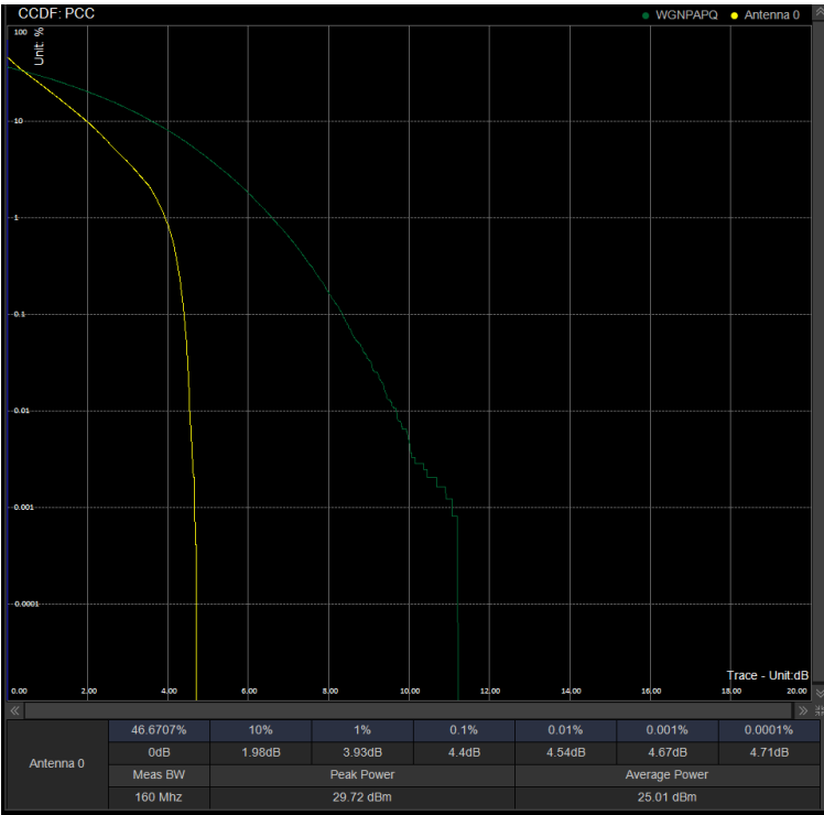
PAPR/PC2\N78(3450-3550)\50M DFT 635000 100%RB QPSK
