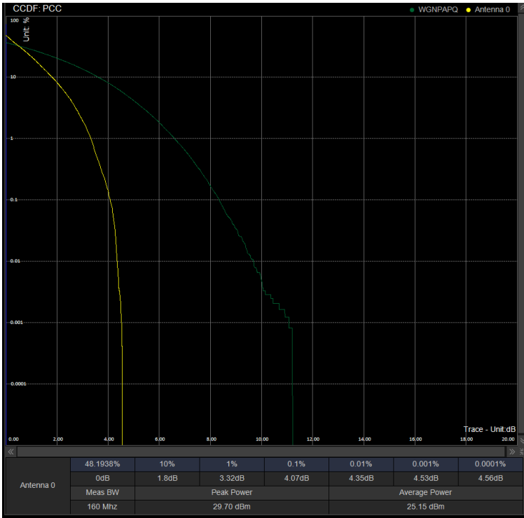
PAPR/PC2\N78(3450-3550)\60M DFT 633334 100%RB QPSK
