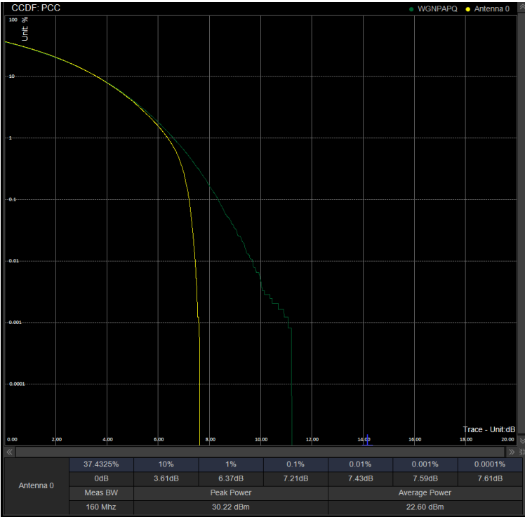
PAPR/PC2\N78(3450-3550)\90M CP 633334 100%RB QPSK
