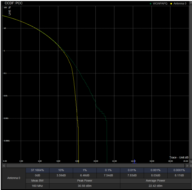
PAPR/PC2\N78(3450-3550)\80M CP 634000 100%RB 256QAM
