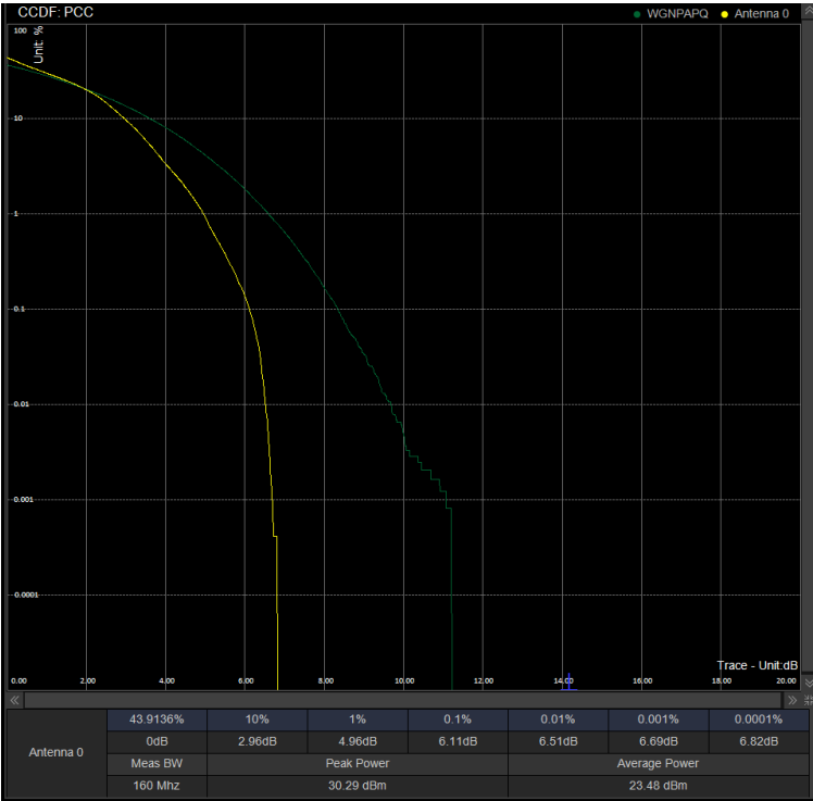
PAPR/PC2\N78(3450-3550)\80M DFT 632668 100%RB 16QAM
