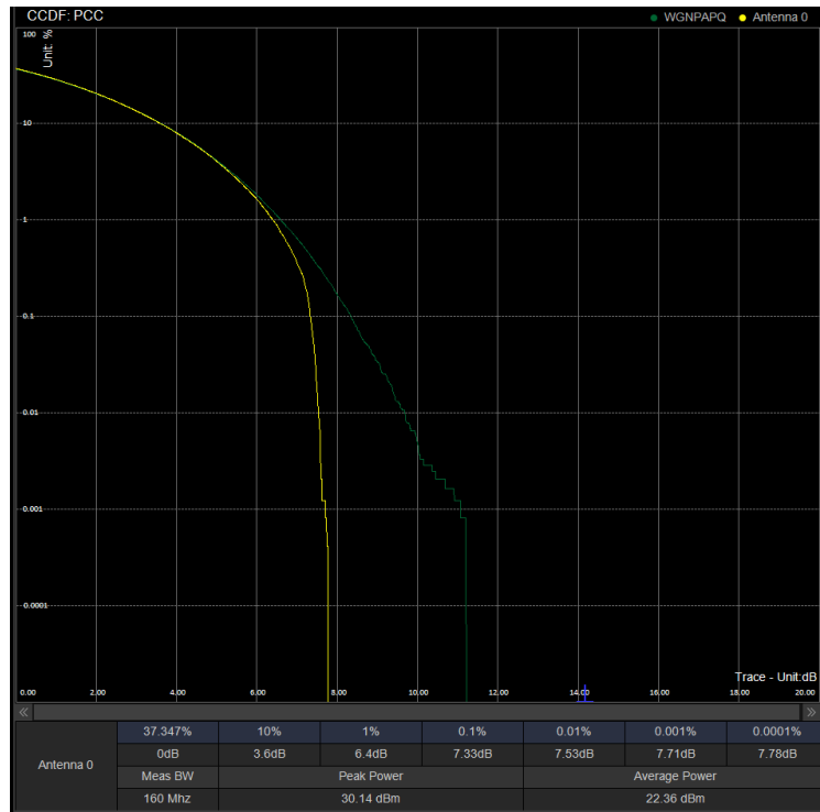
PAPR/PC2\N78(3450-3550)\70M CP 634332 100%RB 16QAM
