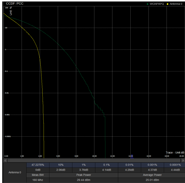
PAPR/PC2\N78(3450-3550)\80M DFT 632668 100%RB BPSK
