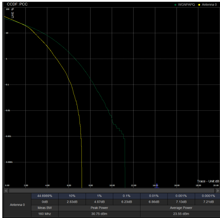
PAPR/PC2\N78(3450-3550)\70M DFT 632334 100%RB 16QAM
