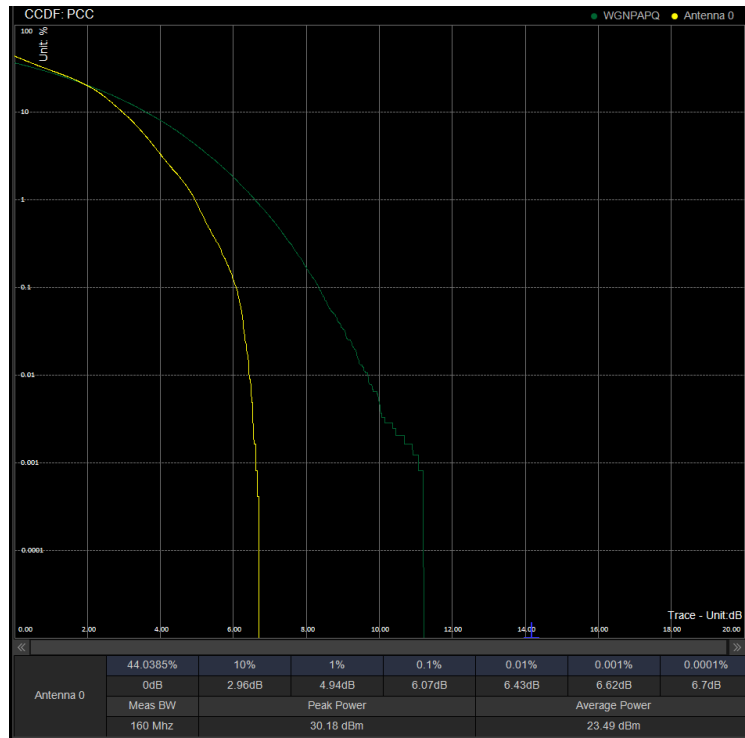
PAPR/PC2\N78(3450-3550)\80M DFT 633334 100%RB 16QAM
