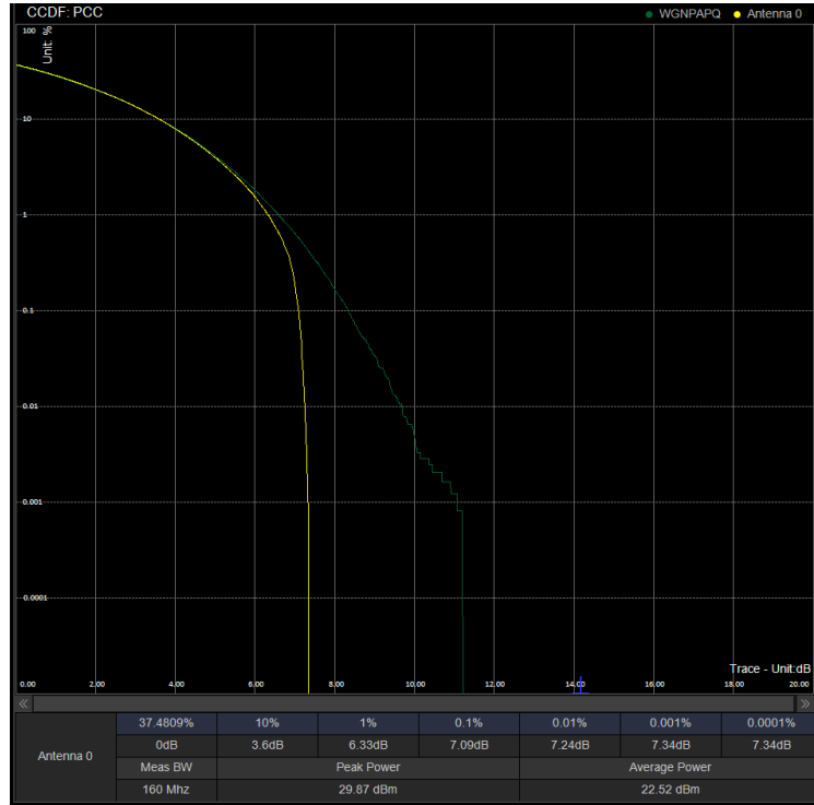
PAPR/PC2\N78(3450-3550)\70M CP 633334 100%RB QPSK
