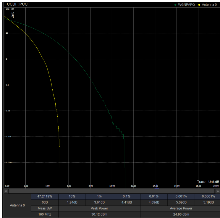
PAPR/PC2\N78(3450-3550)\70M DFT 633334 100%RB BPSK
