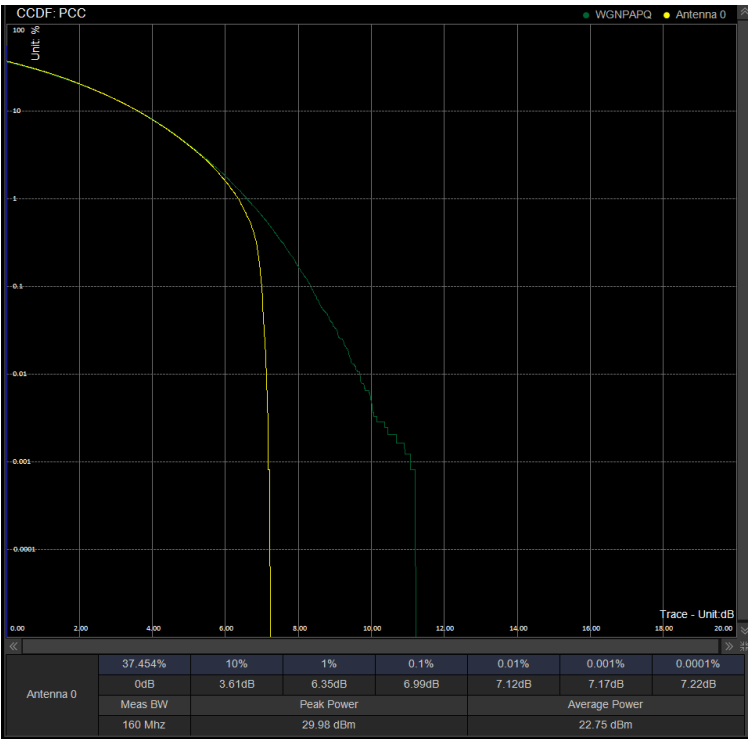
PAPR/PC2\N78(3450-3550)\60M CP 632000 100%RB 64QAM
