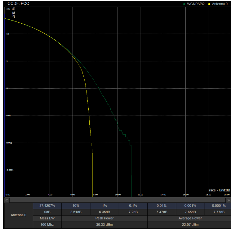
PAPR/PC2\N78(3450-3550)\90M CP 633666 100%RB QPSK
