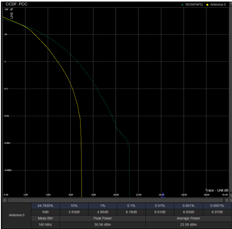
PAPR/PC2\N78(3450-3550)\70M DFT 633334 100%RB 16QAM
