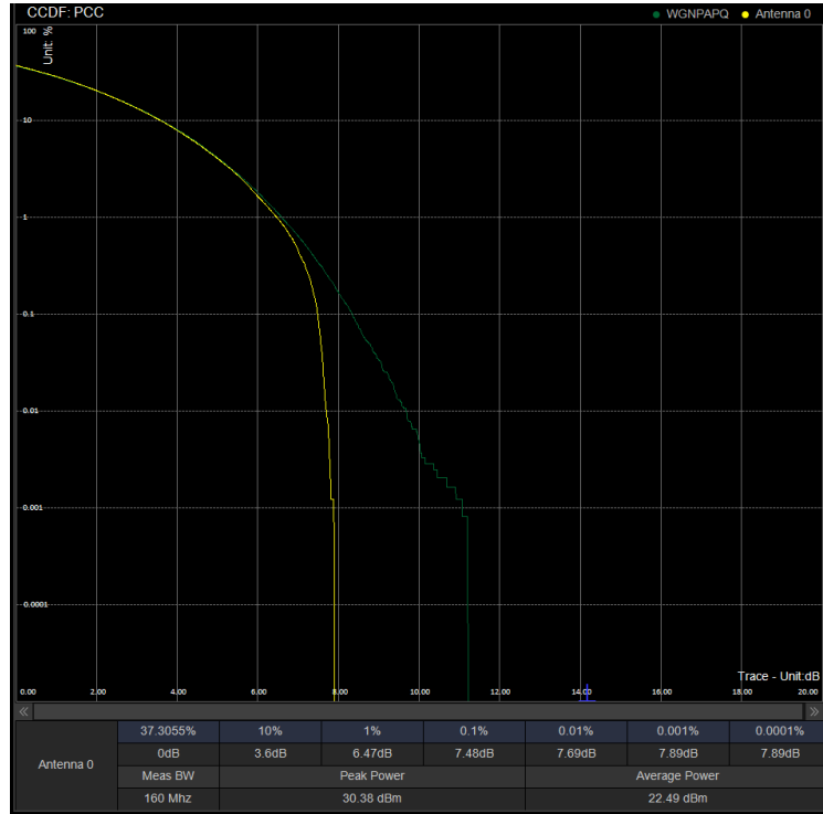
PAPR/PC2\N78(3450-3550)\80M CP 633334 100%RB 64QAM
