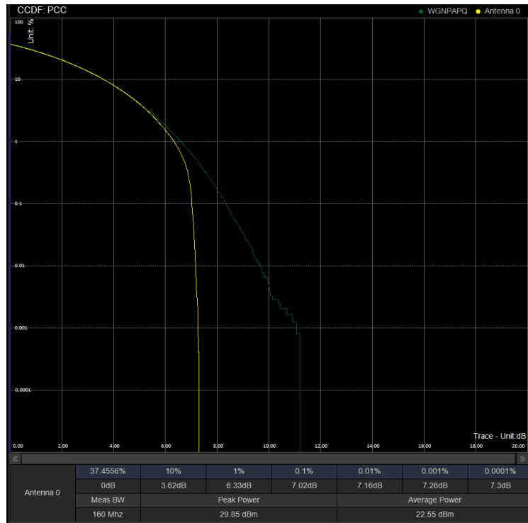
PAPR/PC2\N78(3450-3550)\60M CP 633334 100%RB QPSK
