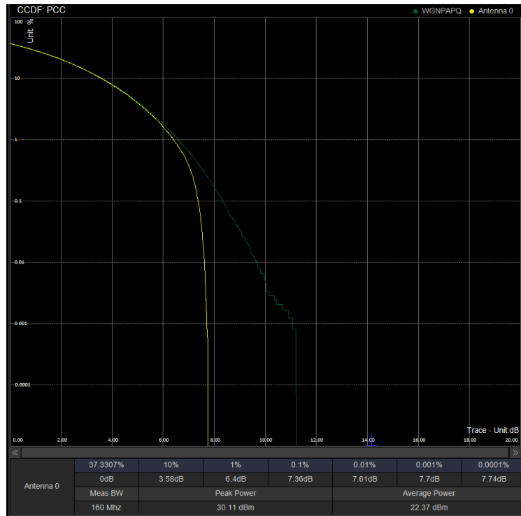
PAPR/PC2/N78(3450-3550)\90M CP 633334 100%RB 16QAM
