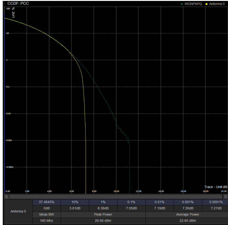
PAPR/PC2\N78(3450-3550)\60M CP 633334 100%RB 64QAM
