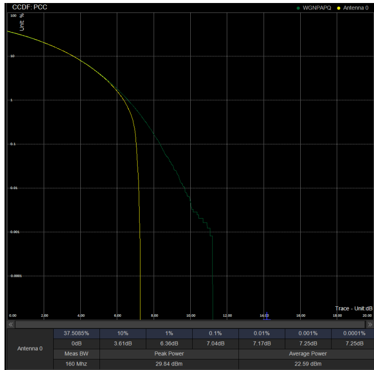
PAPR/PC2\N78(3450-3550)\60M CP 634666 100%RB 256QAM
