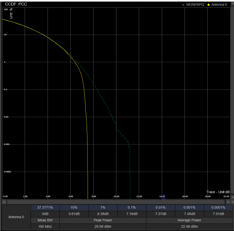
PAPR/PC2/N78(3450-3550)\70M CP 632334 100%RB QPSK
