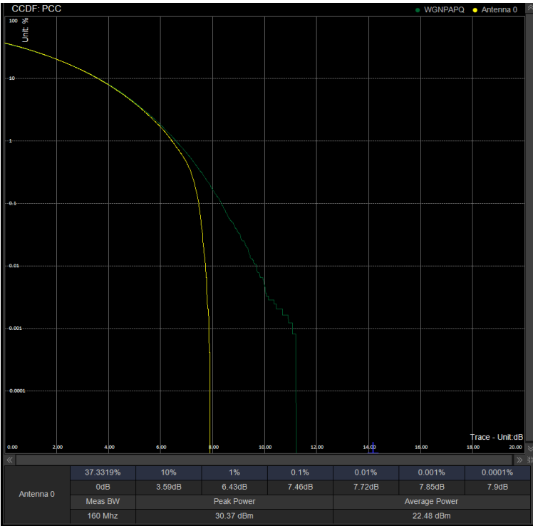
PAPR/PC2\N78(3450-3550)\80M CP 632668 100%RB QPSK
