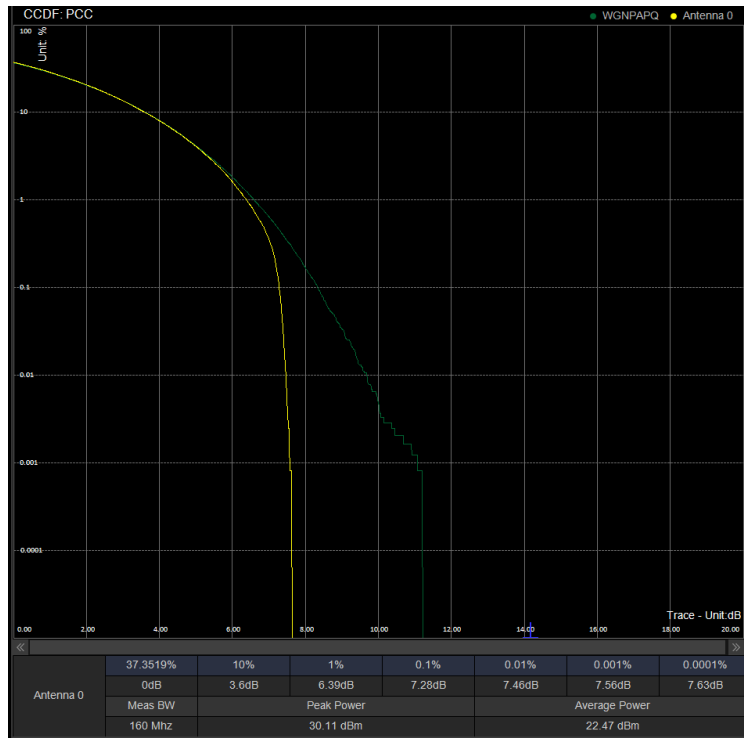
PAPR/PC2\N78(3450-3550)\70M CP 632334 100%RB 16QAM
