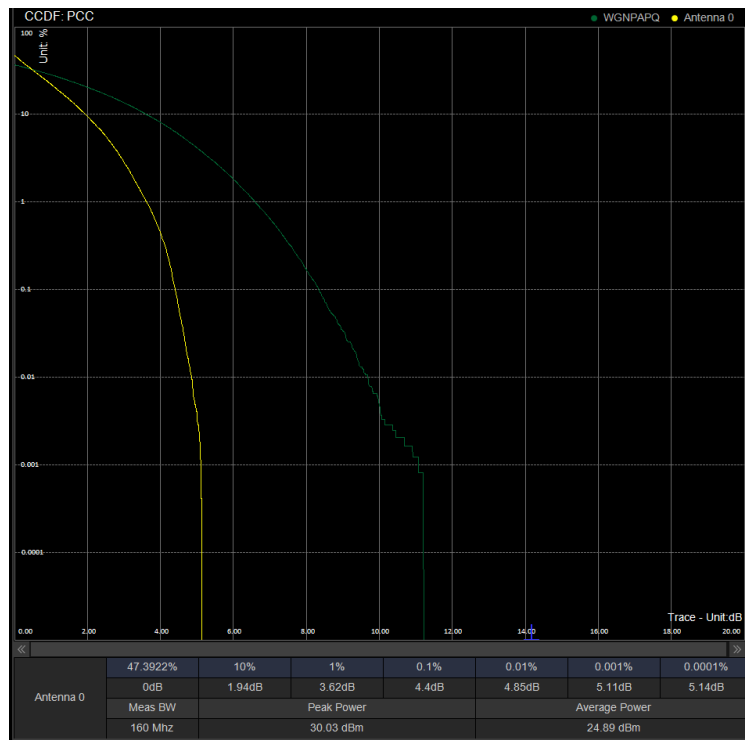
PAPR/PC2\N78(3450-3550)\70M DFT 634332 100%RB QPSK
