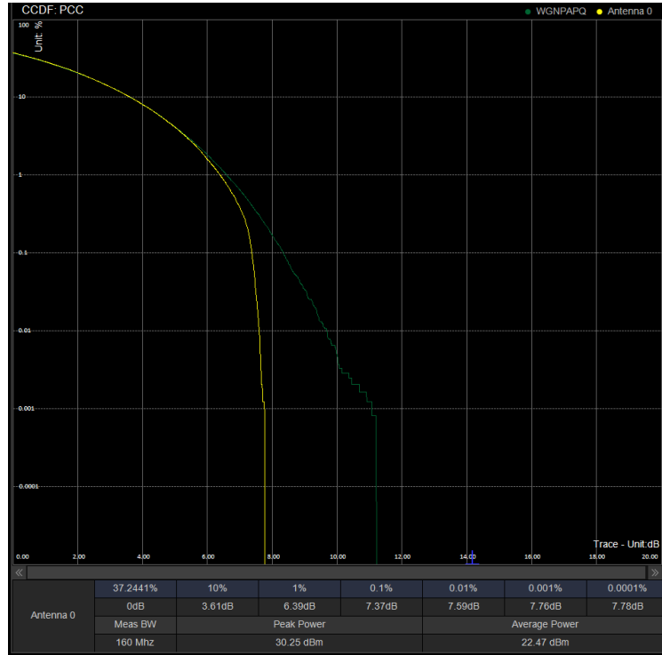
PAPR/PC2\N78(3450-3550)\80M CP 633334 100%RB 16QAM
