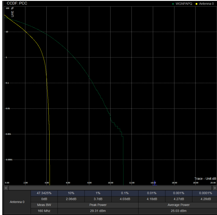
PAPR/PC2\N78(3450-3550)\80M DFT 633334 100%RB BPSK
