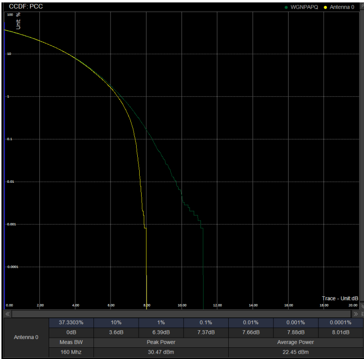
PAPR/PC2\N78(3450-3550)\90M CP 633666 100%RB 256QAM
