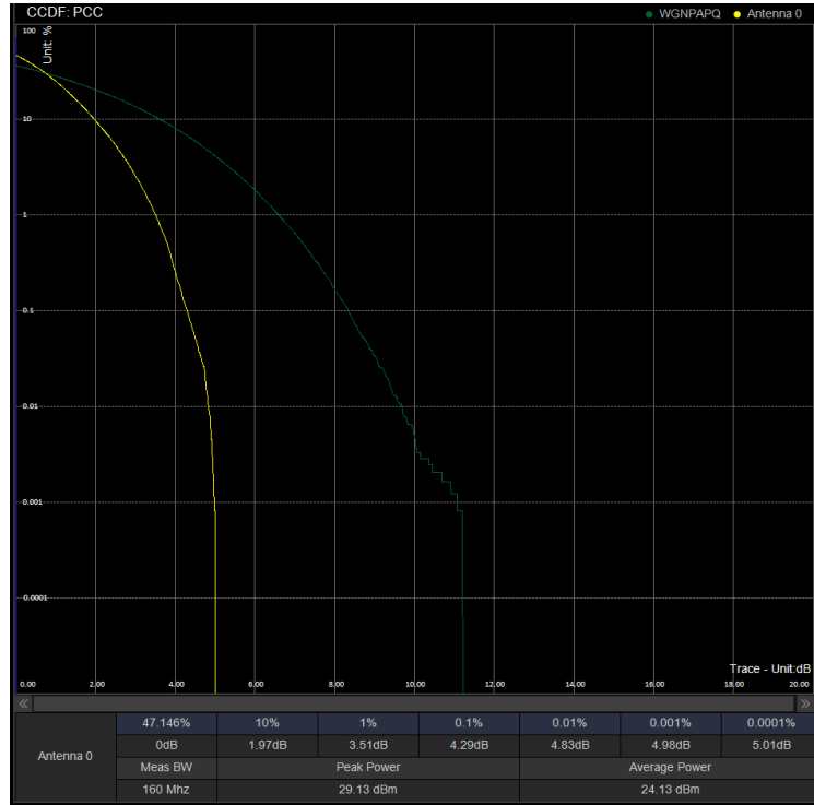
PAPR/PC2\N41\60M DFT 518598 100%RB QPSK
