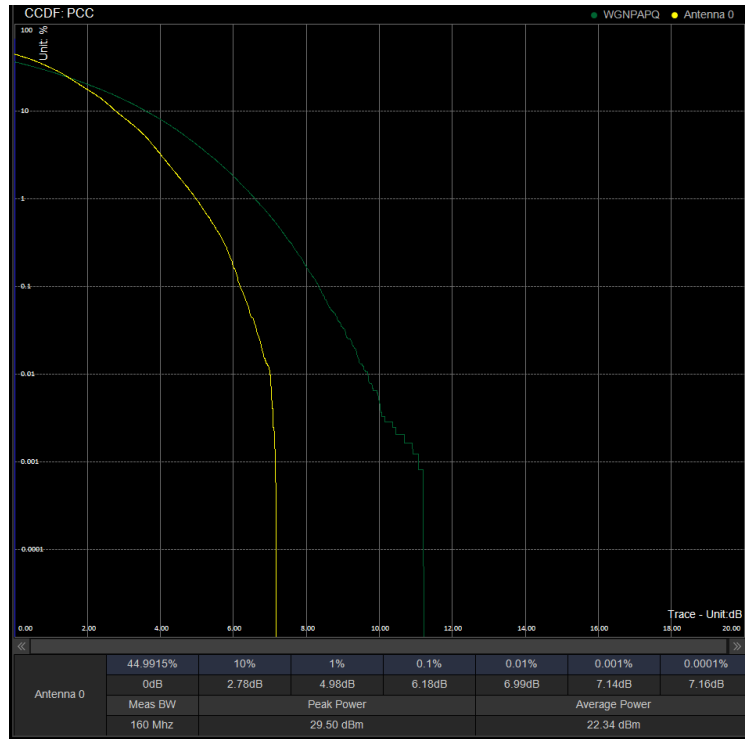
PAPR/PC2\N41\30M DFT 534996 100%RB 64QAM
