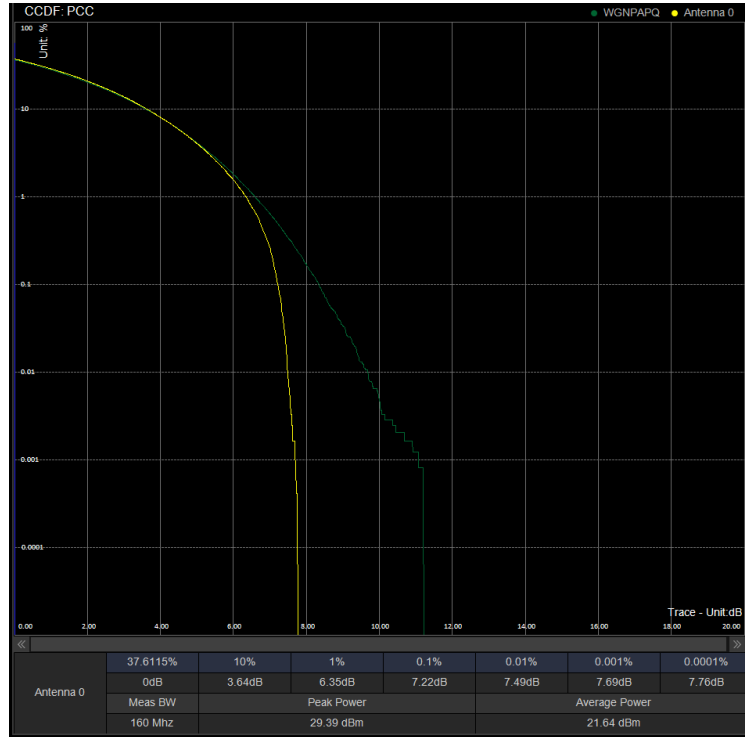
PAPR/PC2\N41\60M CP 518598 100%RB 256QAM
