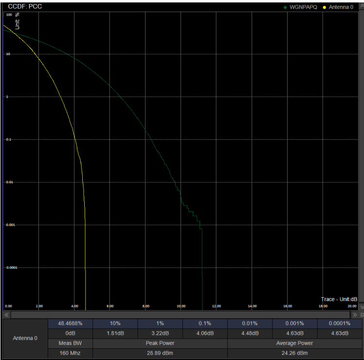
PAPR/PC2\N41\30M DFT 518598 100%RB BPSK
