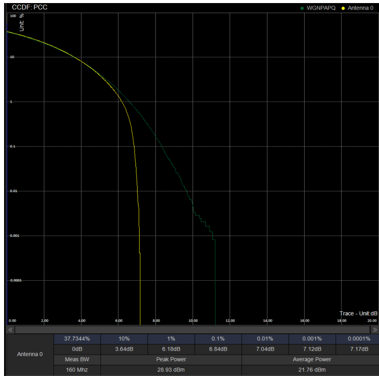
PAPR/PC2\N41\40M CP 518598 100%RB 16QAM
