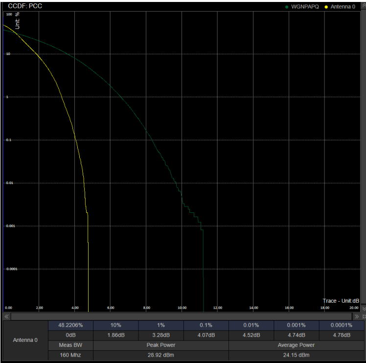
PAPR/PC2\N41\60M DFT 531996 100%RB QPSK
