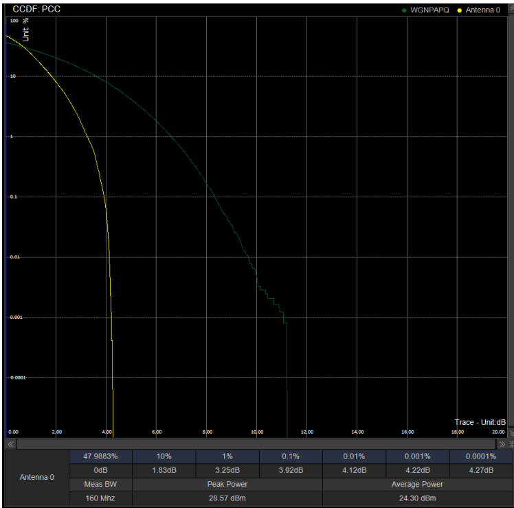
PAPR/PC2\N41\60M DFT 505200 100%RB BPSK
