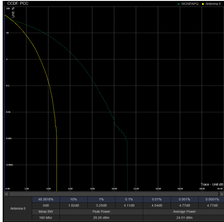
PAPR/PC2\N41\30M DFT 502200 100%RB QPSK
