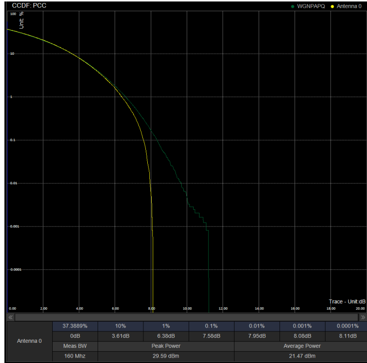
PAPR/PC2\N41\70M CP 506202 100%RB 64QAM
