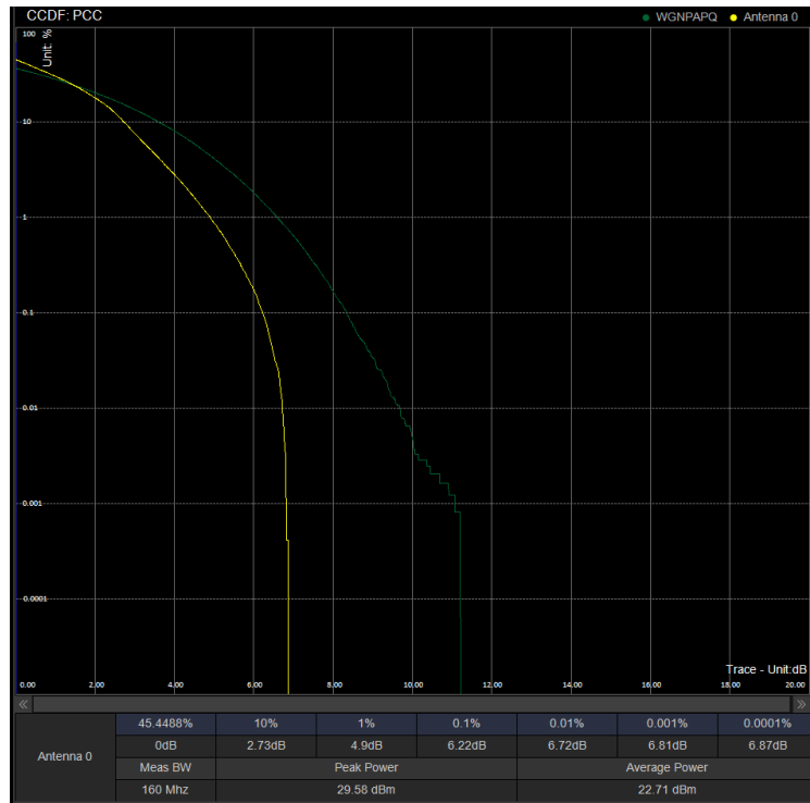
PAPR/PC2\N41\30M DFT 518598 100%RB 16QAM
