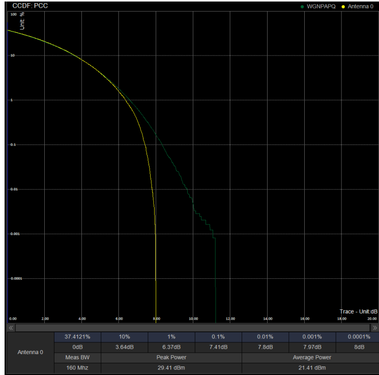
PAPR/PC2\N41\70M CP 518598 100%RB 16QAM
