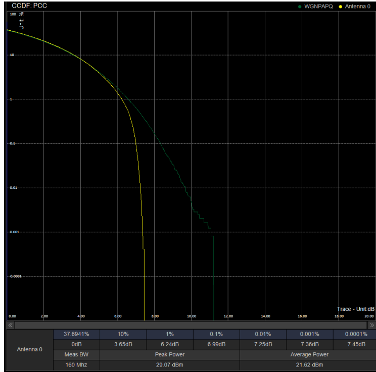
PAPR/PC2\N41\50M CP 518598 100%RB 16QAM
