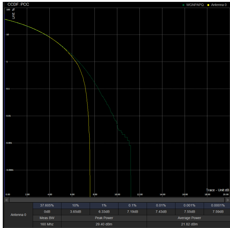
PAPR/PC2\N41\60M CP 505200 100%RB 64QAM
