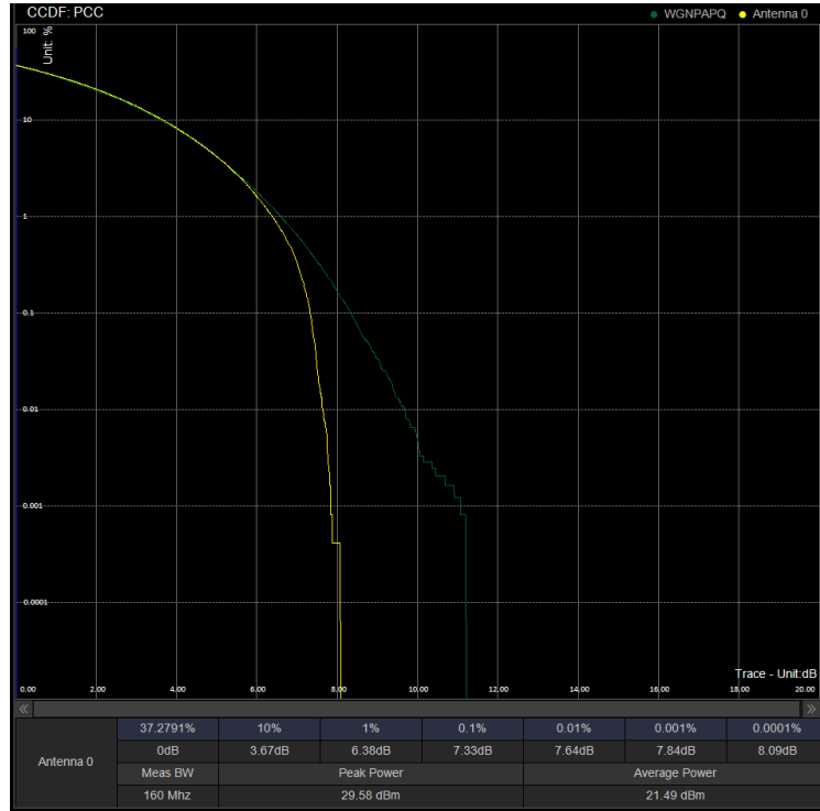
PAPR/PC2\N41\70M CP 531000 100%RB 16QAM
