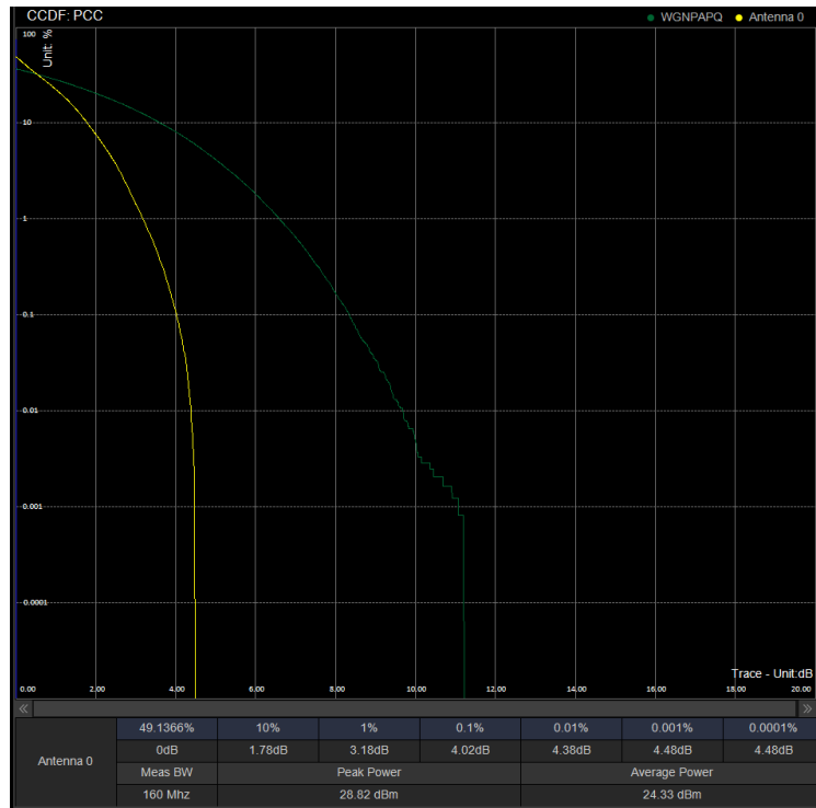
PAPR/PC2\N41\30M DFT 534996 100%RB BPSK
