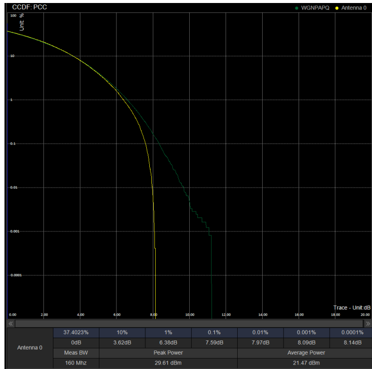
PAPR/PC2\N41\70M CP 506202 100%RB 256QAM
