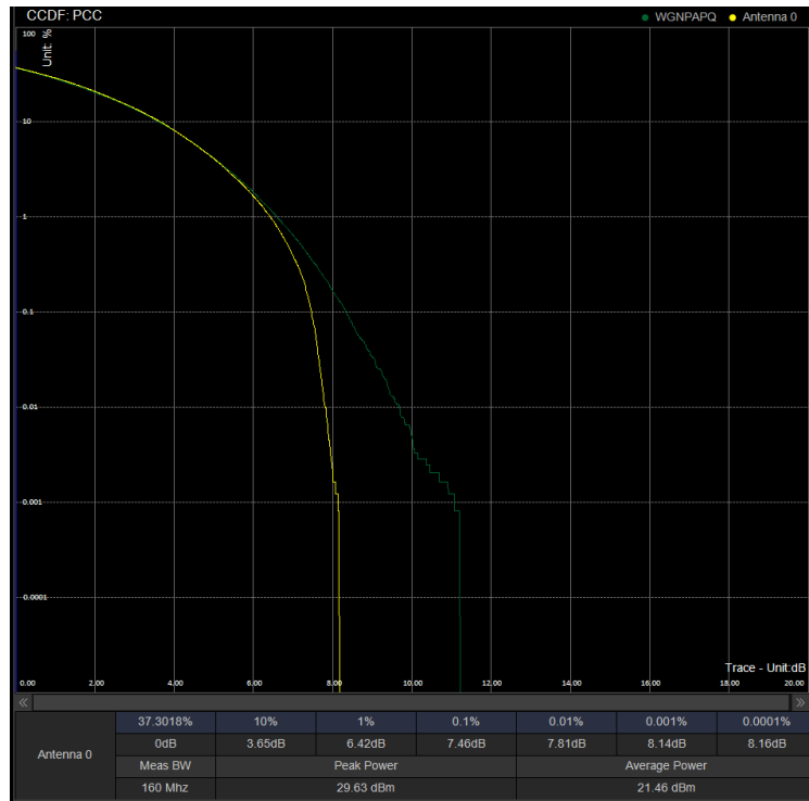
PAPR/PC2\N41\70M CP 531000 100%RB 256QAM
