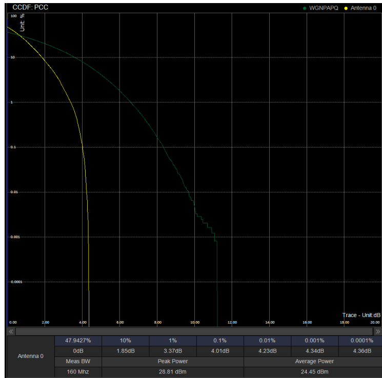
PAPR/PC2\N41\40M DFT 503202 100%RB QPSK
