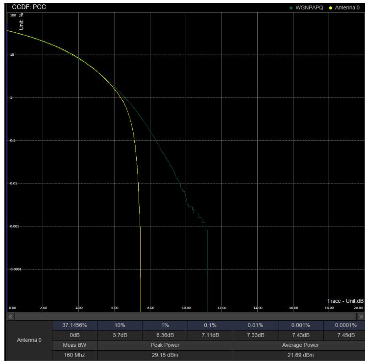
PAPR/PC2\N41\60M CP 531996 100%RB 16QAM
