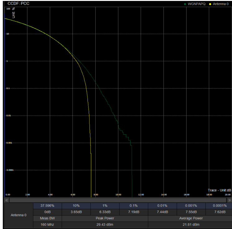
PAPR/PC2\N41\60M CP 505200 100%RB 256QAM
