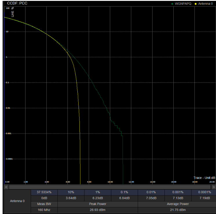
PAPR/PC2\N41\40M CP 518598 100%RB 256QAM
