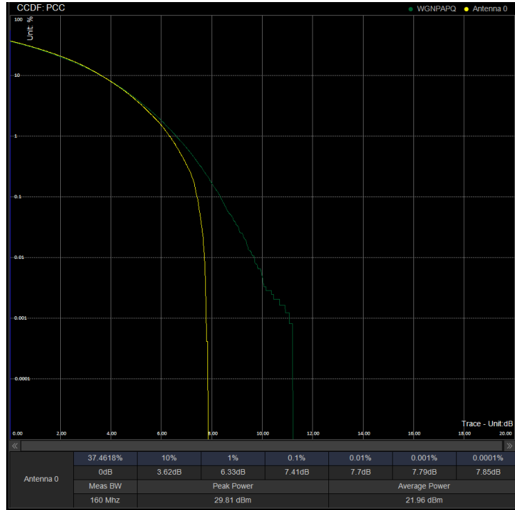
PAPR/PC2\N41\40M CP 503202 100%RB 256QAM
