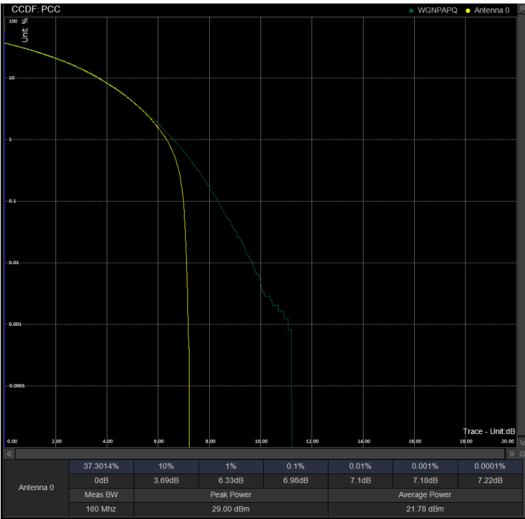
PAPR/PC2\N41\40M CP 534000 100%RB 256QAM
