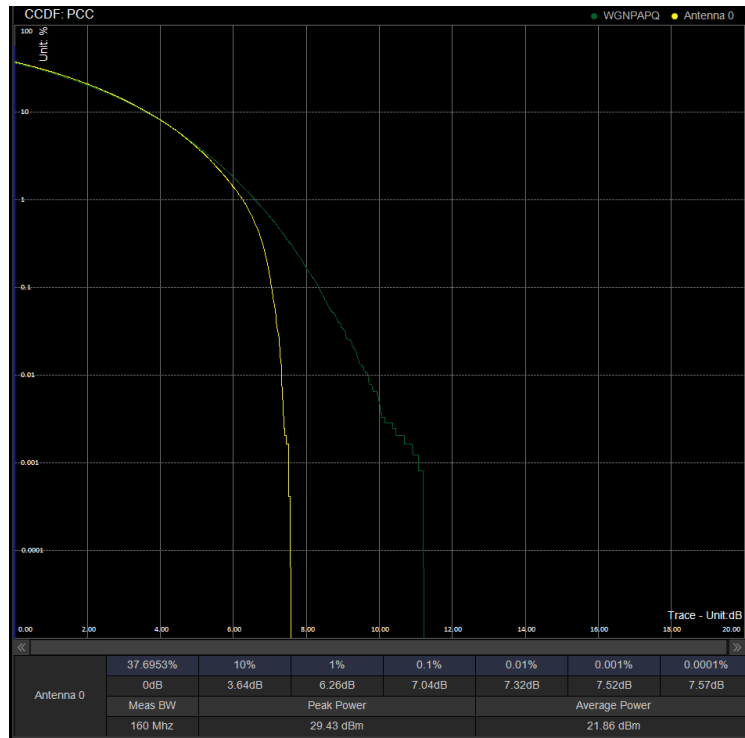
PAPR/PC2\N41\50M CP 504204 100%RB QPSK
