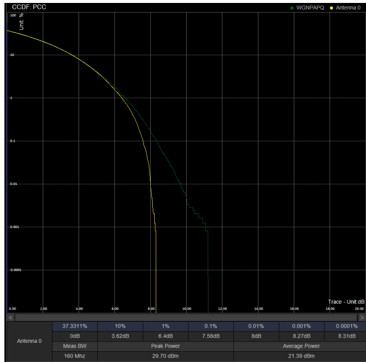
PAPR/PC2\N41\70M CP 518598 100%RB 256QAM
