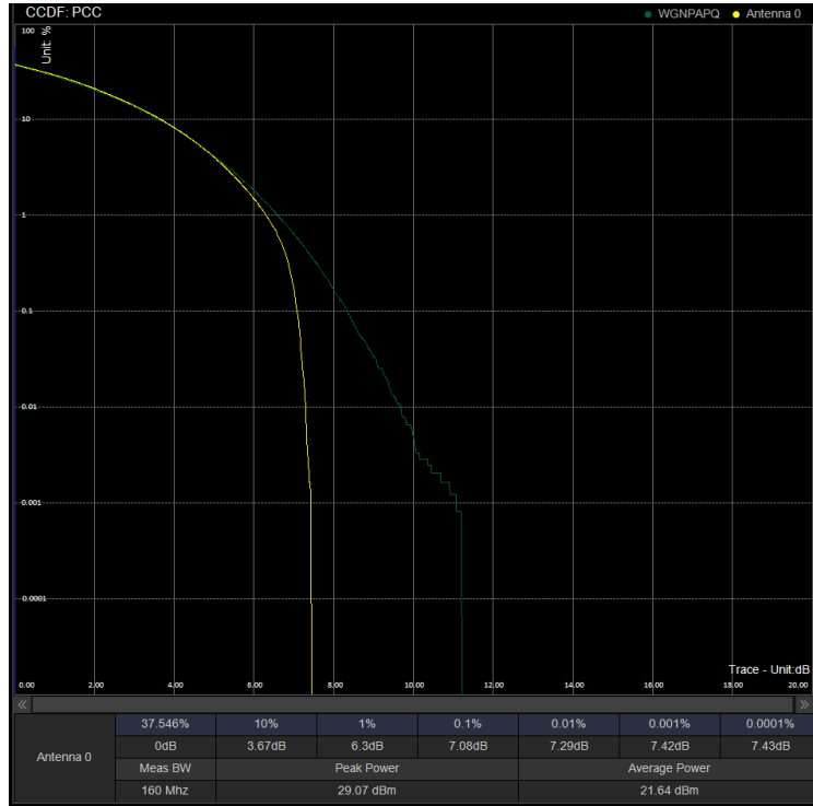
PAPR/PC2\N41\50M CP 518598 100%RB 64QAM
