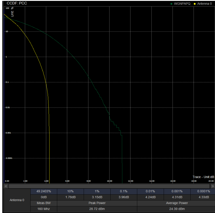
PAPR/PC2\N41\30M DFT 534996 100%RB QPSK
