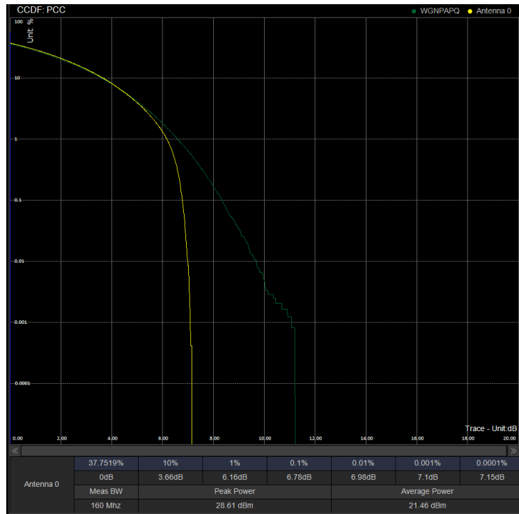
PAPR/PC2\N41\70M CP 506202 100%RB QPSK
