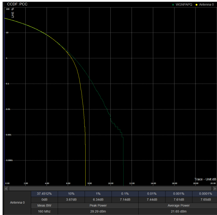
PAPR/PC2\N41\60M CP 518598 100%RB 16QAM
