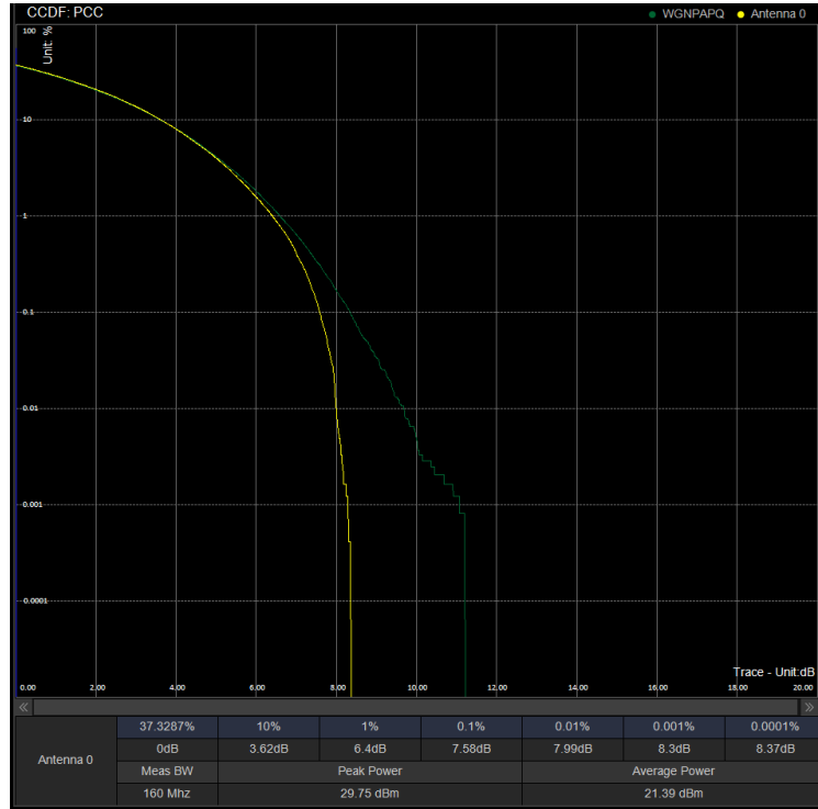
PAPR/PC2\N41\70M CP 518598 100%RB 64QAM
