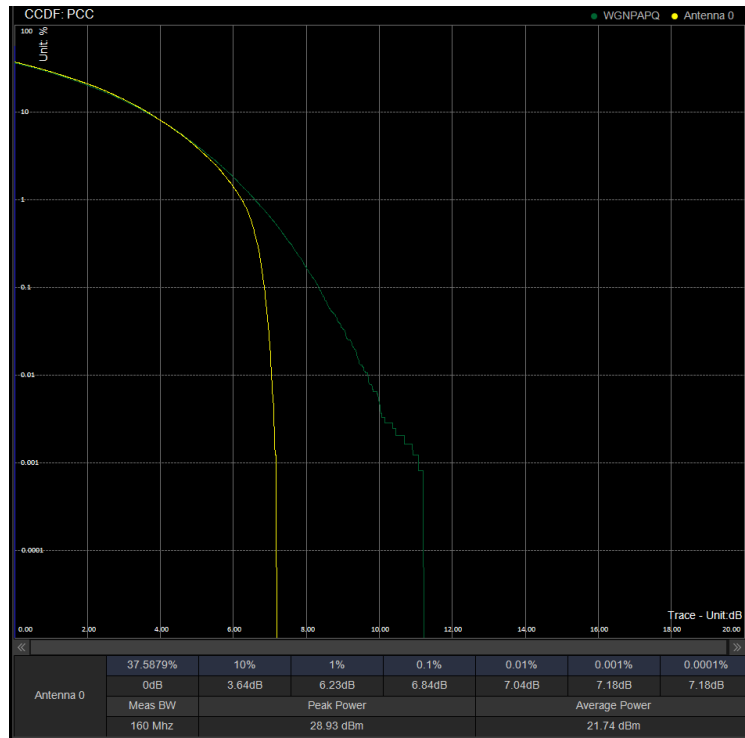
PAPR/PC2\N41\40M CP 518598 100%RB 64QAM
