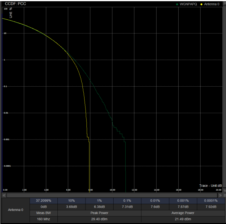
PAPR/PC2\N41\70M CP 531000 100%RB QPSK
