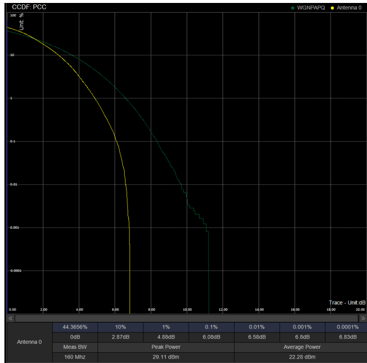
PAPR/PC2\N41\60M DFT 505200 100%RB 64QAM
