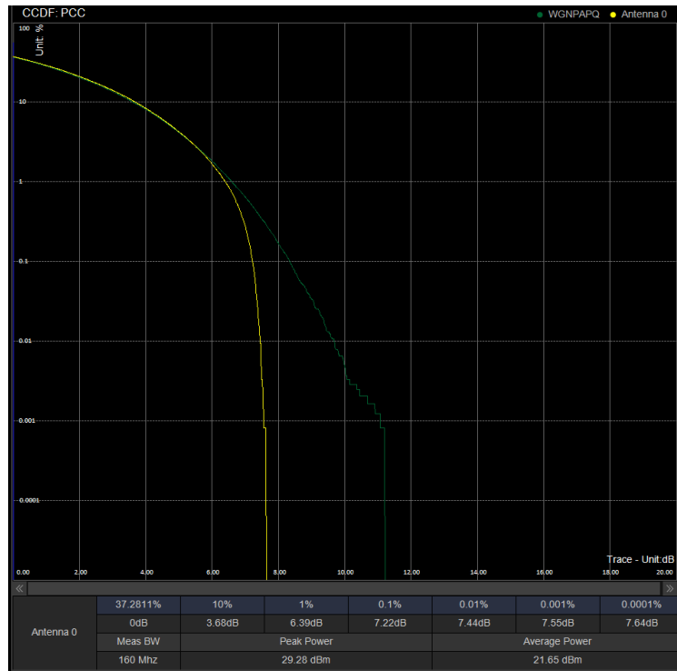
PAPR/PC2\N41\60M CP 531996 100%RB 64QAM
