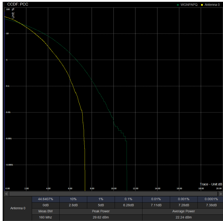
PAPR/PC2\N41\30M DFT 518598 100%RB 64QAM
