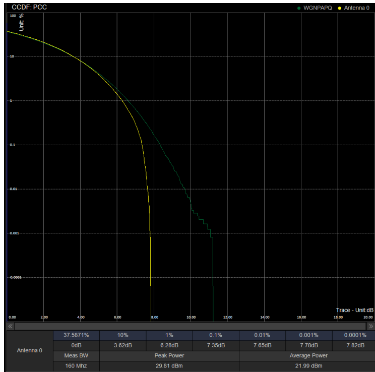
PAPR/PC2\N41\40M CP 503202 100%RB 16QAM
