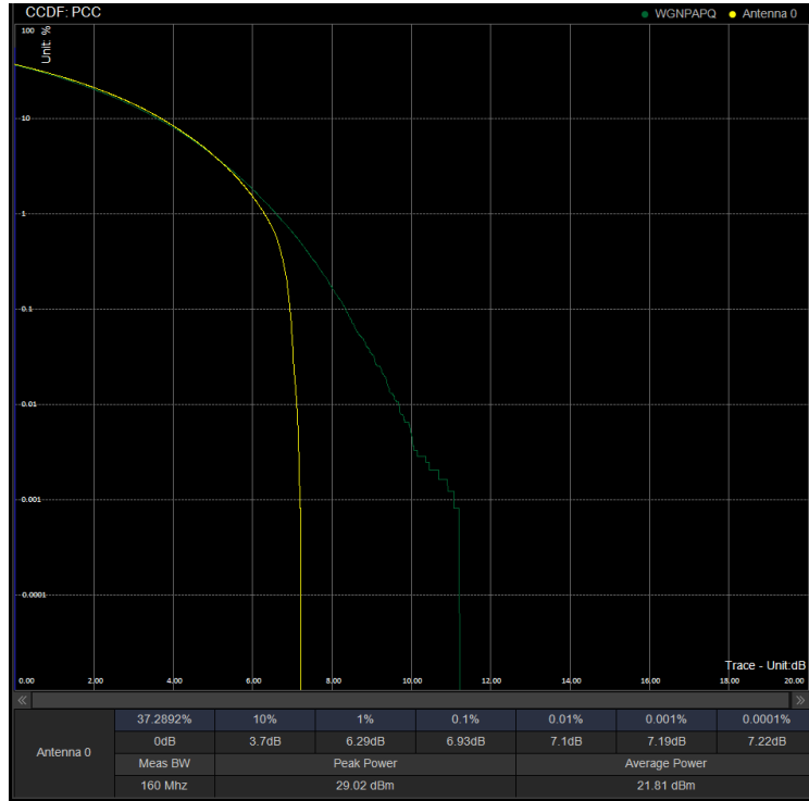
PAPR/PC2\N41\40M CP 534000 100%RB QPSK
