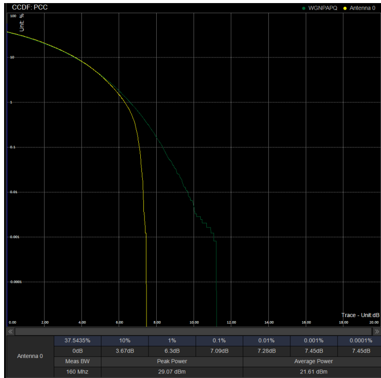
PAPR/PC2\N41\50M CP 518598 100%RB 256QAM
