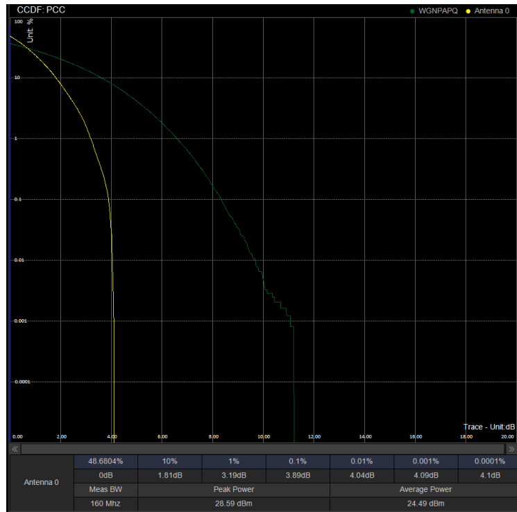
PAPR/PC2\N41\30M DFT 502200 100%RB BPSK
