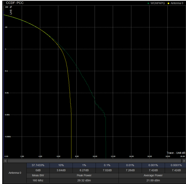
PAPR/PC2\N41\50M CP 504204 100%RB 64QAM
