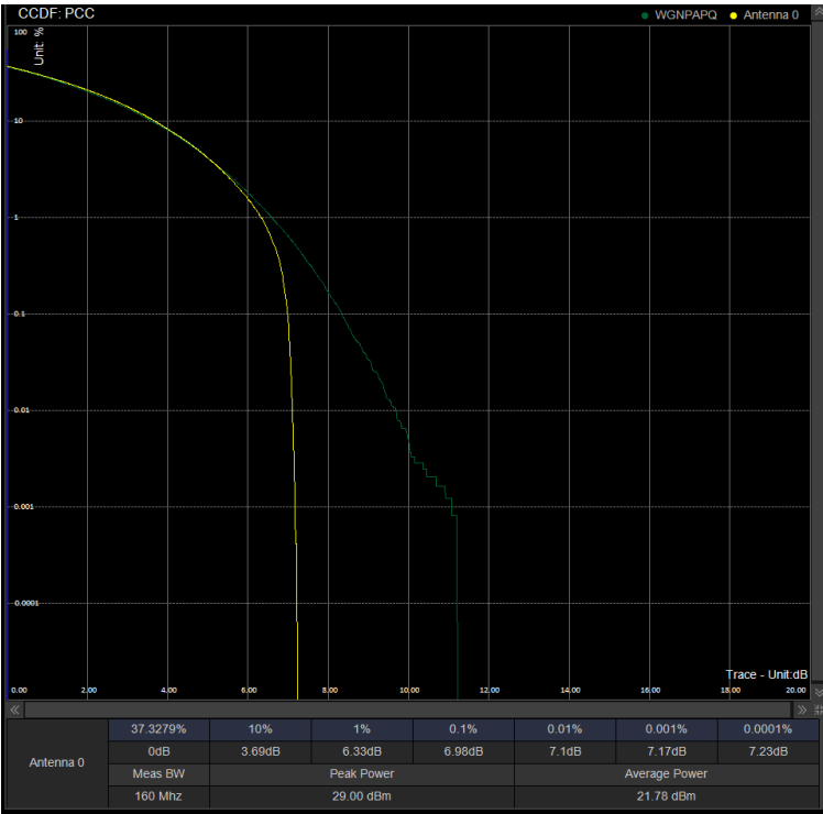
PAPR/PC2\N41\40M CP 534000 100%RB 64QAM
