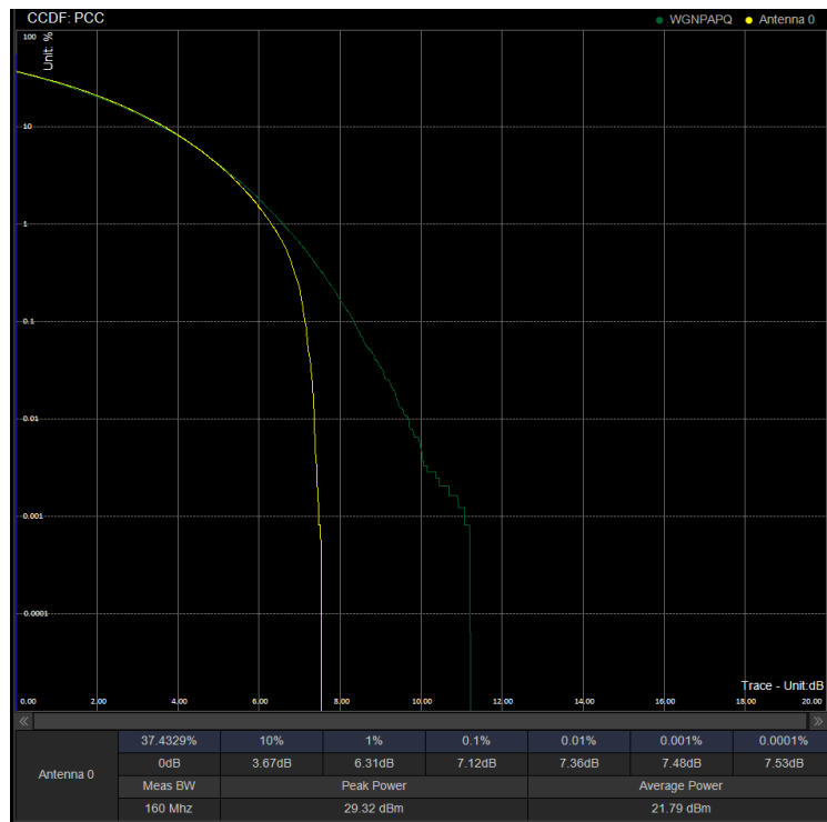
PAPR/PC2\N41\60M CP 505200 100%RB 16QAM
