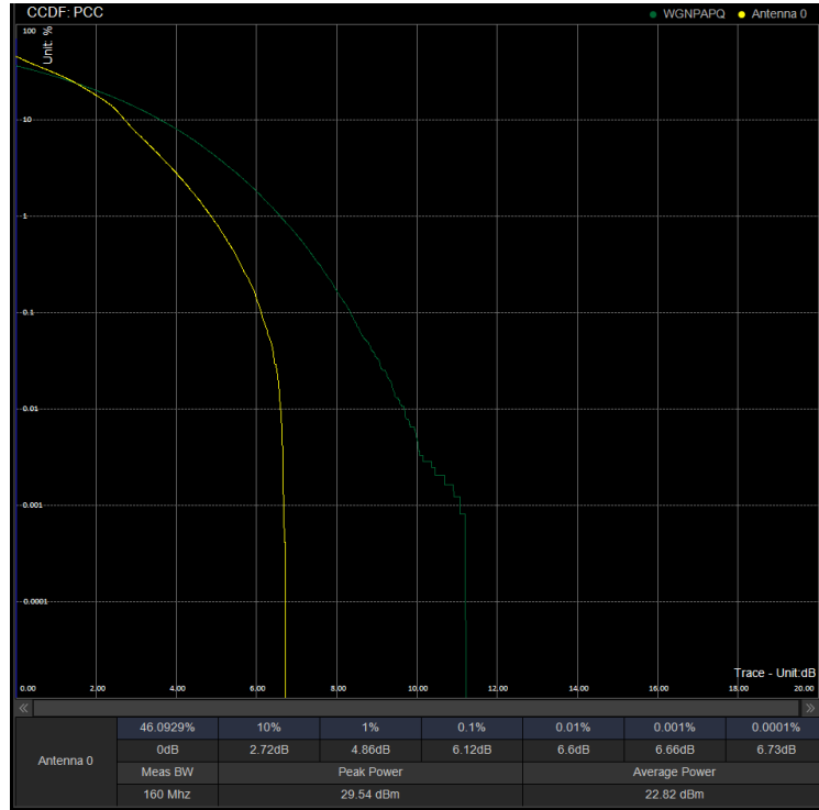
PAPR/PC2\N41\30M DFT 534996 100%RB 16QAM
