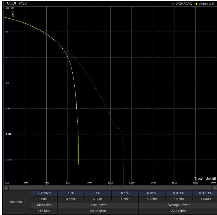
PAPR/PC2\N41\40M CP 503202 100%RB QPSK
