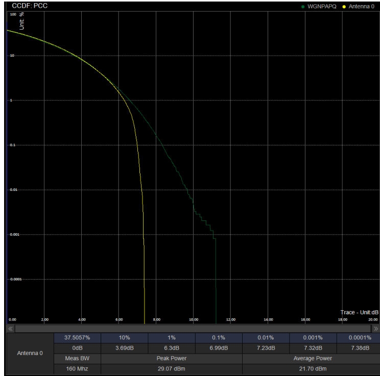
PAPR/PC2\N41\50M CP 532998 100%RB 16QAM
