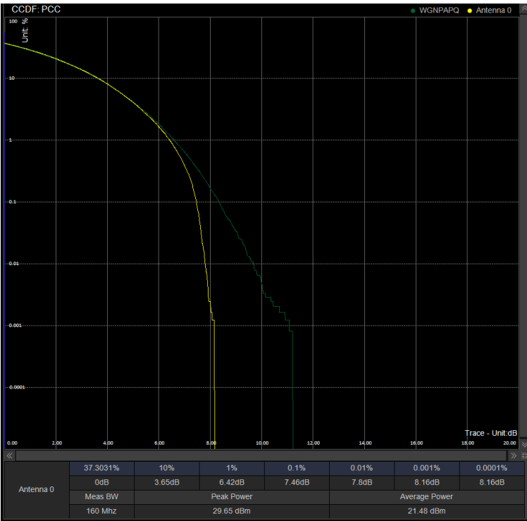
PAPR/PC2\N41\70M CP 531000 100%RB 64QAM
