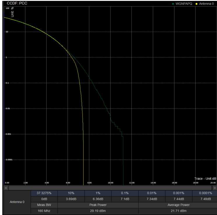
PAPR/PC2\N41\50M CP 532998 100%RB 64QAM
