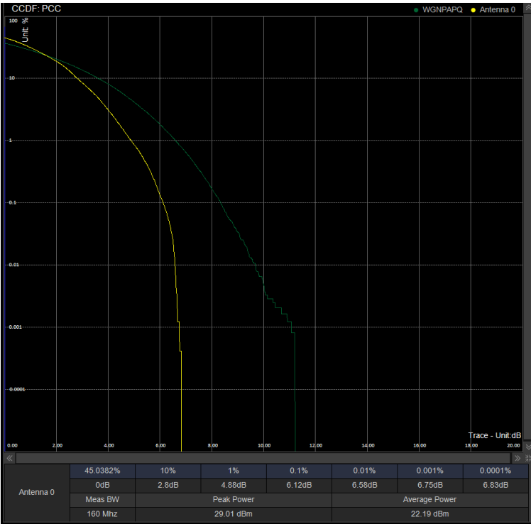
PAPR/PC2\N41\20M DFT 501204 100%RB 64QAM
