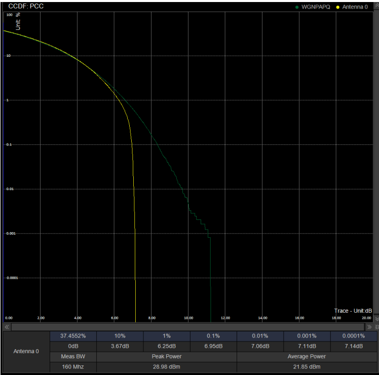
PAPR/PC2\N41\20M CP 535998 100%RB 16QAM
