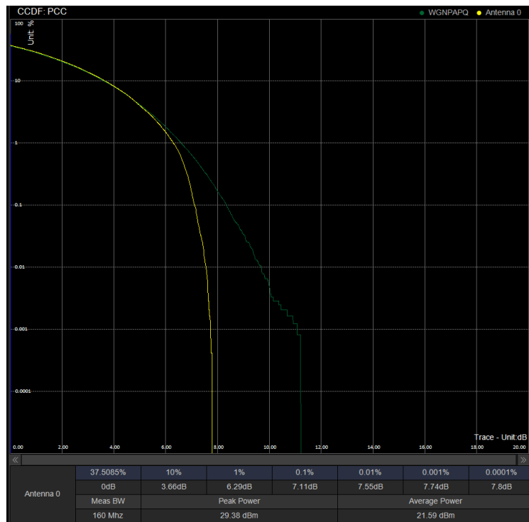
PAPR/PC2\N41\100M CP 509202 100%RB 256QAM
