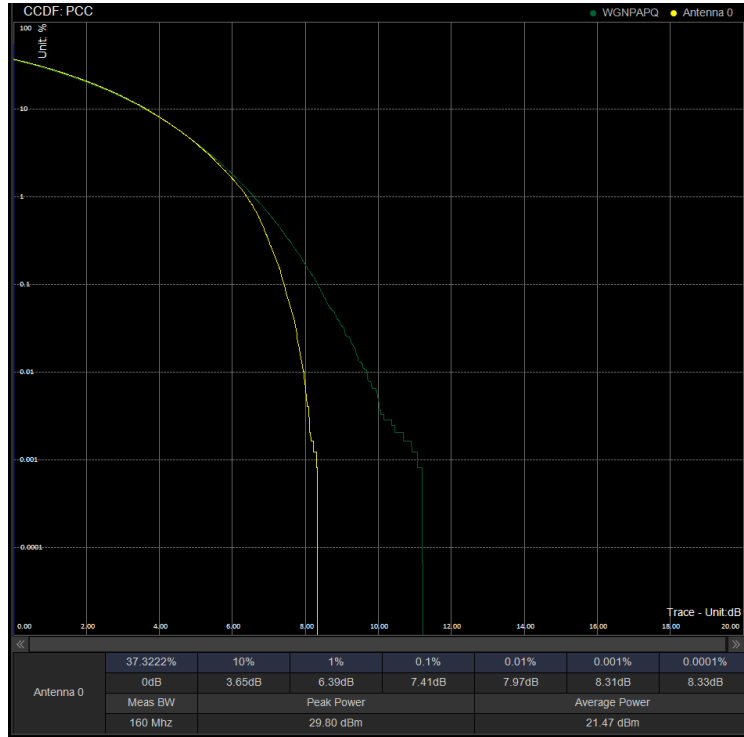
PAPR/PC2\N41\100M CP 528000 100%RB 64QAM
