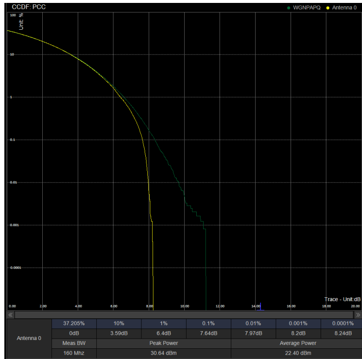
PAPR/PC3\N78(3450-3550)\90M CP 633334 100%RB 256QAM
