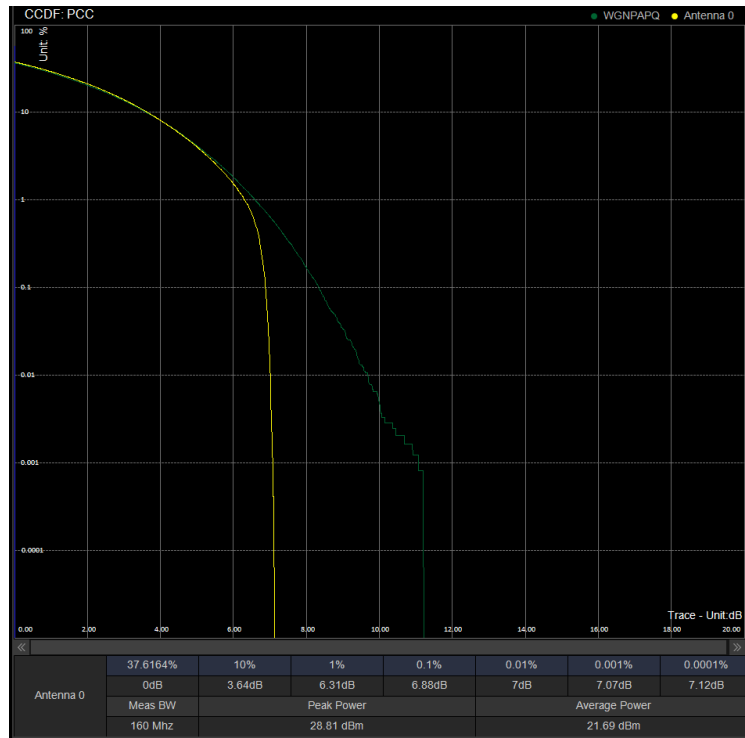
PAPR/PC2\N41\30M CP 518598 100%RB 256QAM
