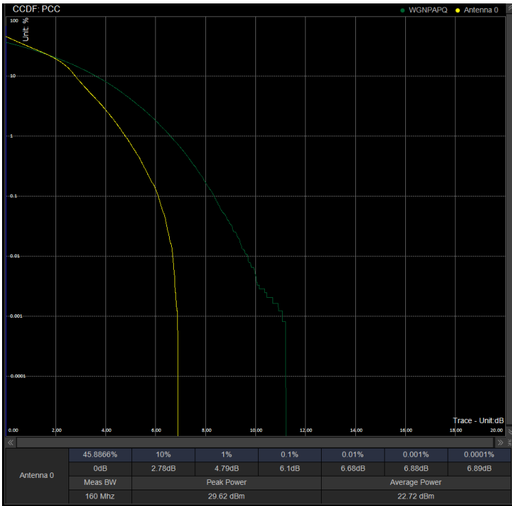
PAPR/PC2\N41\20M DFT 518598 100%RB 16QAM
