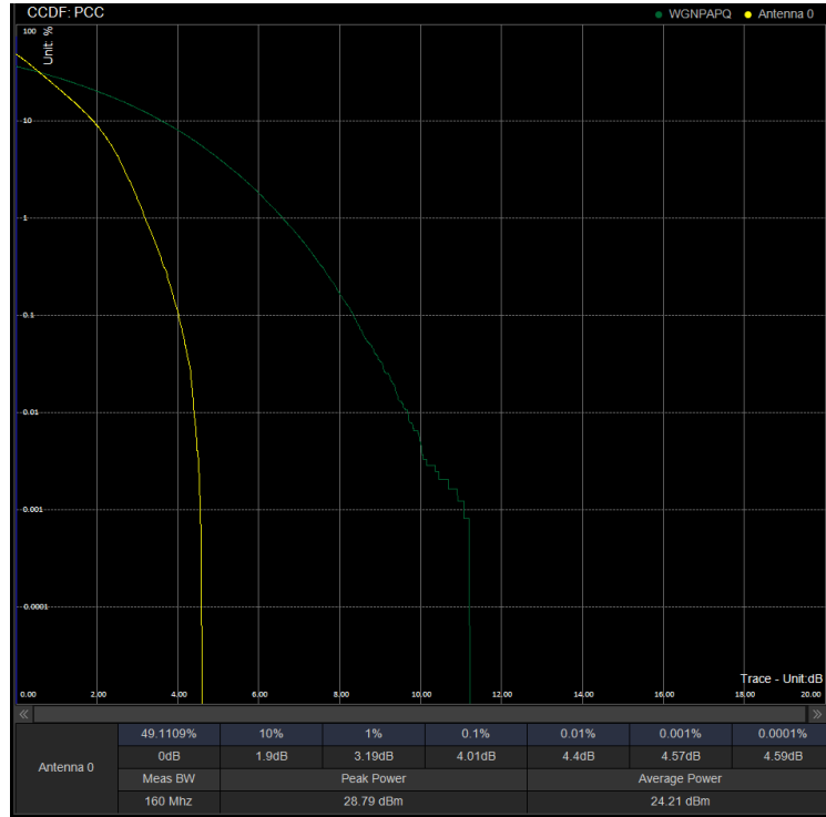
PAPR/PC2\N41\20M DFT 518598 100%RB QPSK
