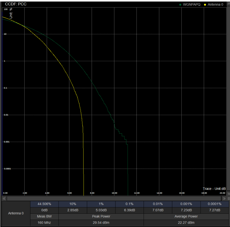
PAPR/PC2\N41\20M DFT 518598 100%RB 64QAM
