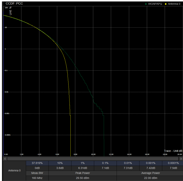
PAPR/PC2\N41\30M CP 502200 100%RB 256QAM
