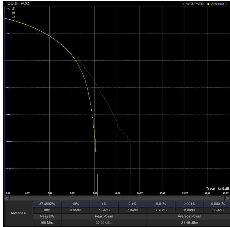
PAPR/PC2\N41\100M CP 528000 100%RB 16QAM
