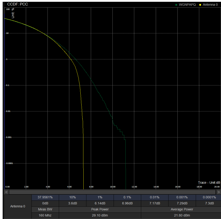
PAPR/PC2\N41\20M CP 501204 100%RB 16QAM
