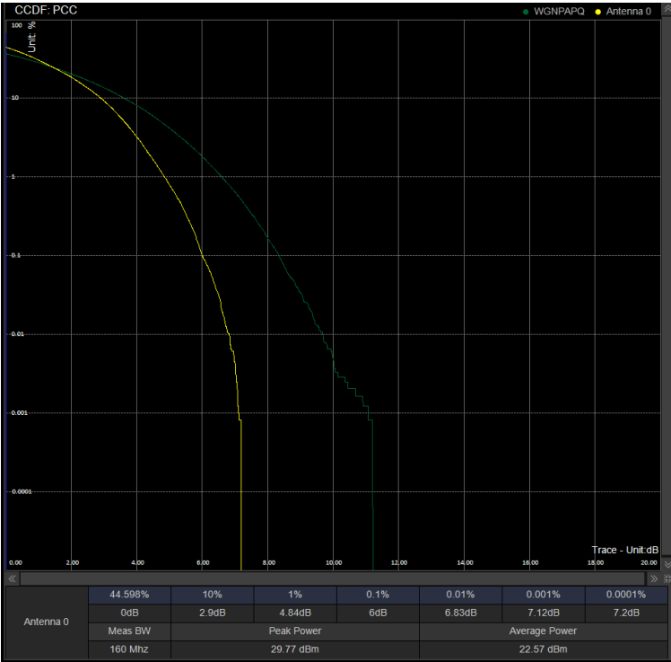
PAPR/PC2\N41\100M DFT 509202 100%RB 16QAM
