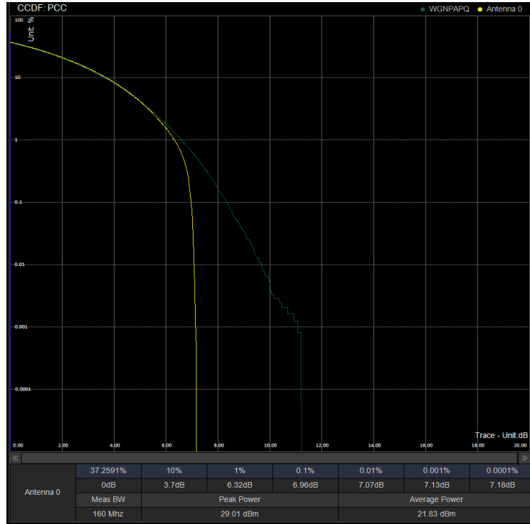
PAPR/PC2\N41\20M CP 535998 100%RB QPSK
