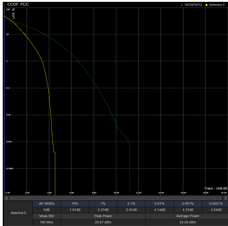
PAPR/PC2\N41\100M DFT 509202 100%RB BPSK
