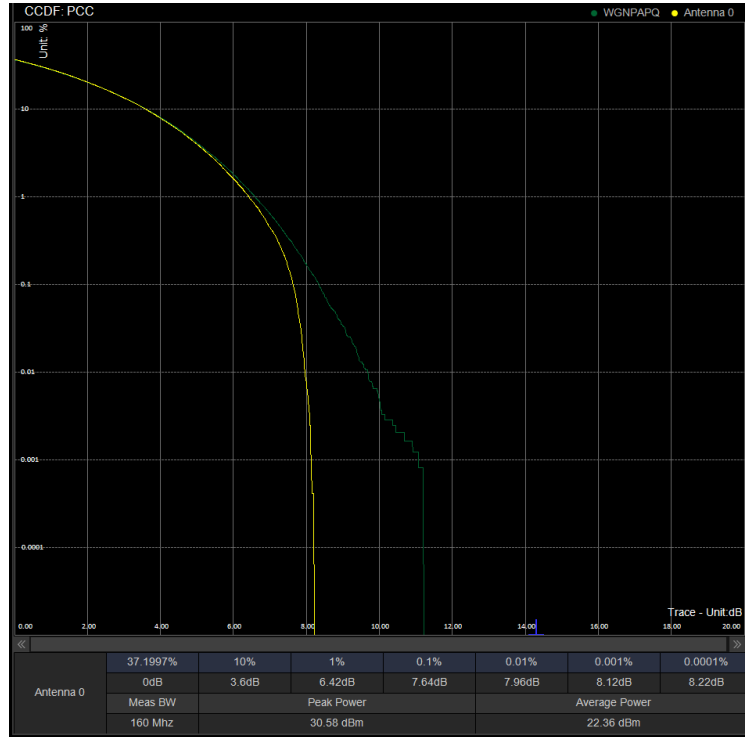
PAPR/PC3\N78(3450-3550)\90M CP 633666 100%RB 64QAM
