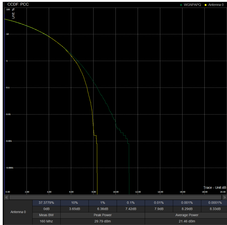
PAPR/PC2\N41\100M CP 528000 100%RB 256QAM
