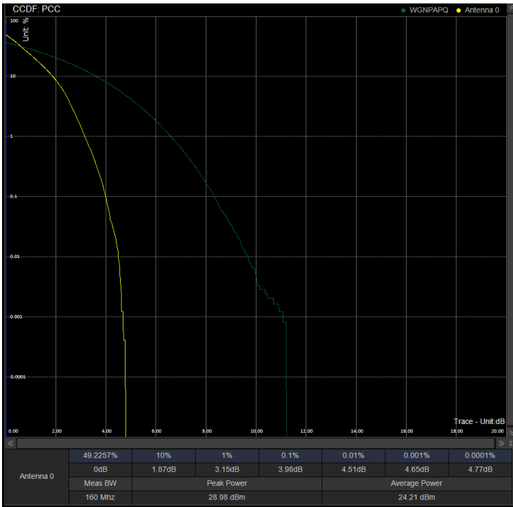
PAPR/PC2\N41\20M DFT 501204 100%RB BPSK
