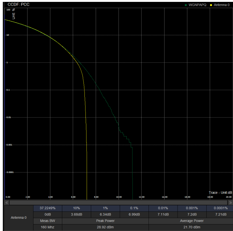
PAPR/PC2\N41\20M CP 518598 100%RB 64QAM
