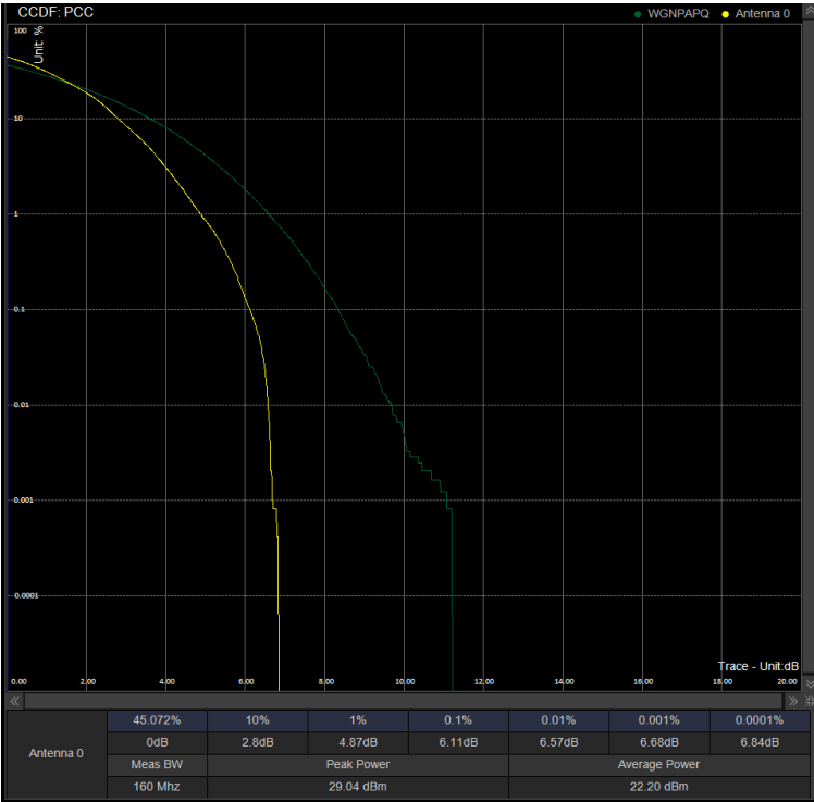
PAPR/PC2\N41\20M DFT 501204 100%RB 256QAM
