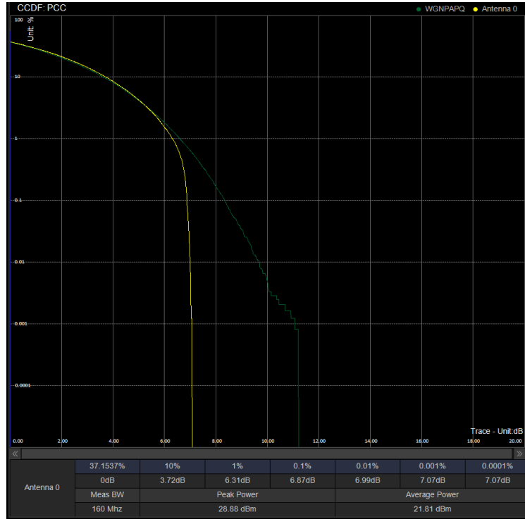
PAPR/PC2\N41\30M CP 534996 100%RB 16QAM
