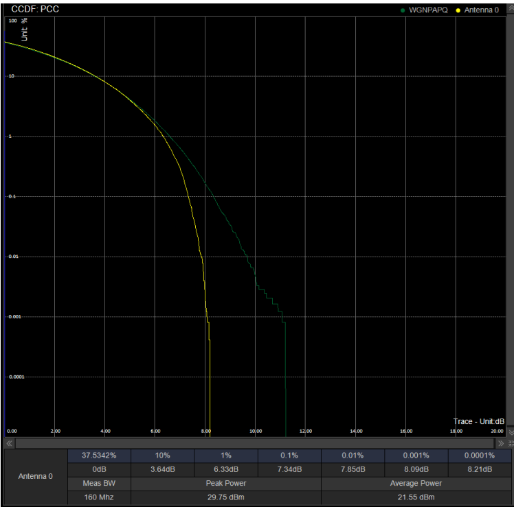
PAPR/PC2\N41\100M CP 518598 100%RB 16QAM
