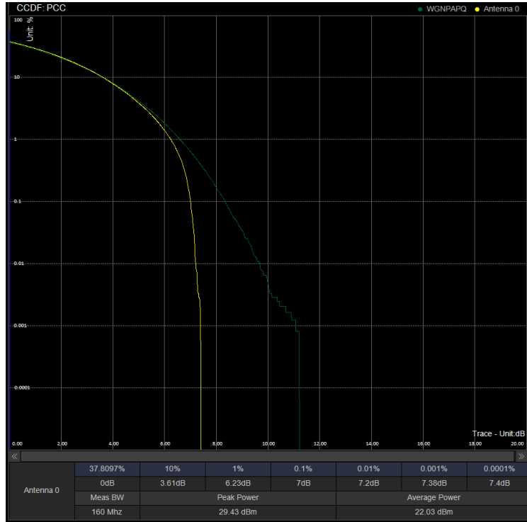
PAPR/PC2\N41\30M CP 502200 100%RB 16QAM
