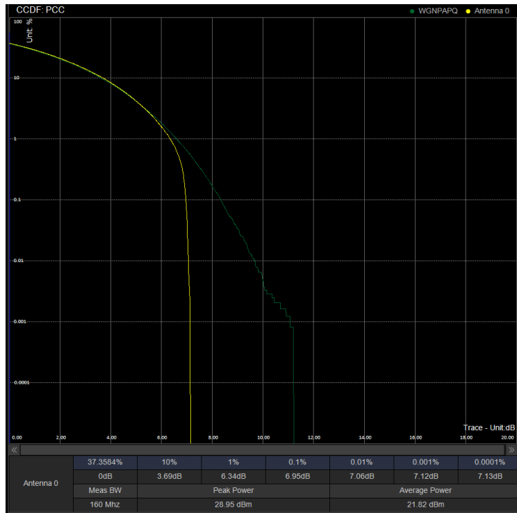
PAPR/PC2\N41\30M CP 534996 100%RB QPSK
