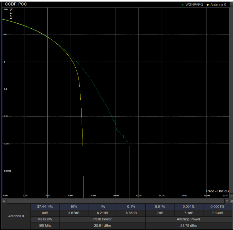
PAPR/PC2\N41\20M CP 518598 100%RB QPSK
