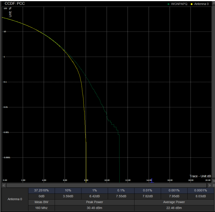
PAPR/PC3\N78(3450-3550)\90M CP 633334 100%RB QPSK
