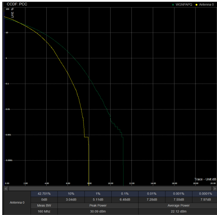
PAPR/PC2\N41\100M DFT 518598 100%RB 64QAM
