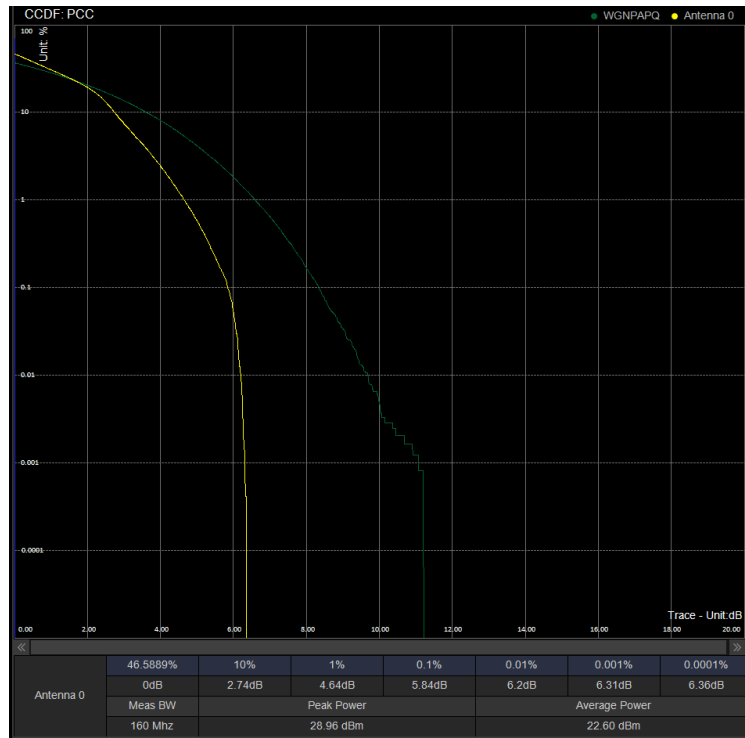
PAPR/PC2\N41\20M DFT 501204 100%RB 16QAM
