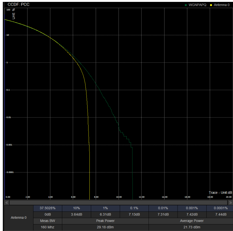
PAPR/PC2\N41\20M CP 501204 100%RB 64QAM
