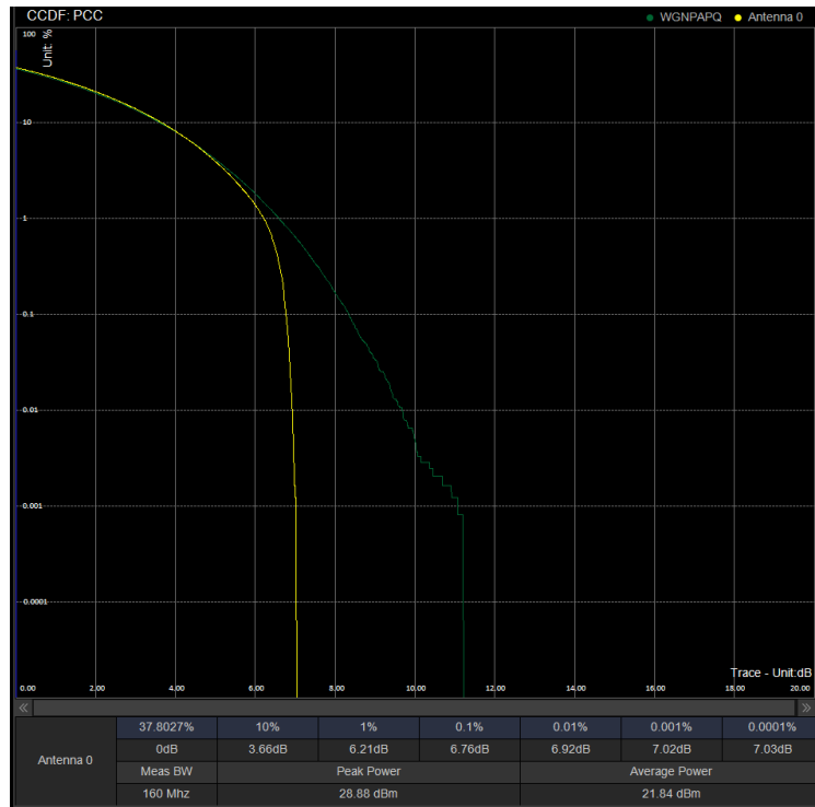
PAPR/PC2\N41\30M CP 518598 100%RB QPSK
