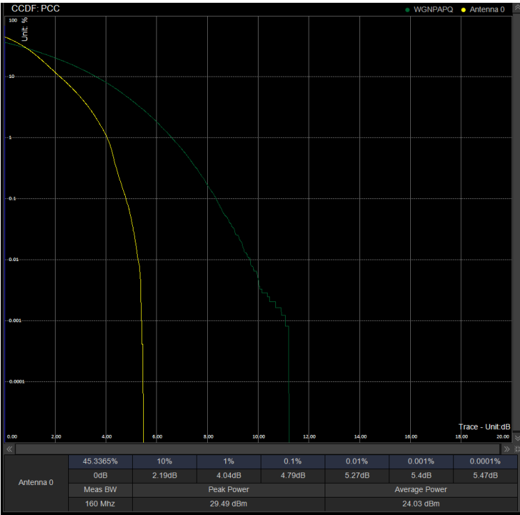
PAPR/PC2\N41\100M DFT 518598 100%RB QPSK
