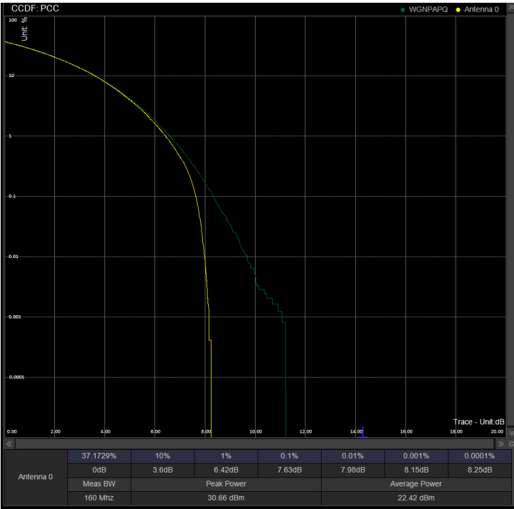
PAPR/PC3\N78(3450-3550)\90M CP 633000 100%RB 256QAM
