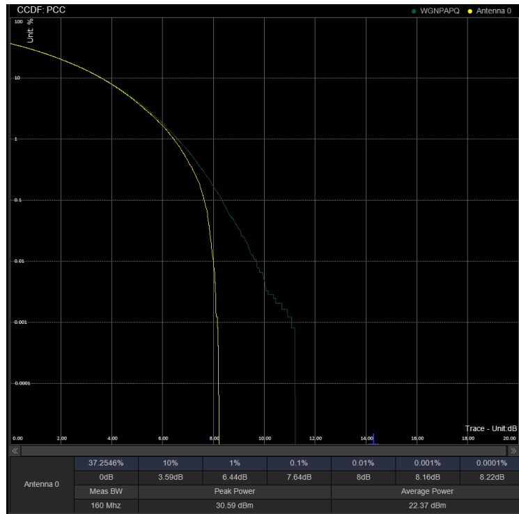
PAPR/PC3\N78(3450-3550)\90M CP 633666 100%RB 256QAM
