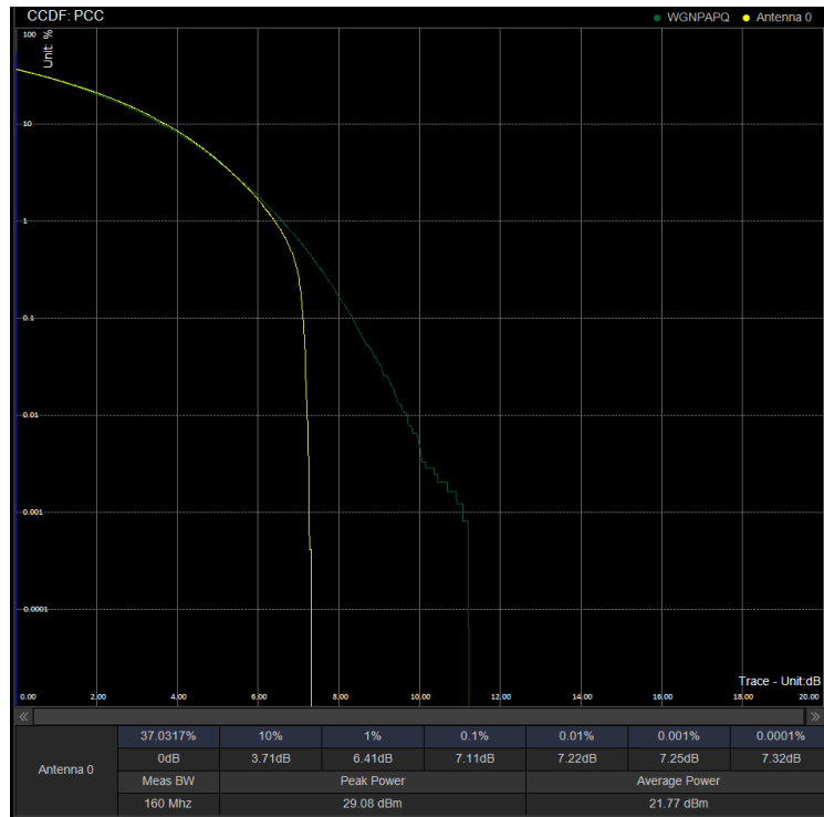
PAPR/PC2\N41\20M CP 535998 100%RB 64QAM
