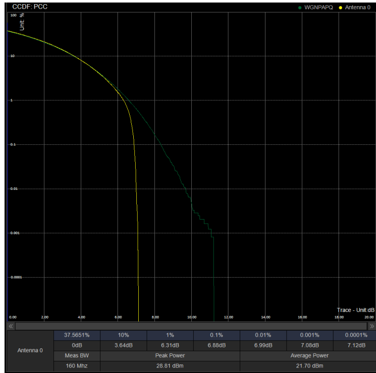
PAPR/PC2\N41\30M CP 518598 100%RB 64QAM
