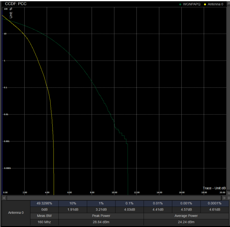
PAPR/PC2\N41\20M DFT 535998 100%RB QPSK
