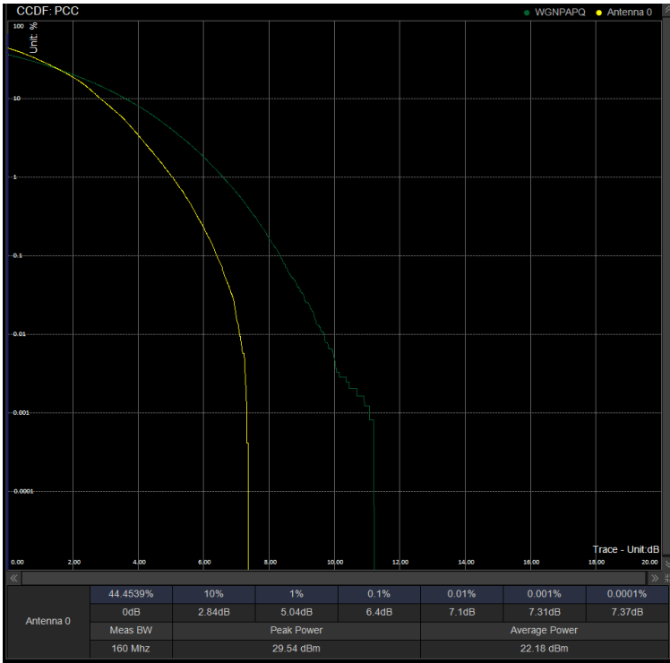
PAPR/PC2\N41\20M DFT 518598 100%RB 256QAM
