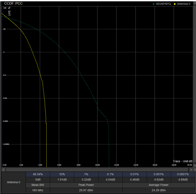
PAPR/PC2\N41\20M DFT 535998 100%RB BPSK
