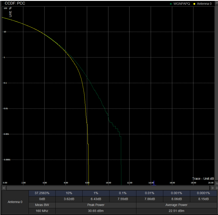
PAPR/PC3\N78(3450-3550)\90M CP 633334 100%RB 64QAM
