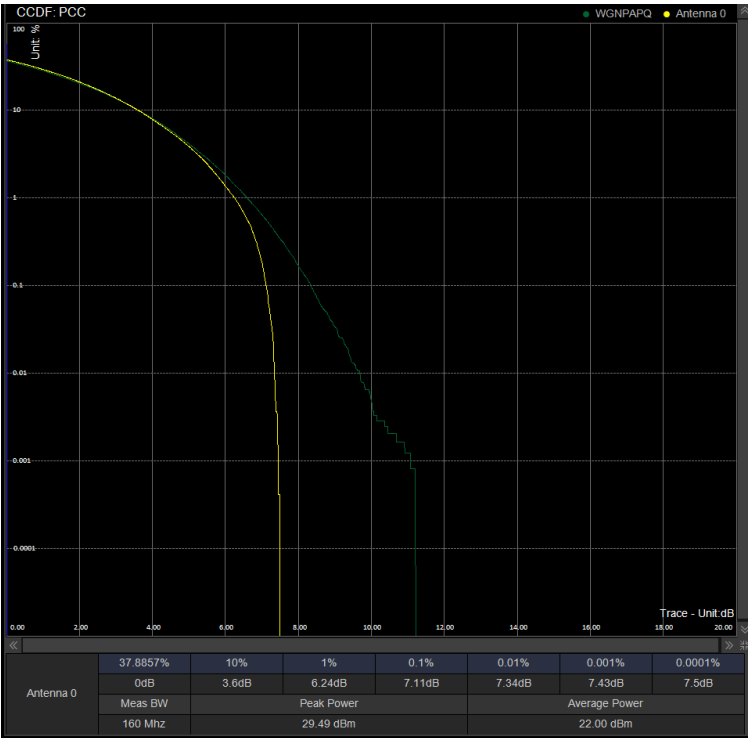
PAPR/PC2\N41\30M CP 502200 100%RB QPSK
