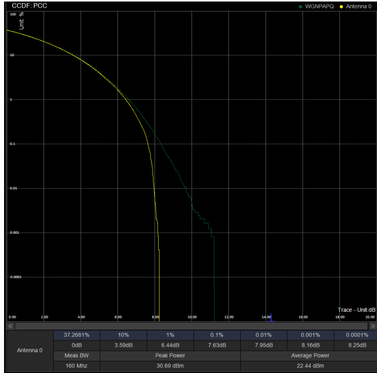
PAPR/PC3\N78(3450-3550)\90M CP 633000 100%RB 64QAM
