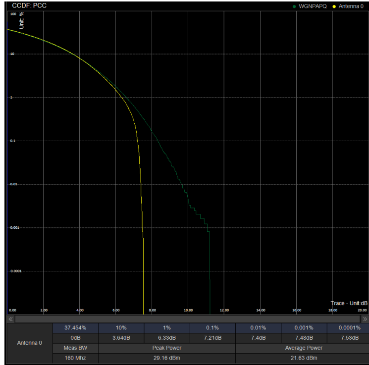
PAPR/PC2\N41\20M CP 501204 100%RB 256QAM
