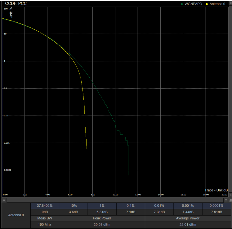
PAPR/PC2\N41\30M CP 502200 100%RB 64QAM
