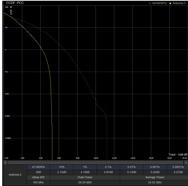
PAPR/PC2\N41\100M DFT 528000 100%RB QPSK
