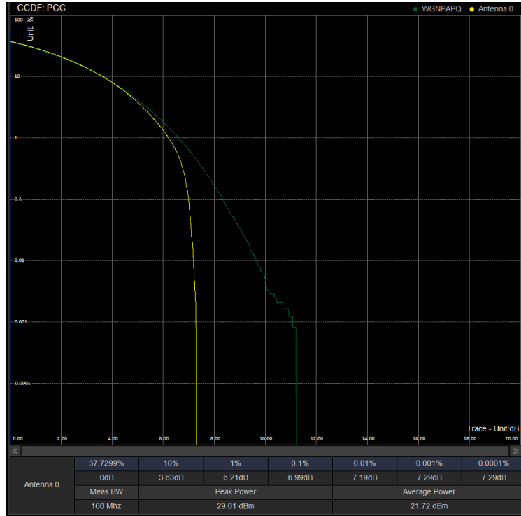
PAPR/PC2\N41\20M CP 501204 100%RB QPSK
