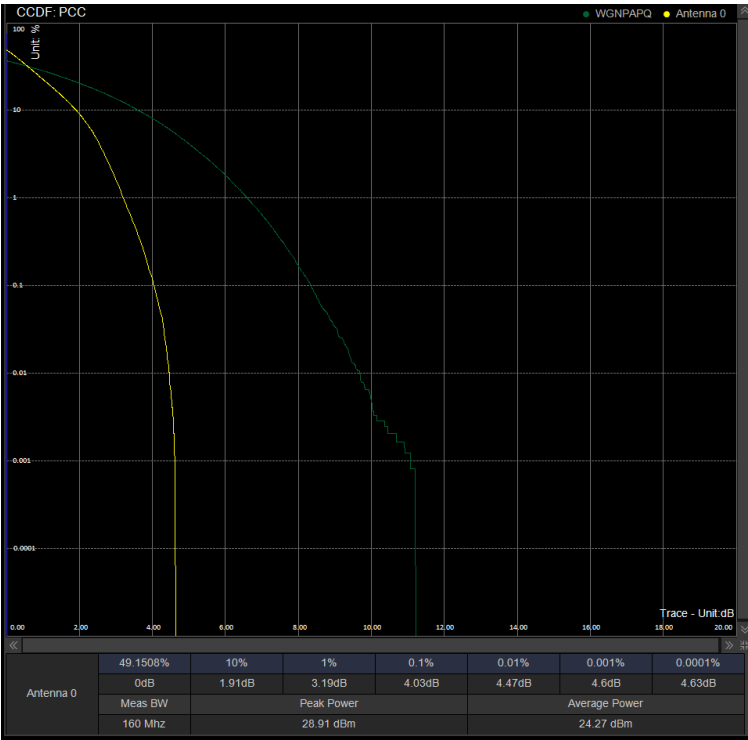
PAPR/PC2\N41\20M DFT 518598 100%RB BPSK
