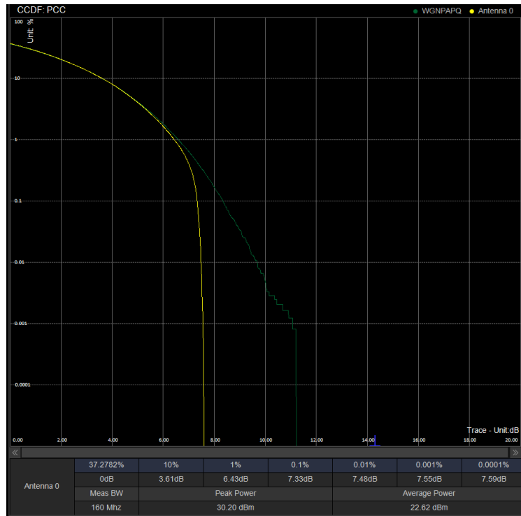
PAPR/PC3\N78(3450-3550)\50M CP 633334 100%RB 256QAM
