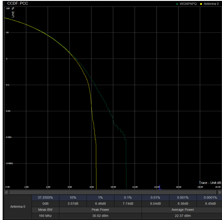
PAPR/PC3\N78(3450-3550)\70M CP 634332 100%RB 64QAM
