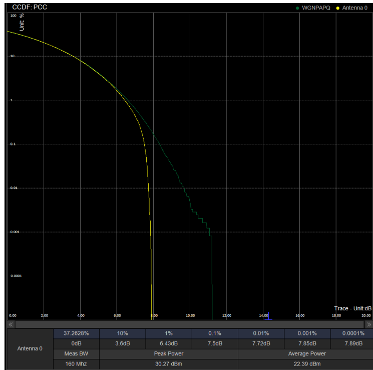
PAPR/PC3\N78(3450-3550)\70M CP 634332 100%RB QPSK
