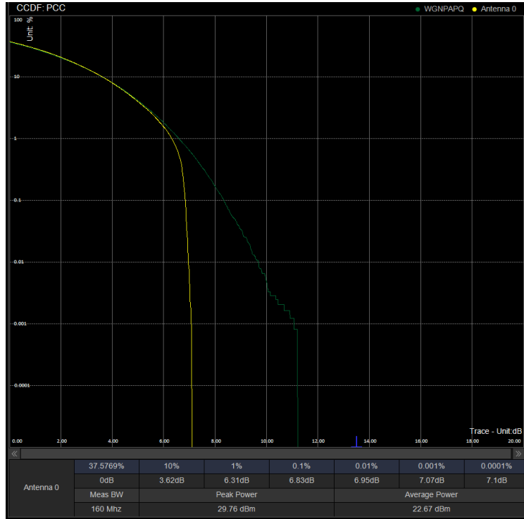
PAPR/PC3\N78(3450-3550)\10M CP 633334 100%RB QPSK
