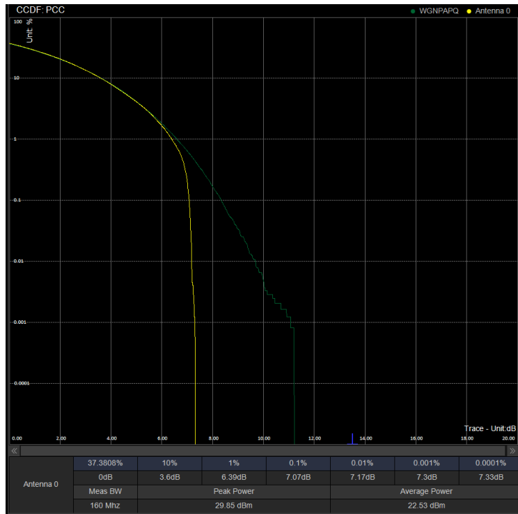
PAPR/PC3\N78(3450-3550)\10M CP 633334 100%RB 16QAM
