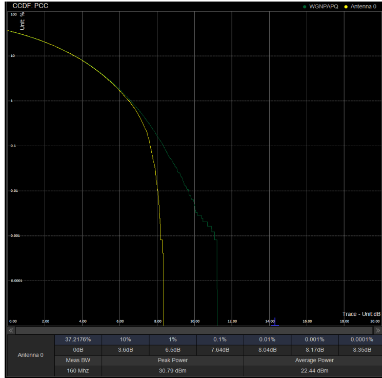
PAPR/PC3\N78(3450-3550)\100M CP 633334 100%RB 64QAM
