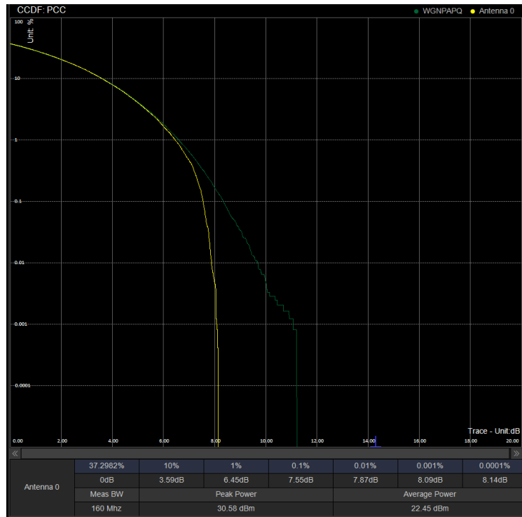
PAPR/PC3\N78(3450-3550)\100M CP 633334 100%RB QPSK
