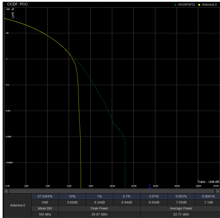
PAPR/PC3\N78(3450-3550)\10M CP 630334 100%RB 16QAM
