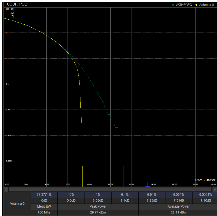
PAPR/PC3\N78(3450-3550)\10M CP 636332 100%RB 16QAM
