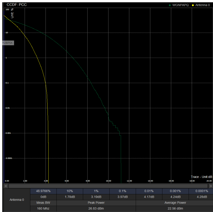
PAPR/PC3\N41\30M DFT 534996 100%RB BPSK
