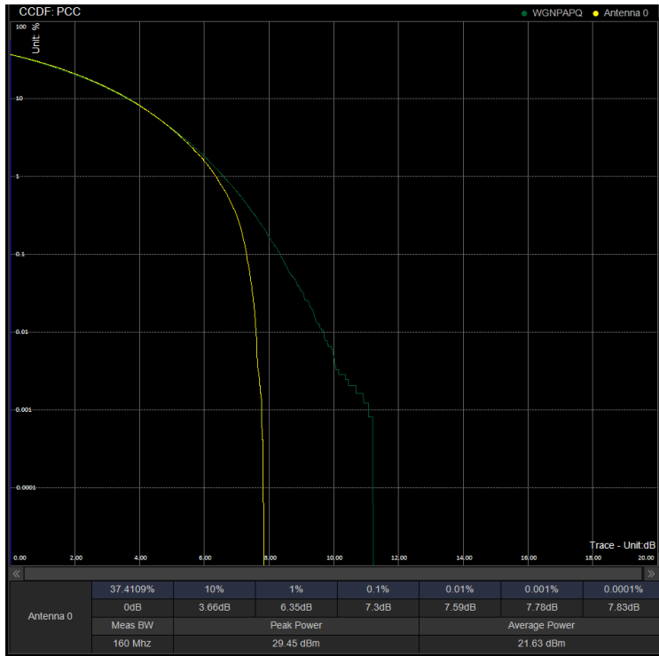
PAPR/PC3\N41\60M CP 505200 100%RB QPSK
