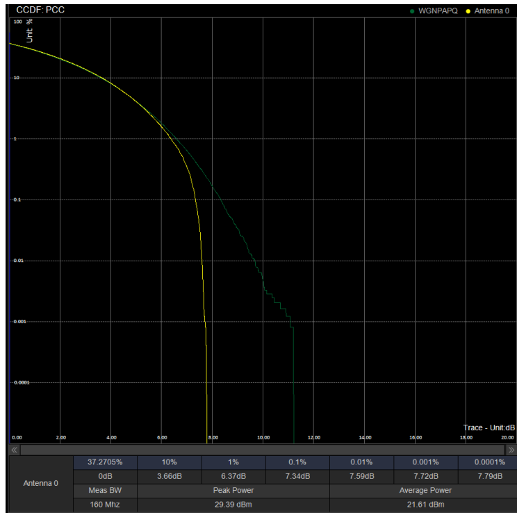
PAPR/PC3\N41\60M CP 505200 100%RB 16QAM
