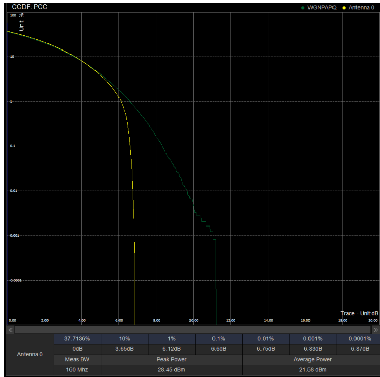
PAPR/PC3\N41\30M CP 518598 100%RB 16QAM
