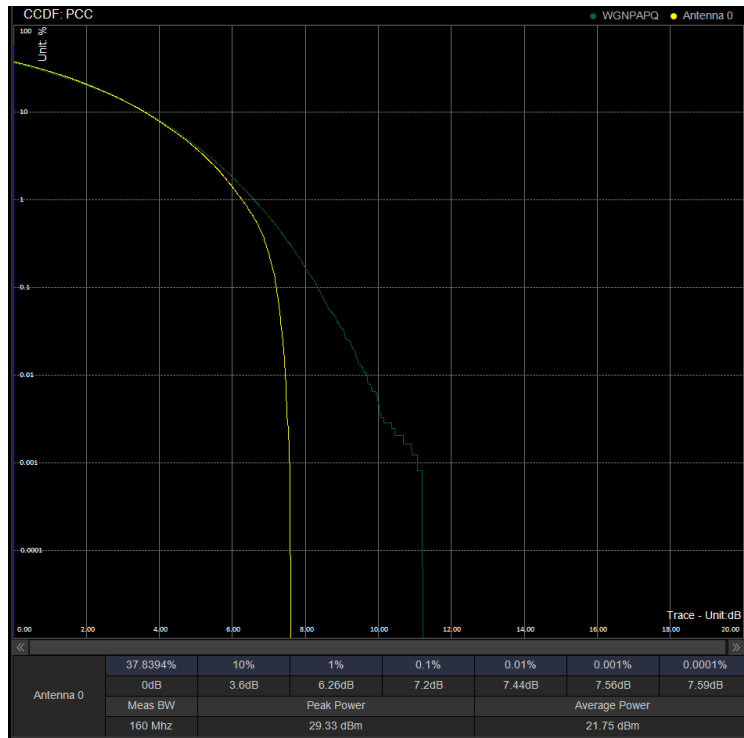
PAPR/PC3\N41\30M CP 502200 100%RB QPSK
