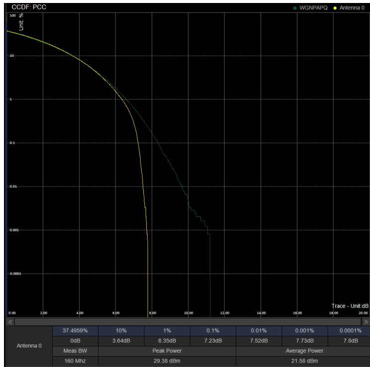
PAPR/PC3\N41\50M CP 504204 100%RB 256QAM
