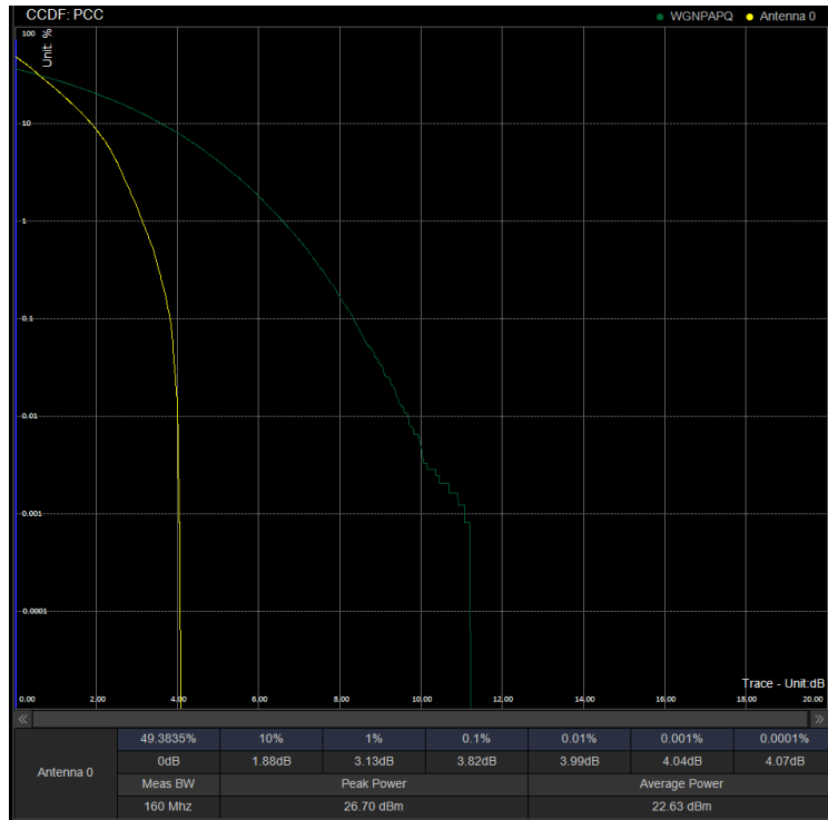
PAPR/PC3\N41\20M DFT 501204 100%RB BPSK
