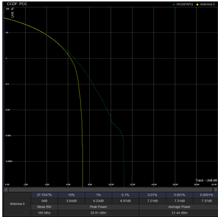
PAPR/PC3\N41\50M CP 518598 100%RB 16QAM
