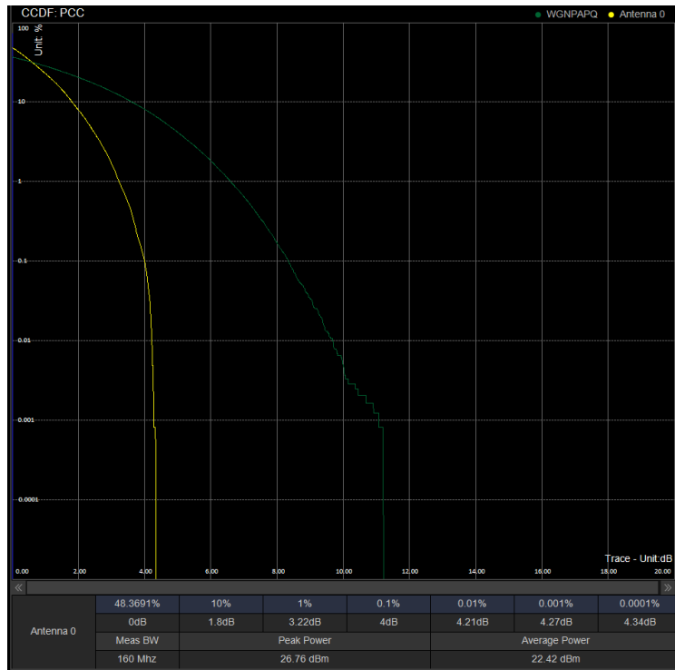
PAPR/PC3\N41\30M DFT 518598 100%RB QPSK
