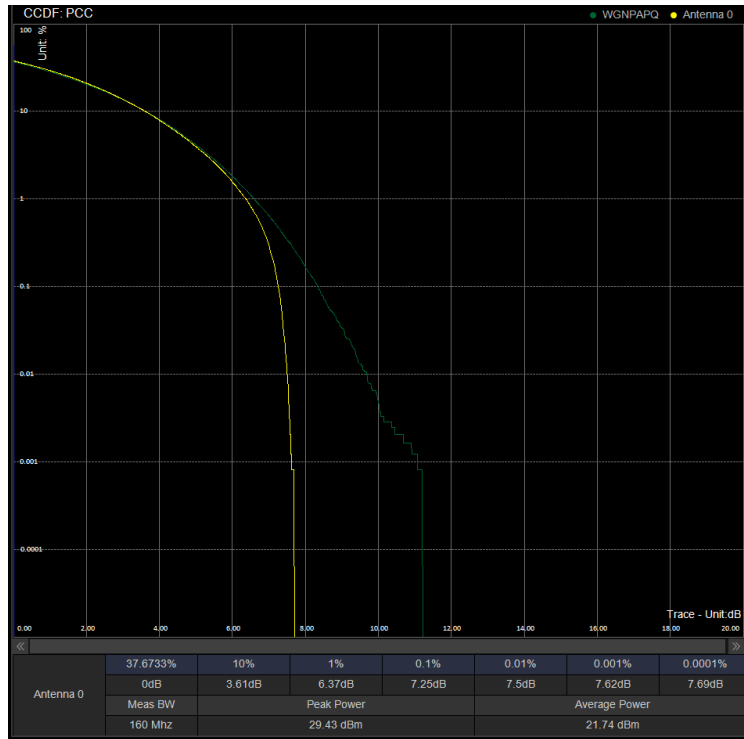
PAPR/PC3\N41\30M CP 502200 100%RB 64QAM
