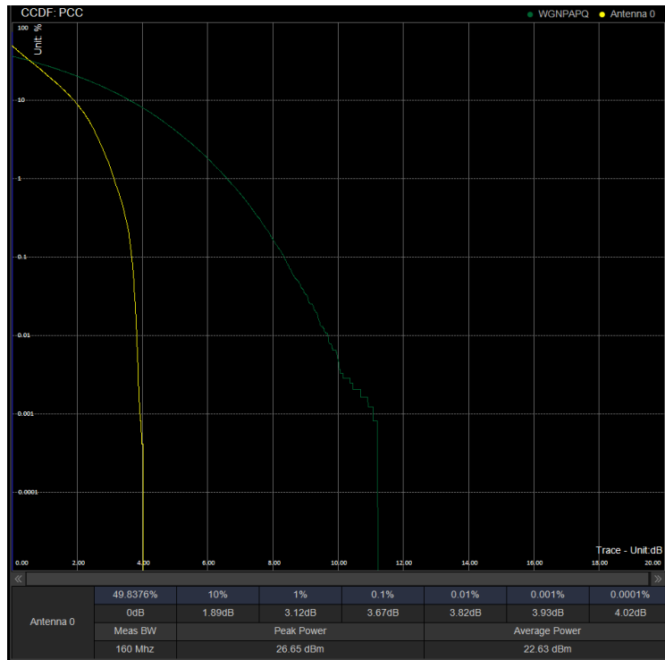
PAPR/PC3\N41\20M DFT 535998 100%RB QPSK
