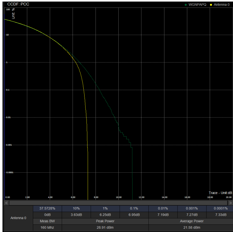
PAPR/PC3\N41\40M CP 518598 100%RB 256QAM
