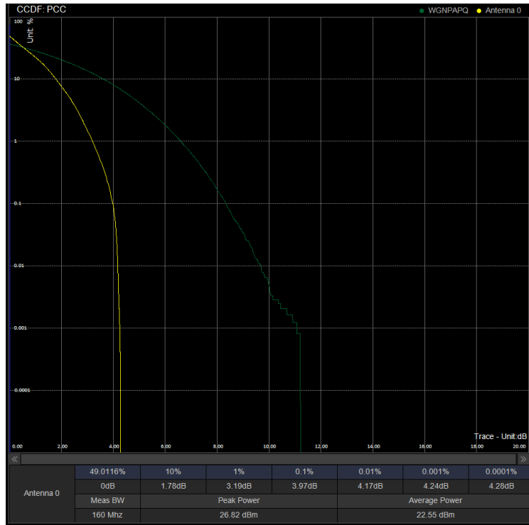
PAPR/PC3\N41\30M DFT 534996 100%RB QPSK
