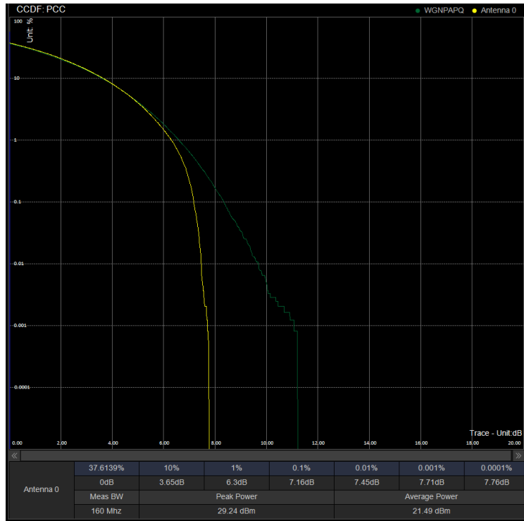
PAPR/PC3\N41\60M CP 518598 100%RB QPSK
