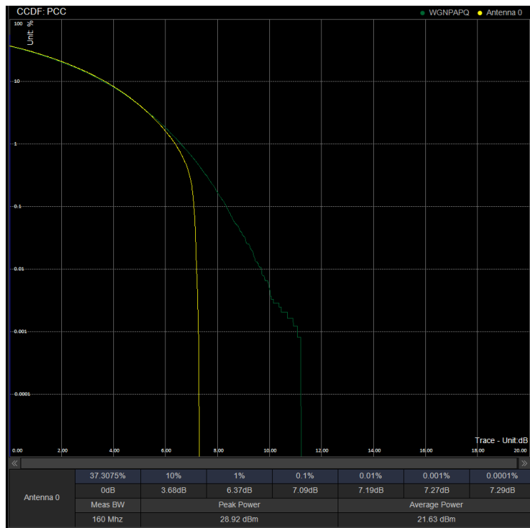
PAPR/PC3\N41\30M CP 534996 100%RB QPSK
