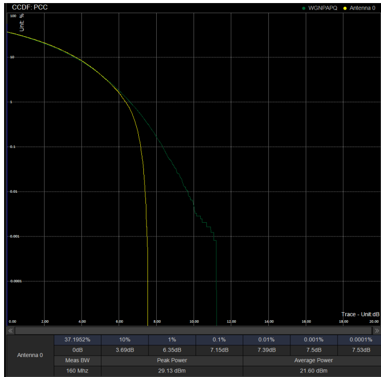
PAPR/PC3\N41\60M CP 531996 100%RB 16QAM
