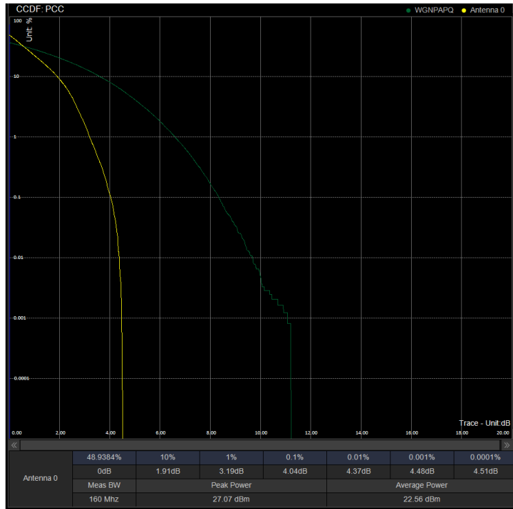
PPR/PC3\N41\20M DFT 518598 100%RB QPSK
