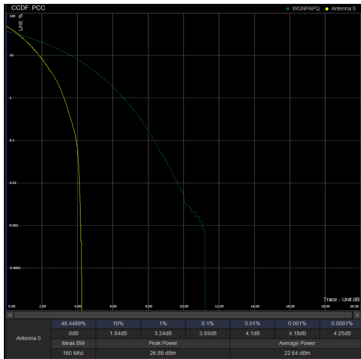
PAPR/PC3\N41\30M DFT 502200 100%RB BPSK
