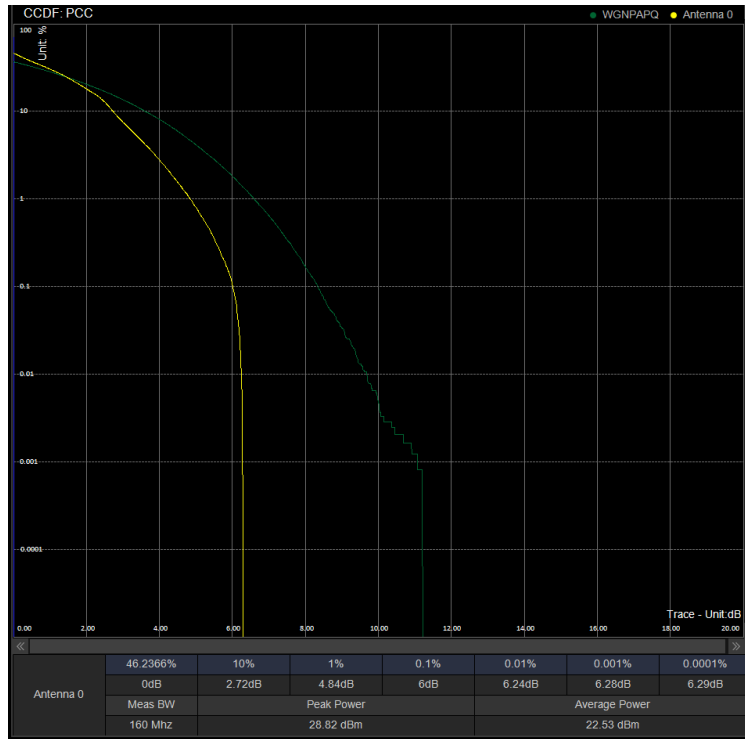
PAPR/PC3\N41\30M DFT 534996 100%RB 16QAM
