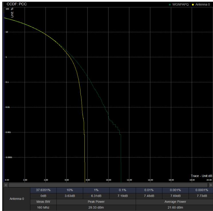
PAPR/PC3\N41\50M CP 504204 100%RB QPSK
