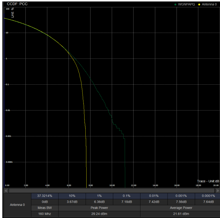
PAPR/PC3\N41\60M CP 531996 100%RB 256QAM
