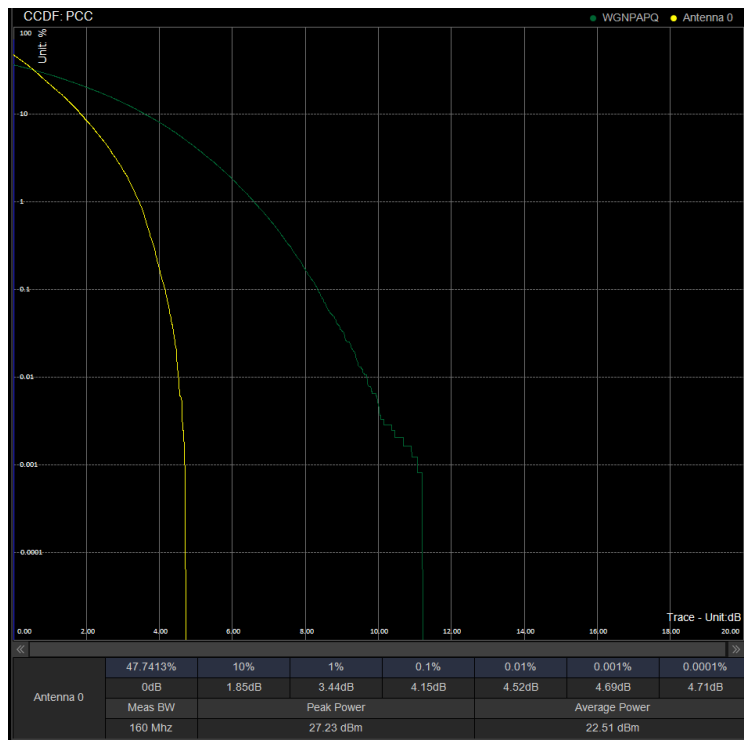
PAPR/PC3\N41\40M DFT 518598 100%RB BPSK
