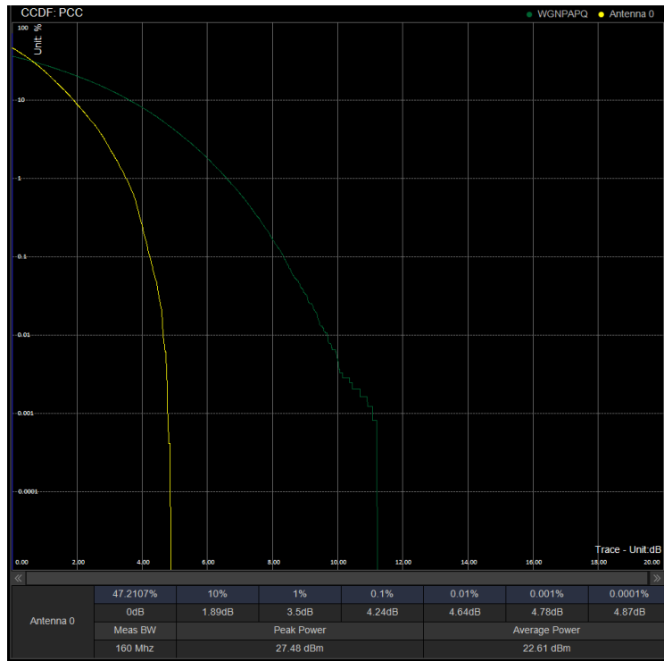
PAPR/PC3\N41\40M DFT 503202 100%RB QPSK
