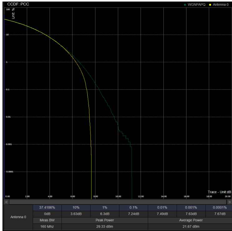
PAPR/PC3\N41\30M CP 502200 100%RB 16QAM
