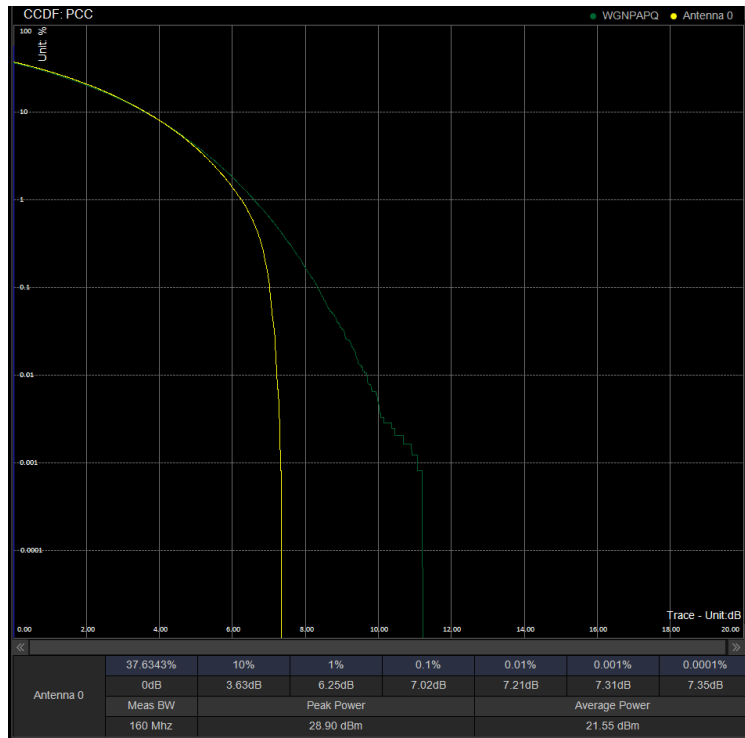
PAPR/PC3\N41\40M CP 518598 100%RB 16QAM
