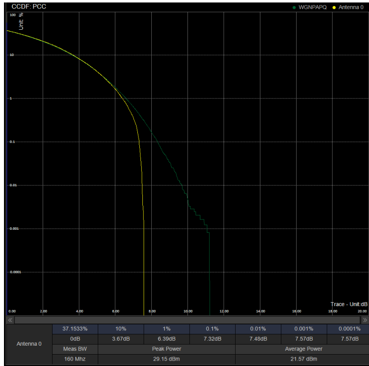
PAPR/PC3\N41\40M CP 534000 100%RB 256QAM
