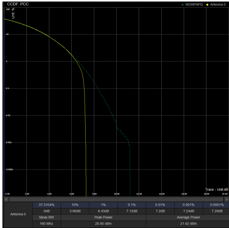
PAPR/PC3\N41\30M CP 534996 100%RB 64QAM
