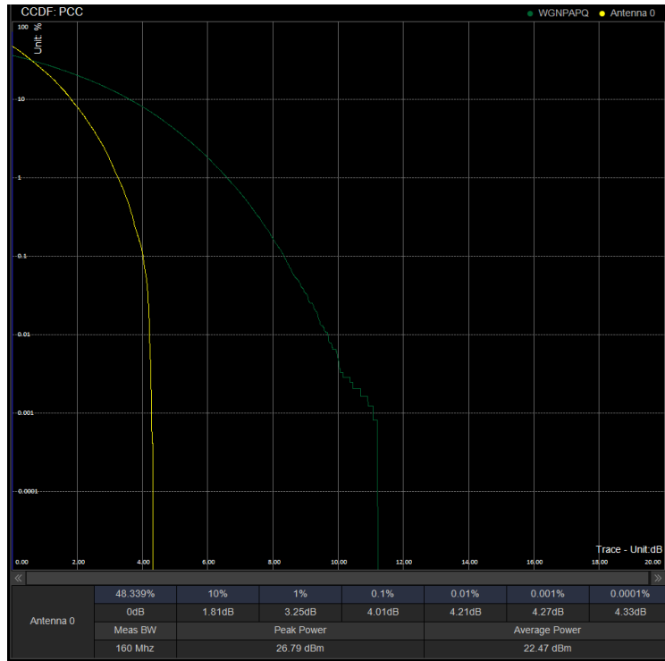
PAPR/PC3\N41\30M DFT 518598 100%RB BPSK
