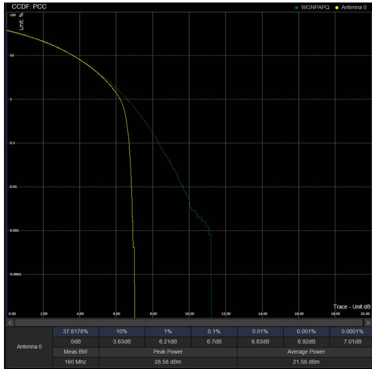
PAPR/PC3\N41\30M CP 518598 100%RB 64QAM
