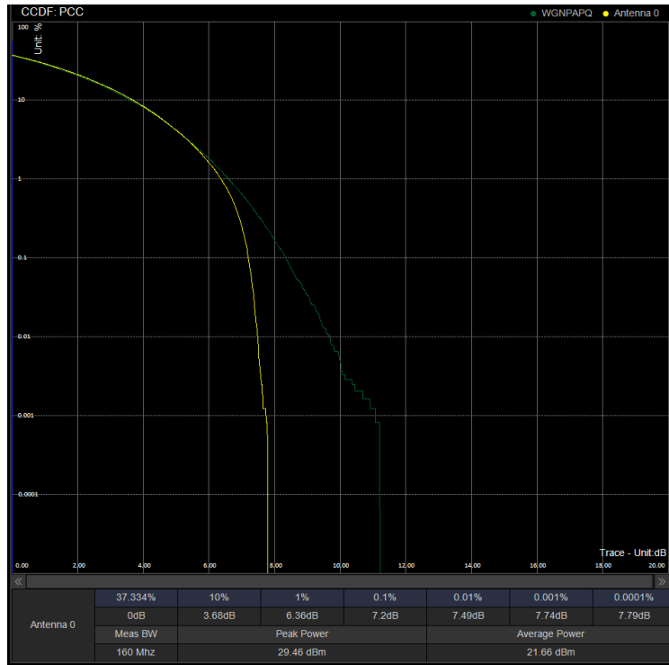
PAPR/PC3\N41\60M CP 531996 100%RB QPSK
