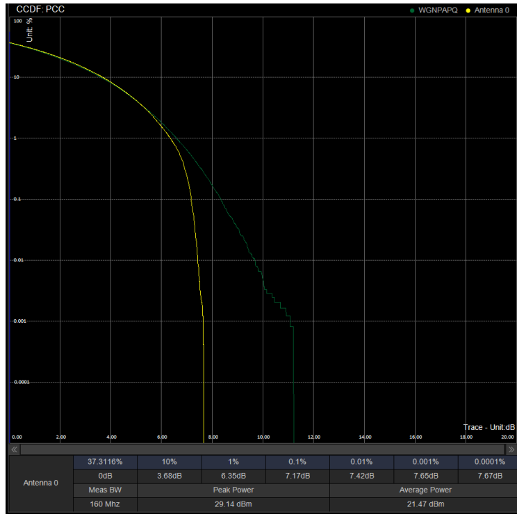
PAPR/PC3\N41\50M CP 532998 100%RB 16QAM
