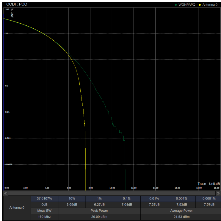
PAPR/PC3\N41\60M CP 518598 100%RB 16QAM
