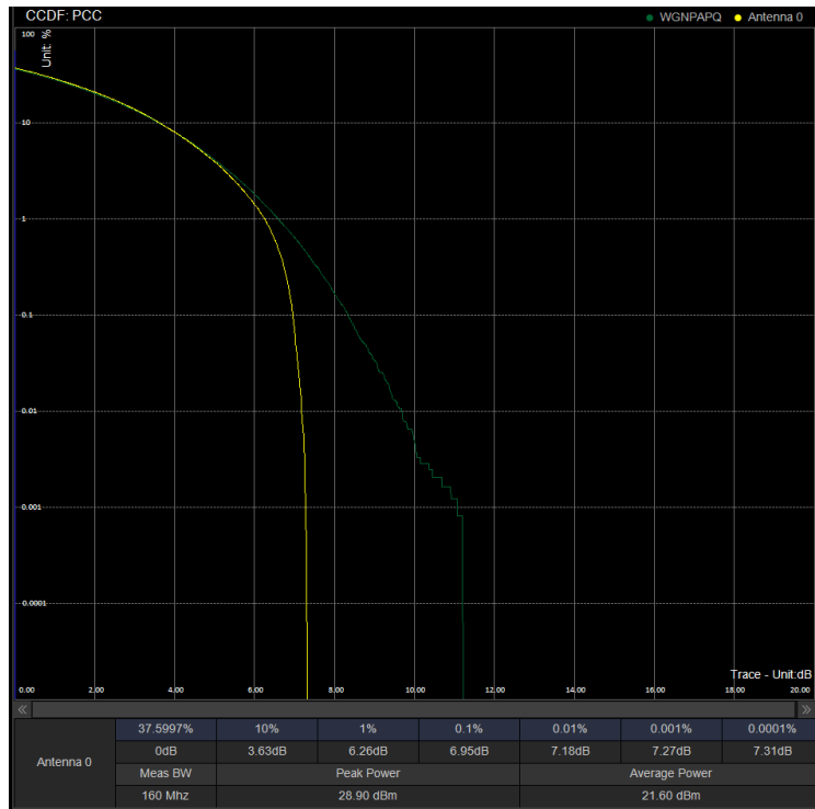
PAPR/PC3\N41\40M CP 518598 100%RB 64QAM
