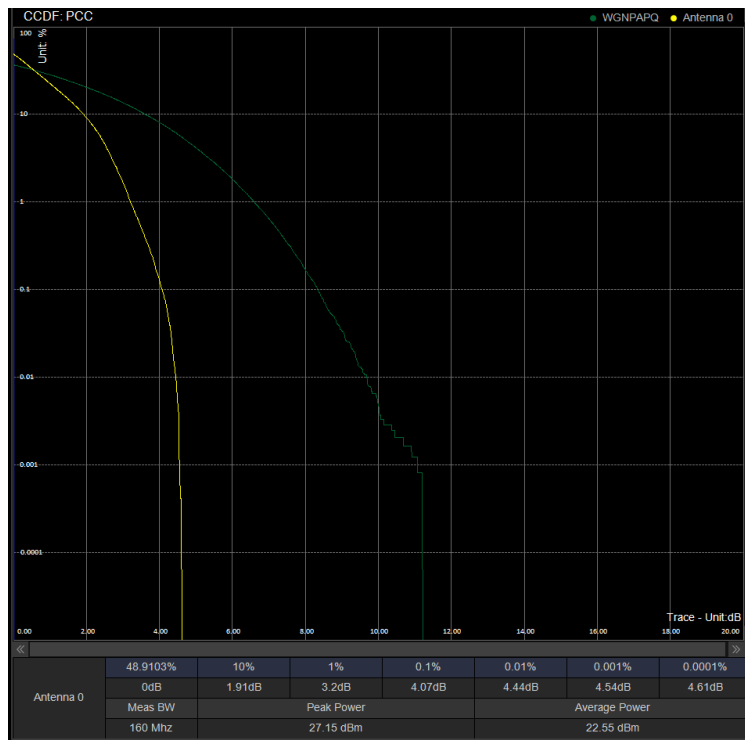
PAPR/PC3\N41\20M DFT 518598 100%RB BPSK
