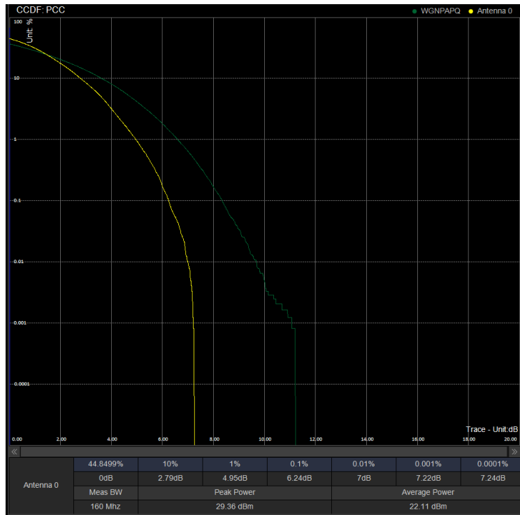
PAPR/PC3\N41\30M DFT 518598 100%RB 64QAM
