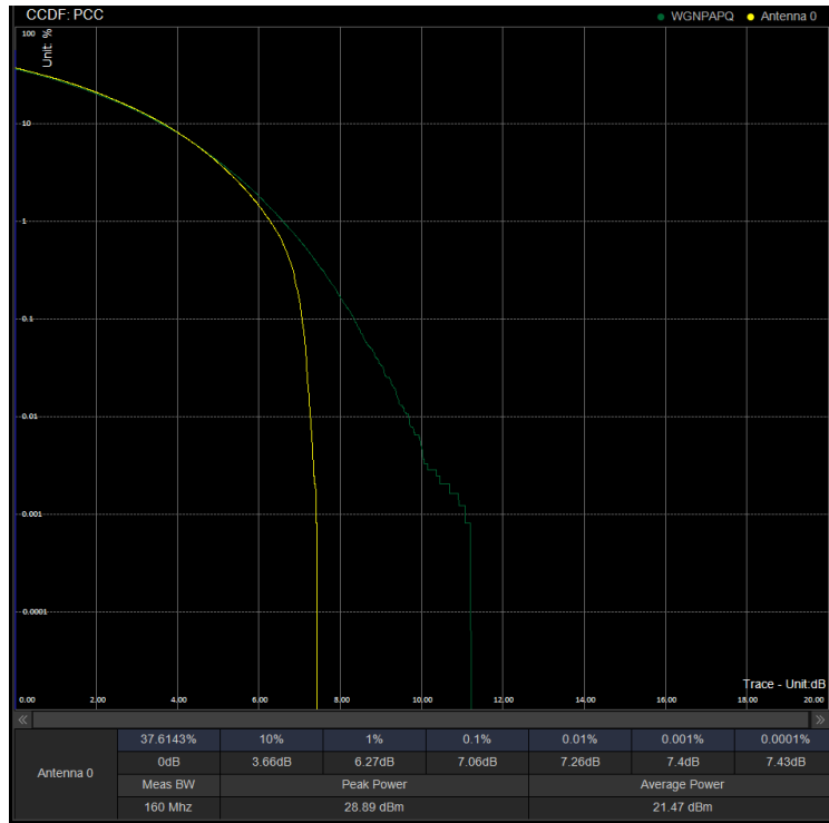
PAPR/PC3\N41\50M CP 518598 100%RB 64QAM
