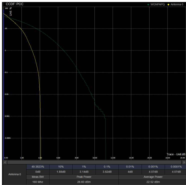
PAPR/PC3\N41\20M DFT 501204 100%RB QPSK
