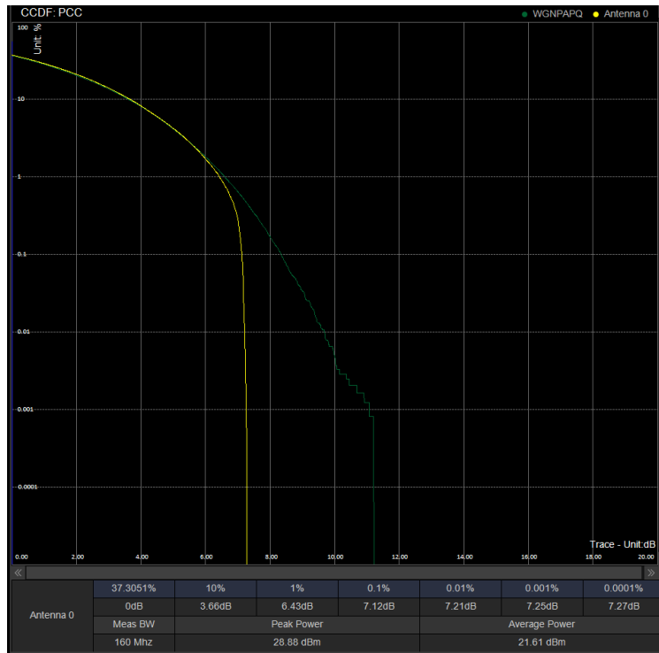
PAPR/PC3\N41\30M CP 534996 100%RB 256QAM
