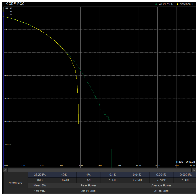
PAPR/PC3\N41\30M CP 518598 100%RB 256QAM
