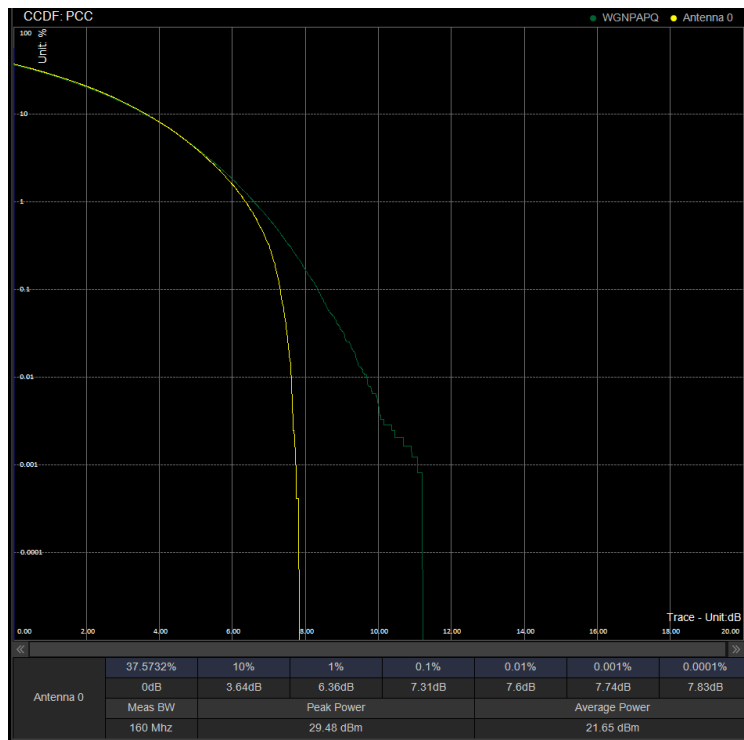
PAPR/PC3\N41\60M CP 505200 100%RB 64QAM
