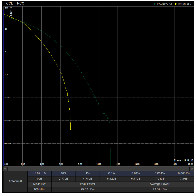
PAPR/PC3\N41\20M DFT 518598 100%RB 16QAM
