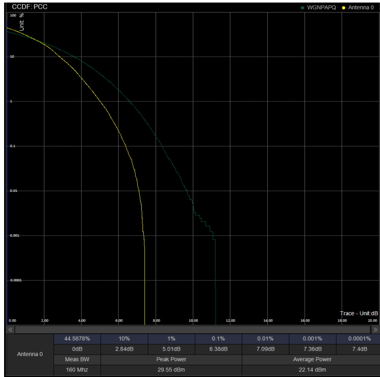
PAPR/PC3\N41\20M DFT 518598 100%RB 64QAM
