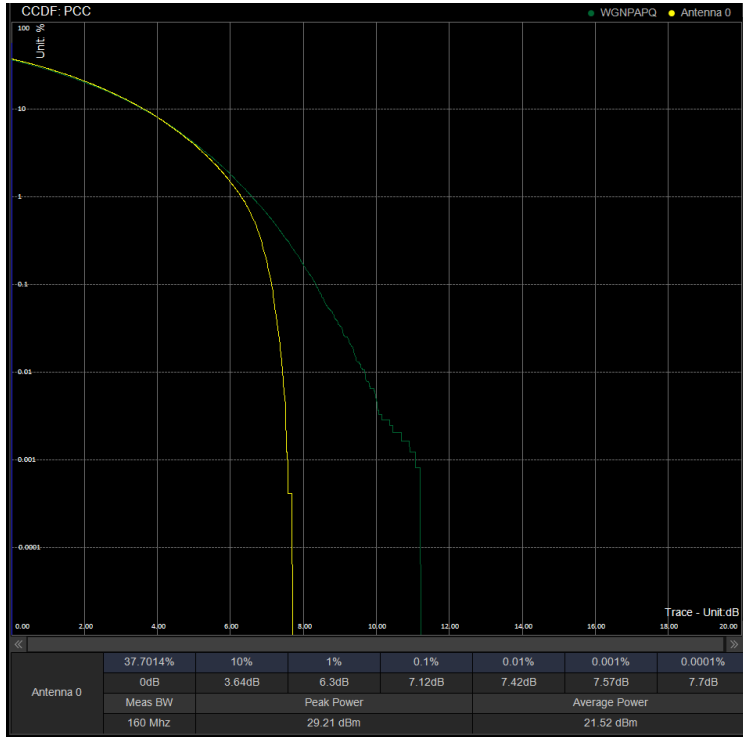
PAPR/PC3\N41\60M CP 518598 100%RB 256QAM
