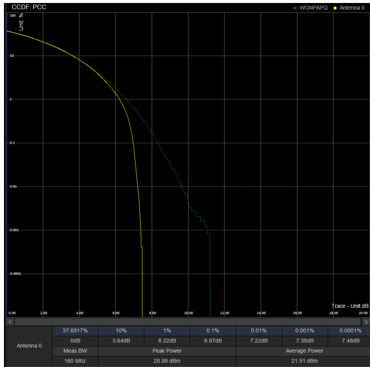
PAPR/PC3\N41\50M CP 518598 100%RB QPSK
