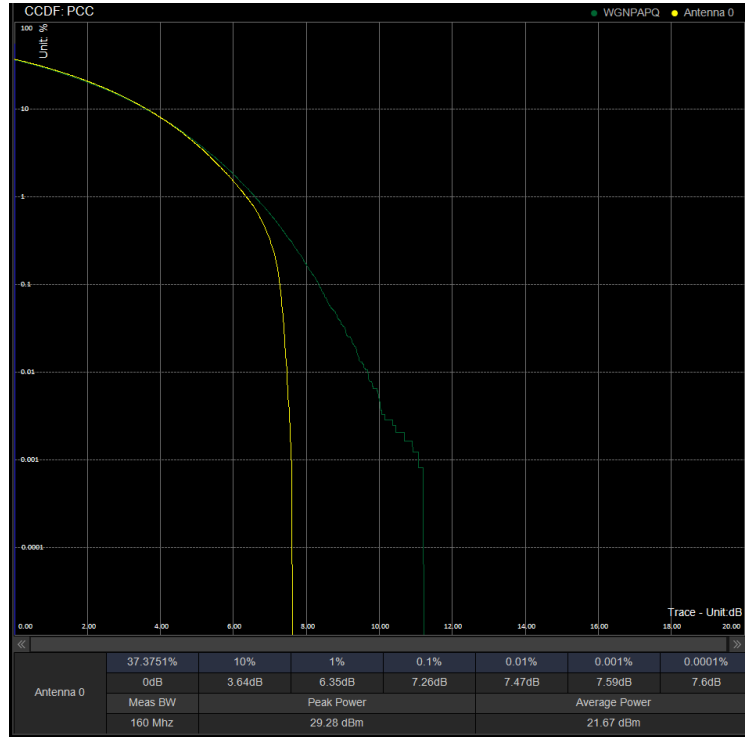
PAPR/PC3\N41\20M CP 501204 100%RB 256QAM
