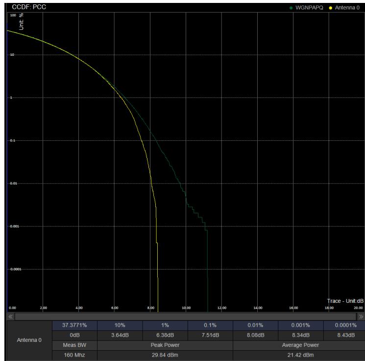
PAPR/PC3\N41\100M CP 518598 100%RB 256QAM
