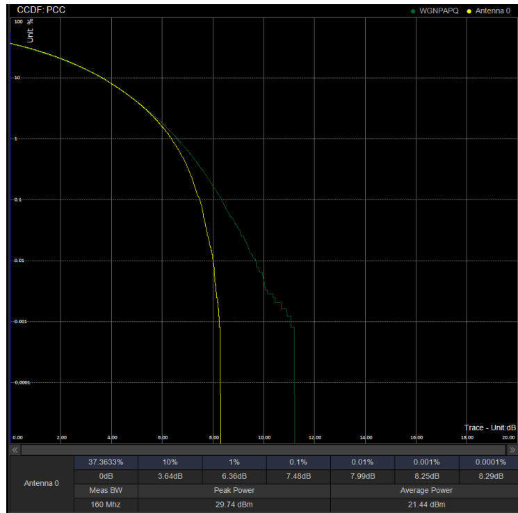
PAPR/PC3\N41\100M CP 528000 100%RB 256QAM
