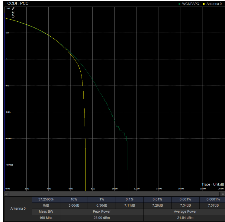
PAPR/PC3\N41\20M CP 518598 100%RB 256QAM
