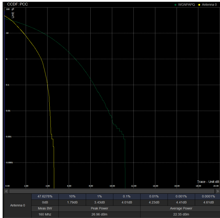
PAPR/PC3\N41\100M DFT 509202 100%RB BPSK
