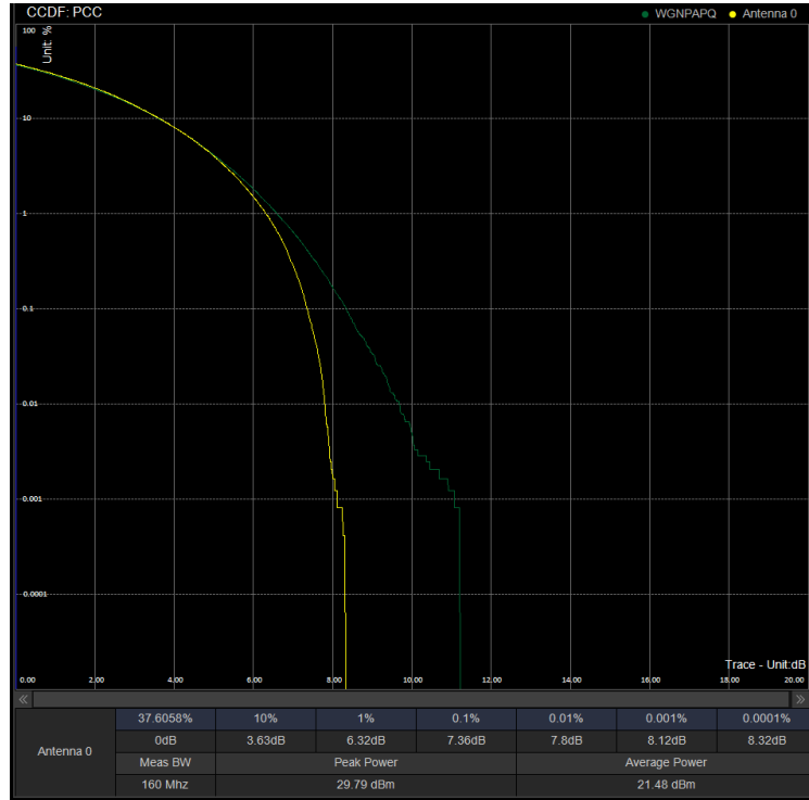
PAPR/PC3\N41\100M CP 528000 100%RB 16QAM
