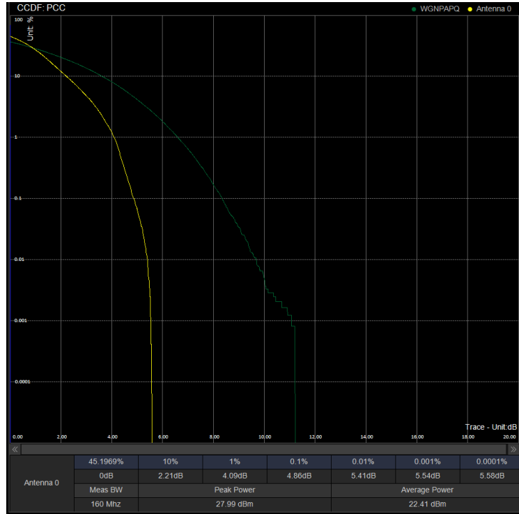
PAPR/PC3\N41\100M DFT 518598 100%RB BPSK
