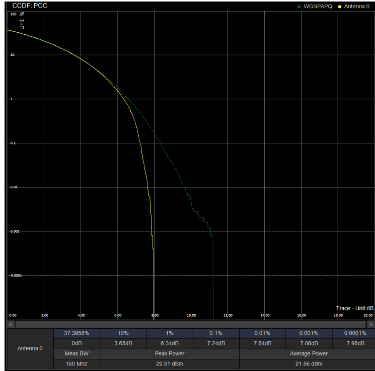
PAPR/PC3\N41\100M CP 509202 100%RB 64QAM
