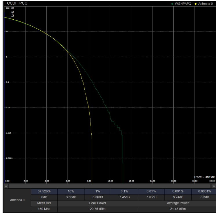
PAPR/PC3\N41\100M CP 518598 100%RB 16QAM
