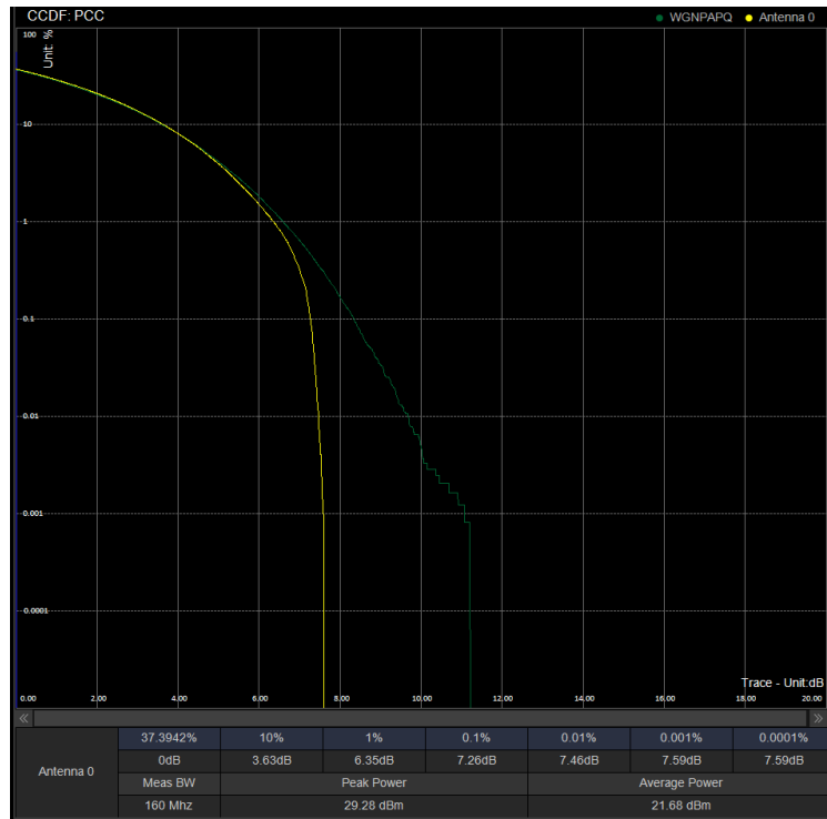
PAPR/PC3\N41\20M CP 501204 100%RB 64QAM
