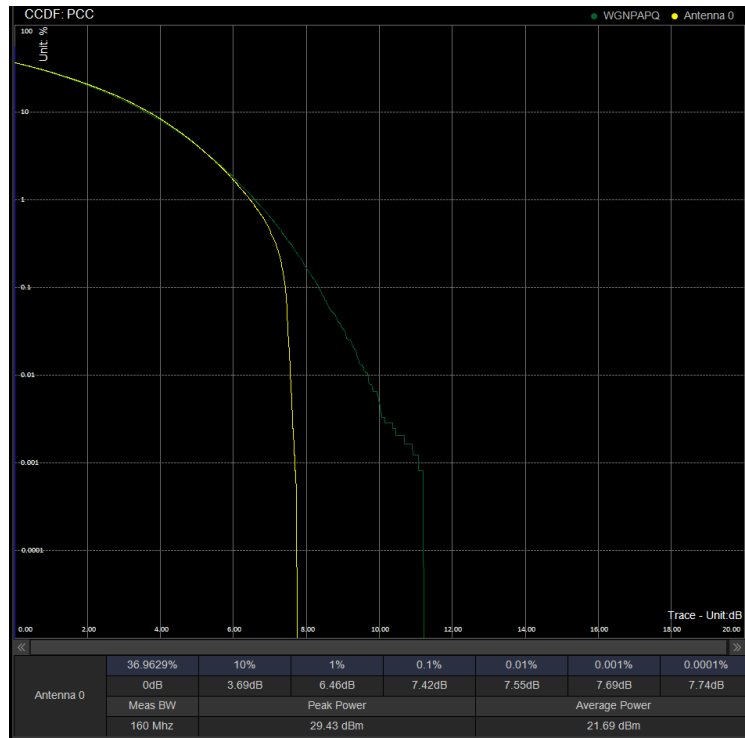
PAPR/PC3\N41\20M CP 535998 100%RB 64QAM
