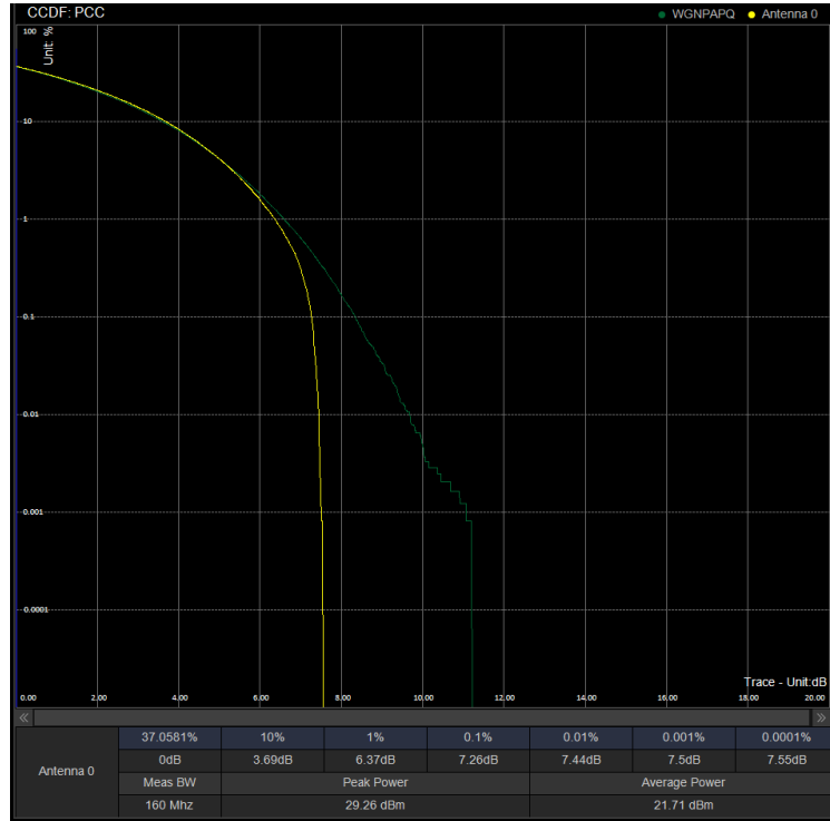
PAPR/PC3\N41\20M CP 535998 100%RB QPSK
