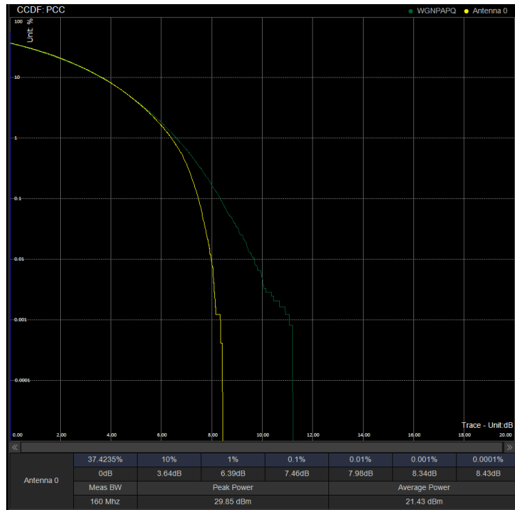
PAPR/PC3\N41\100M CP 528000 100%RB QPSK
