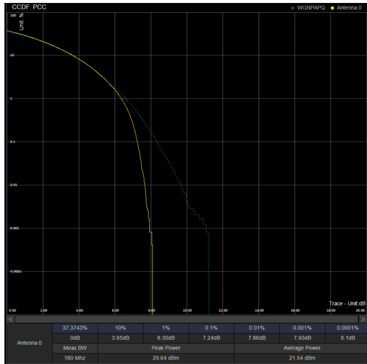
PAPR/PC3\N41\100M CP 509202 100%RB 256QAM
