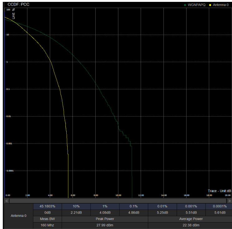
PAPR/PC3\N41\100M DFT 518598 100%RB QPSK
