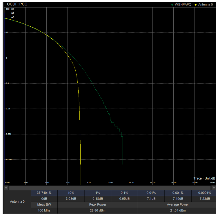
PAPR/PC3\N41\20M CP 518598 100%RB 16QAM
