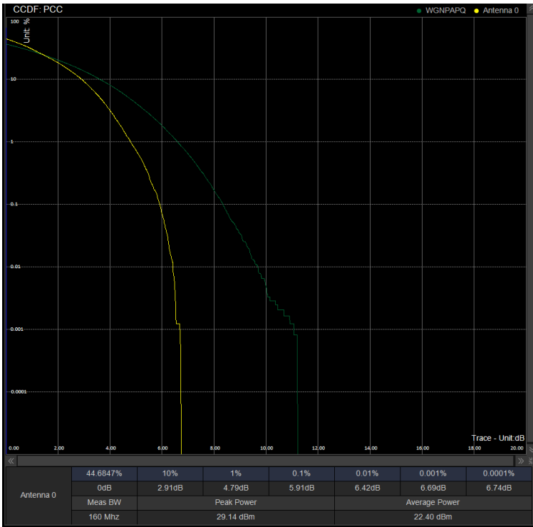
PAPR/PC3\N41\100M DFT 509202 100%RB 16QAM
