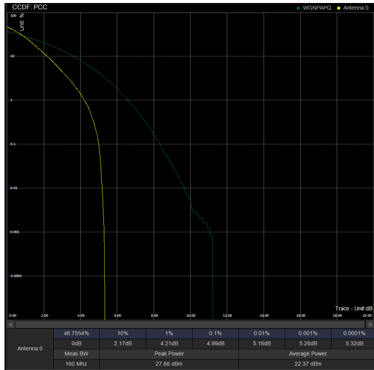
PAPR/PC3\N41\100M DFT 528000 100%RB BPSK
