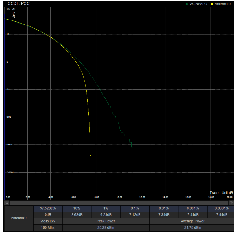
PAPR/PC3\N41\20M CP 501204 100%RB QPSK
