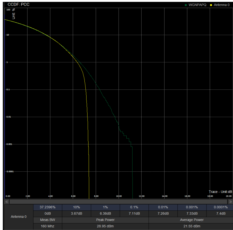
PAPR/PC3\N41\20M CP 518598 100%RB 64QAM
