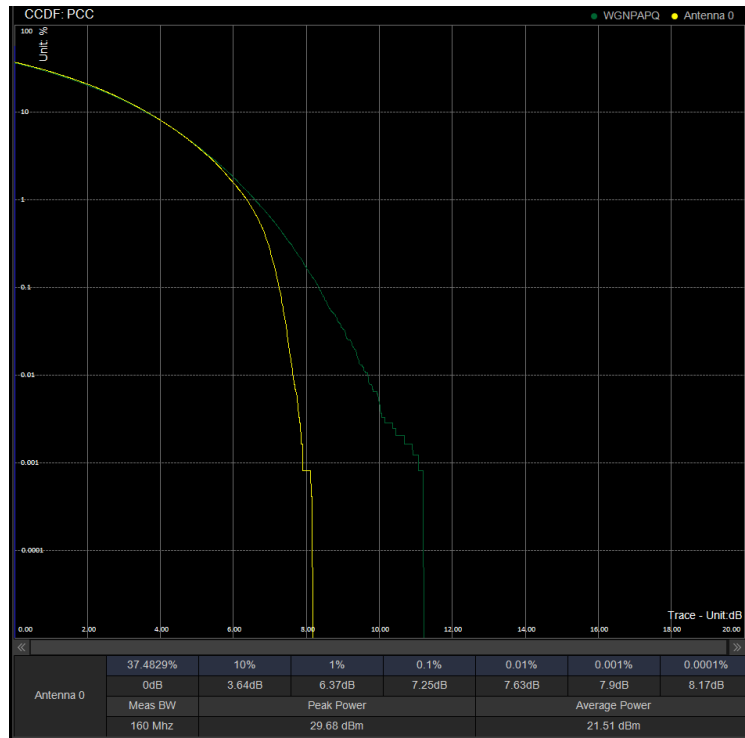
PAPR/PC3\N41\100M CP 509202 100%RB QPSK
