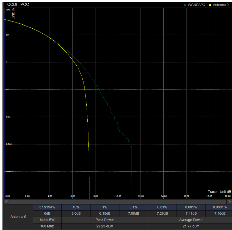
PAPR/PC3\N41\20M CP 501204 100%RB 16QAM
