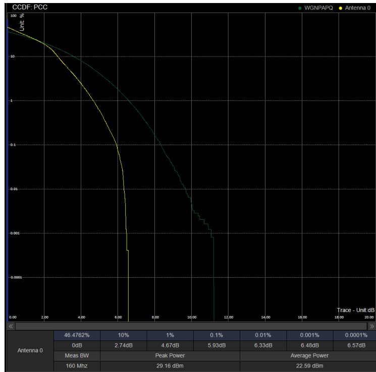
PAPR/PC3\N41\20M DFT 501204 100%RB 16QAM
