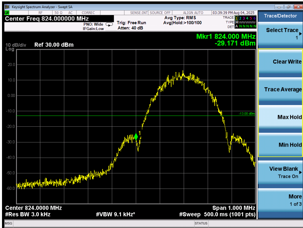
Band edge\GSM850\EGPRS\L
