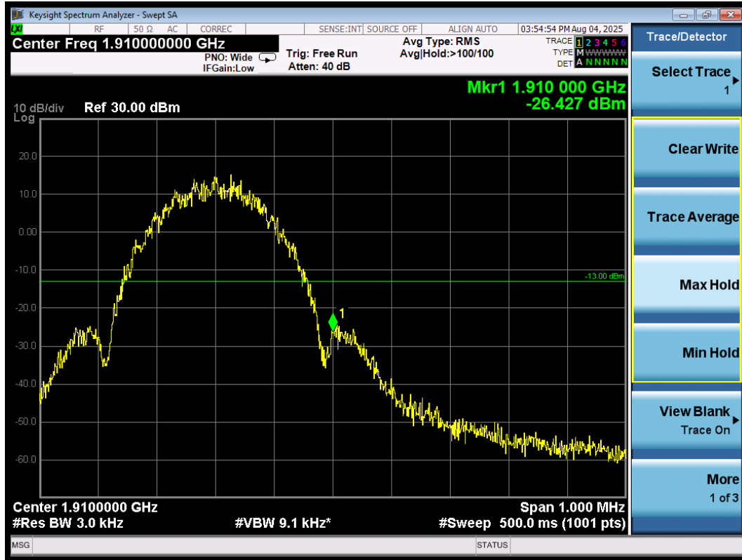
Band edge\GSM1900\EGPRS\H
