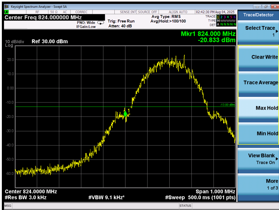
Band edge\GSM850\GSM\L
