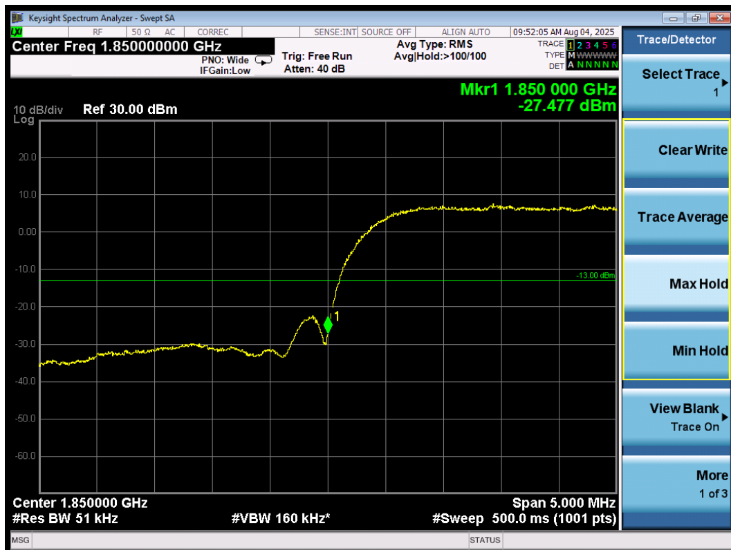
Band edge\B2\L
