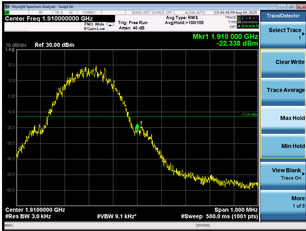
Band edge\GSM1900\GSM\H
