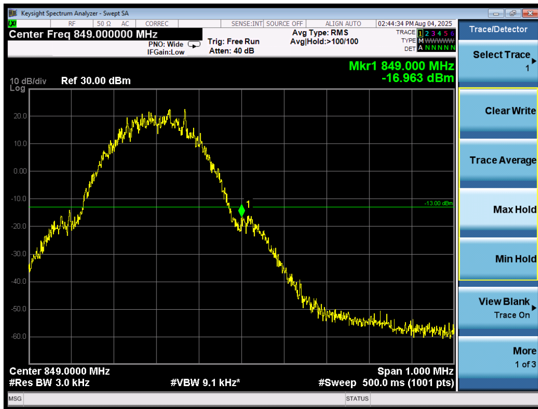
Band edge\GSM850\GSM\H
