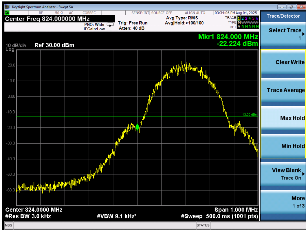
Band edge\GSM850\GPRS\L
