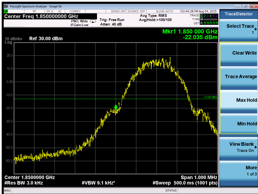
Band edge\GSM1900\GSM\L
