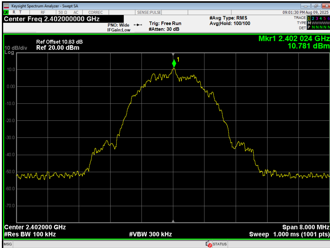
Band Edge BLE (2M) 2402MHz Emission
