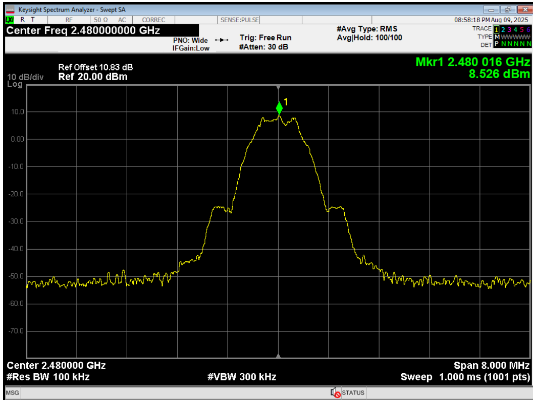
Band Edge BLE (1M)2480MHz Emission
