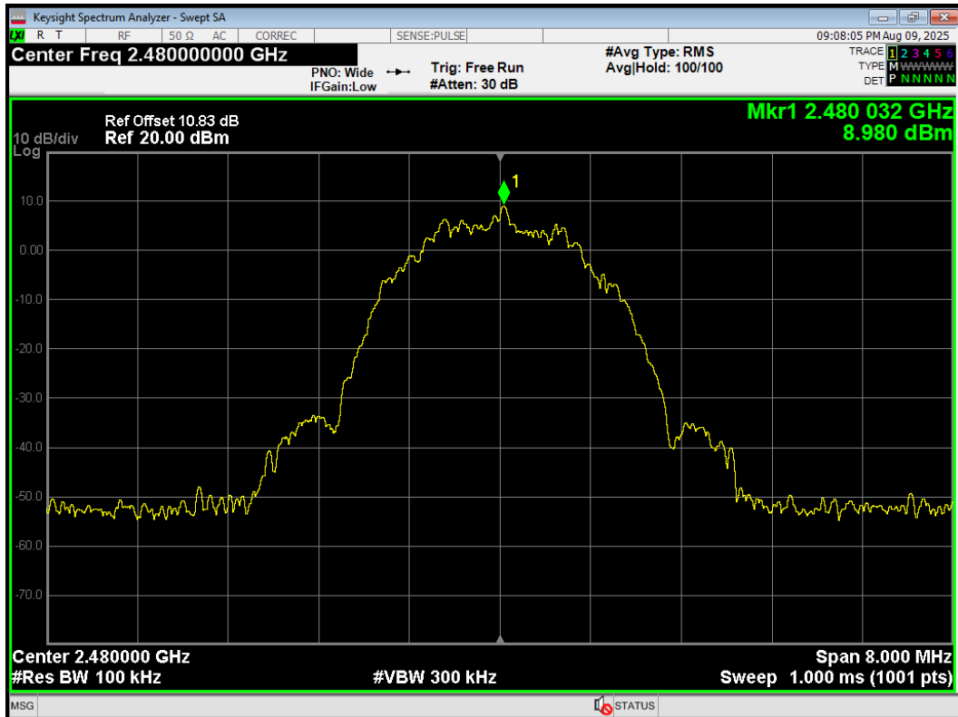
Band Edge BLE (2M) 2480MHz Emission
