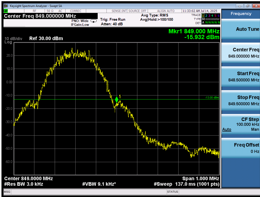
Band Edge\GSM850\H
