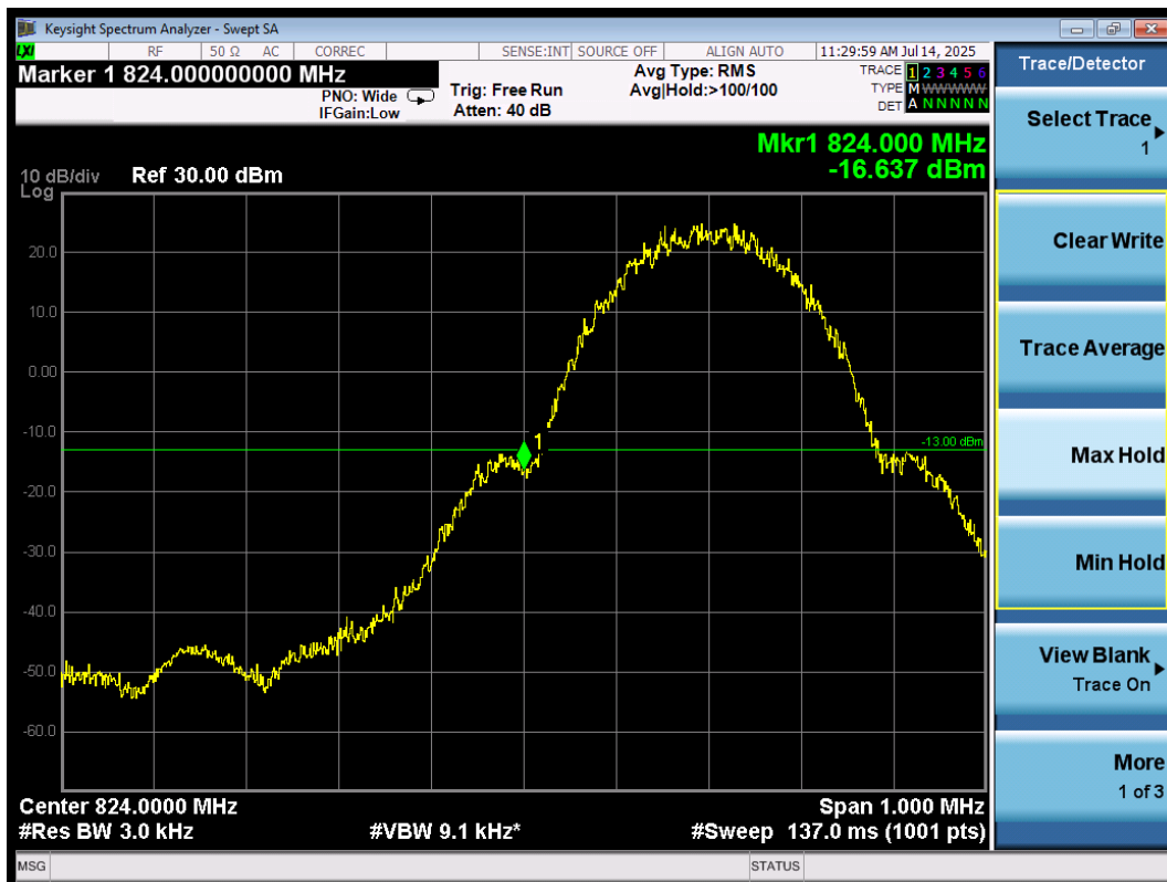
Band Edge\GPRS850\L
