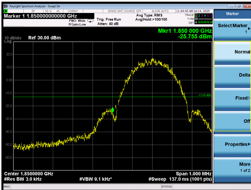
Band Edge\EGPRS1900\L
