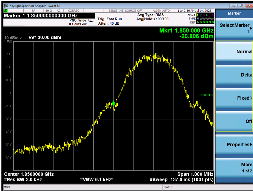
Band Edge\GPRS1900\L
