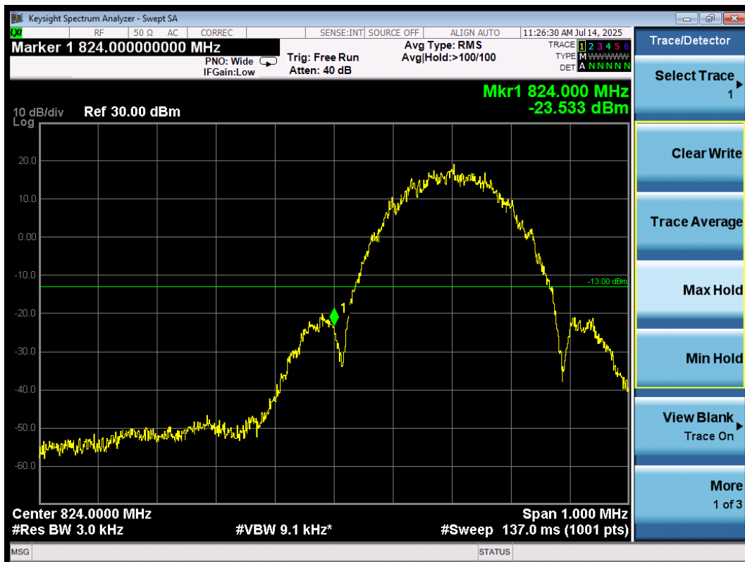
Band Edge\EGPRS850\L
