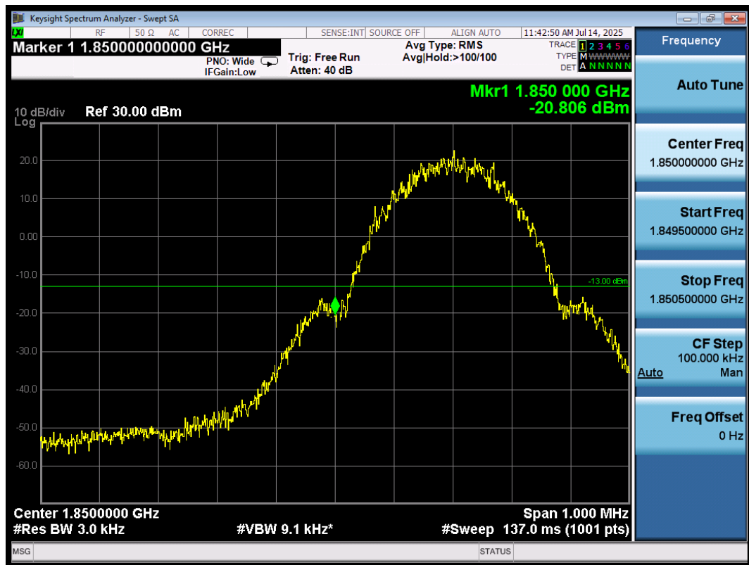
Band Edge\GSM1900\L
