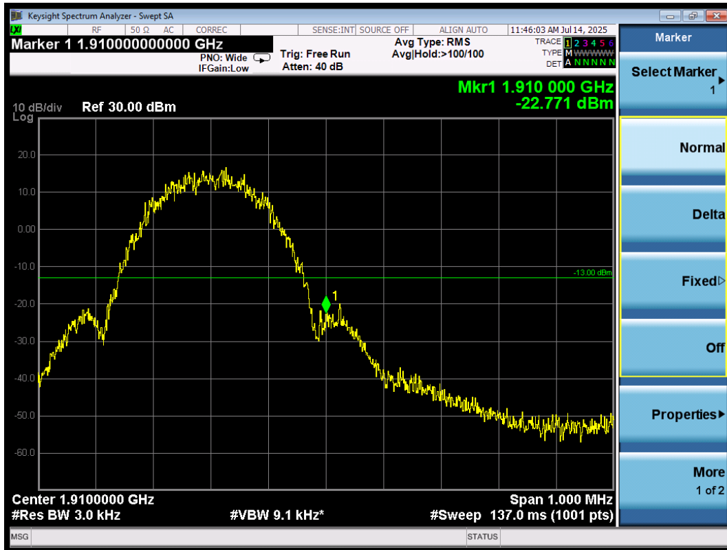
Band Edge\EGPRS1900\H
