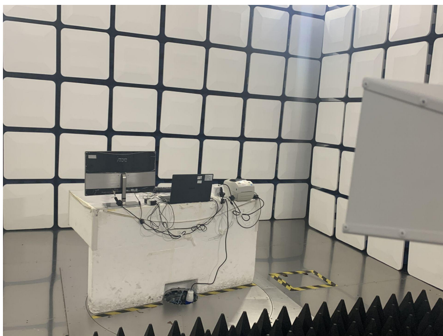
Above 1 GHz(135W)
