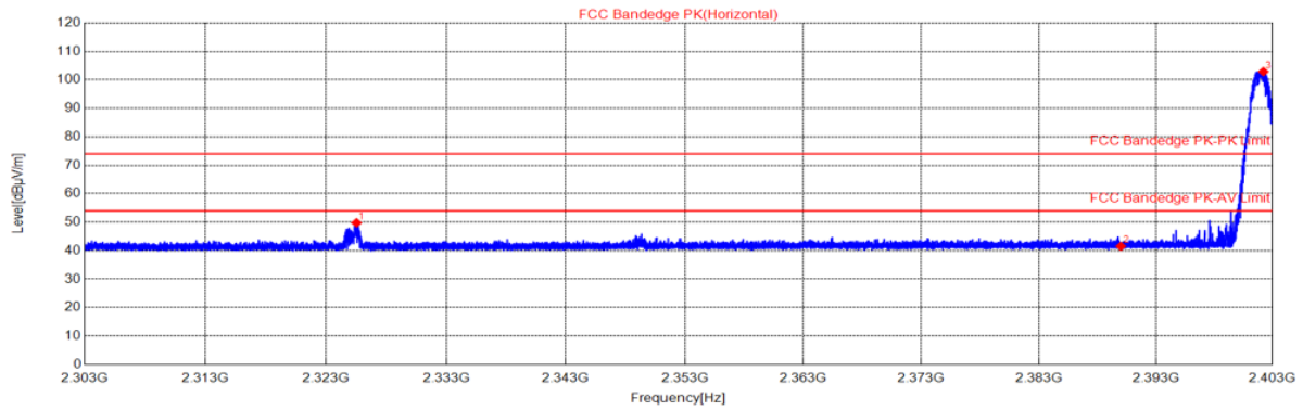
BLE_1M_2402_Ant1/ Horizontal
