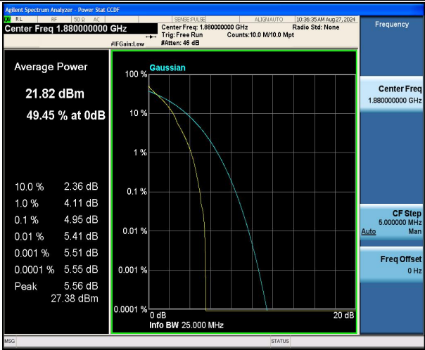
Band2-20MHz-QPSK-18900-1RB#0-PASS
