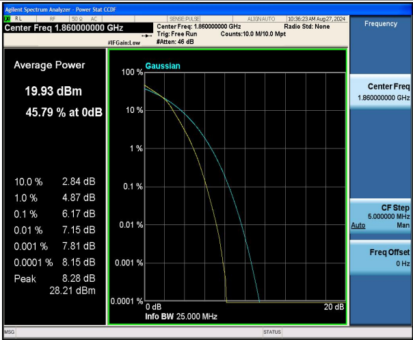
Band2-20MHz-16QAM-18700-100RB#0-PASS
