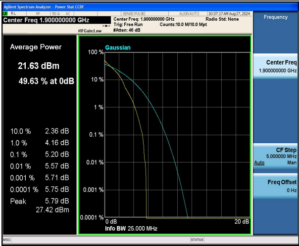
Band2-20MHz-QPSK-19100-1RB#0-PASS
