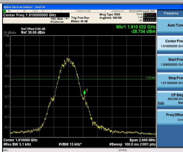
GSM1900-810-0-PASS
