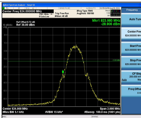
GSM850-128-5-PASS
