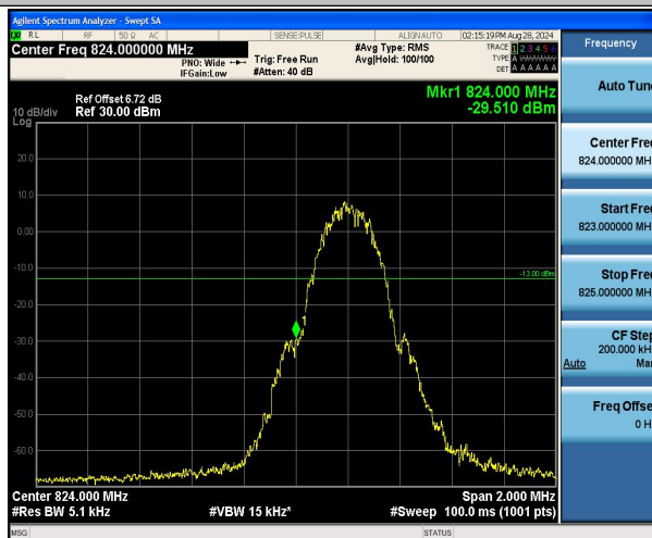
GPRS850-128-5-PASS
