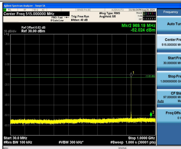
GSM850-190-5-30~1000MHz-PASS
