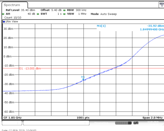
Band25 20MHz QPSK 26140 100RB#0
