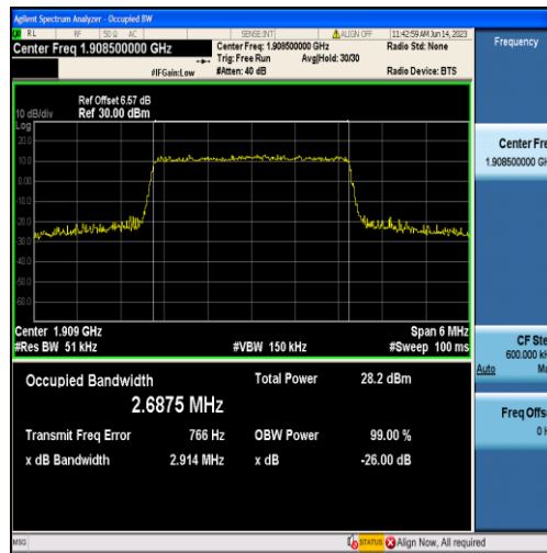
Band2-3MHz-QPSK-19185-15RB#0-2.6875
