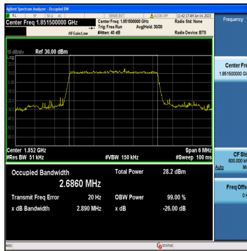
Band2-3MHz-QPSK-18615-15RB#0-2.6860
