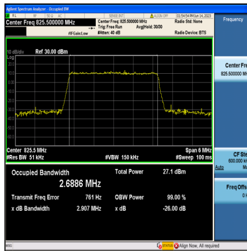
Band5-3MHz-QPSK-20415-15RB#0-2.6886
