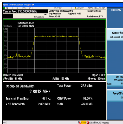
Band5-3MHz-QPSK-20525-15RB#0-2.6818
