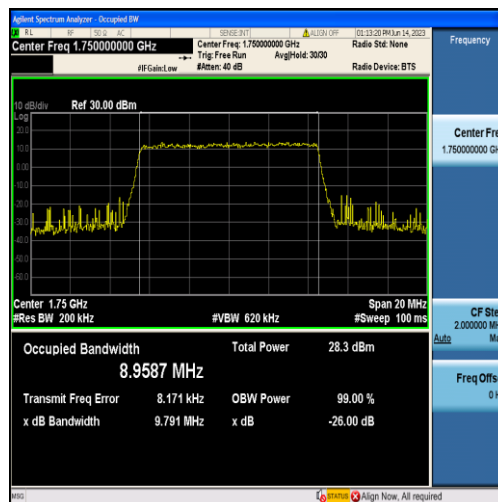
Band4-10MHz-QPSK-20350-50RB#0-8.9587
