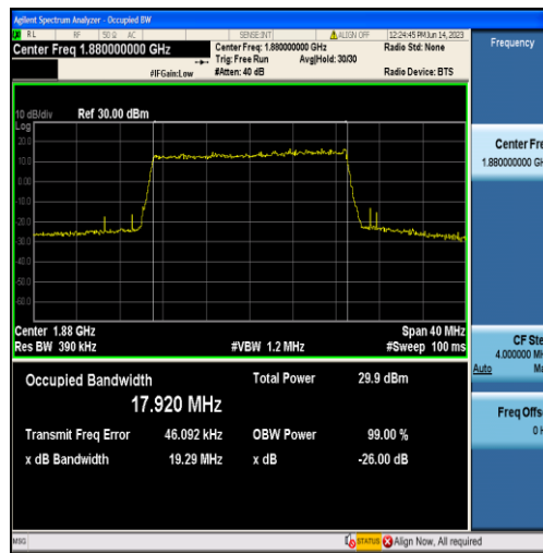
Band2-20MHz-QPSK-18900-100RB#0-17.920
