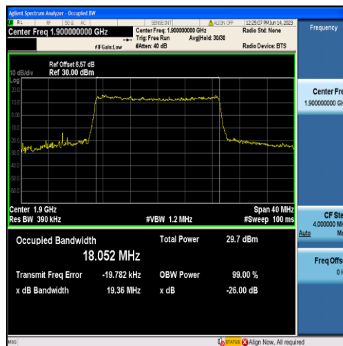
Band2-20MHz-QPSK-19100-100RB#0-18.052
