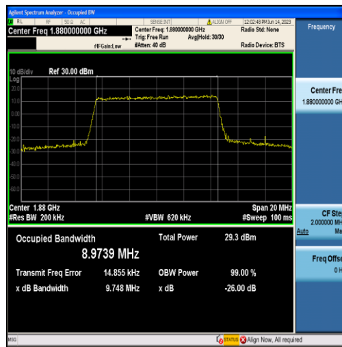
Band2-10MHz-QPSK-18900-50RB#0-8.9739
