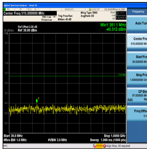
Band4-10MHz-QPSK-20175-50RB#0-Range1:30~1000MHz
