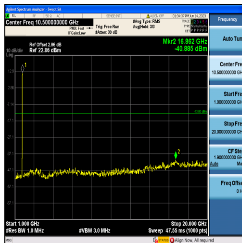
Band4-20MHz-QPSK-20300-100RB#0-Range2:1000~20000MHz
