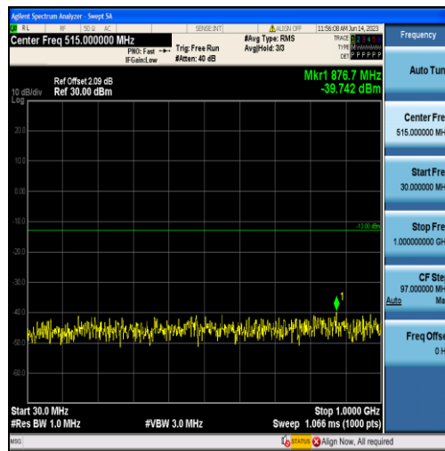
Band2-5MHz-QPSK-18900-25RB#0-Range1:30~1000MHz
