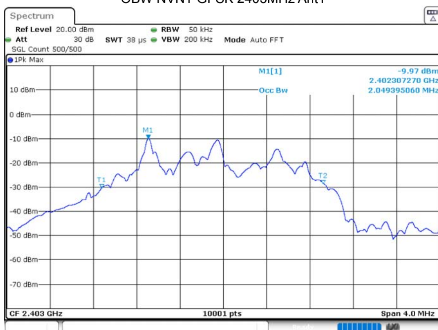
OBW NVNT GFSK 2403MHz Ant1
