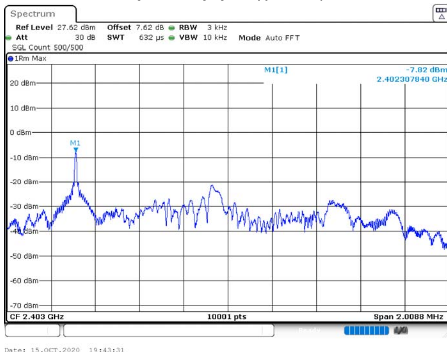
PSD NVNT GFSK 2403MHz Ant1
