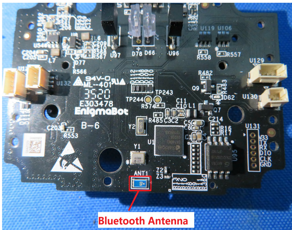
(12) EUT Photo
