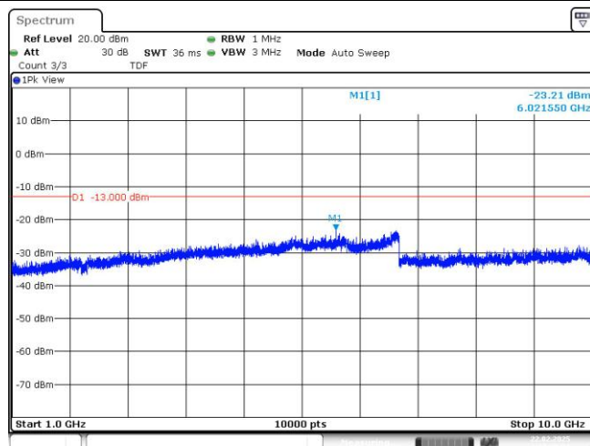
Band14-5MHz-QPSK-23305-25RB#0-Range2:1000~10000MHz
