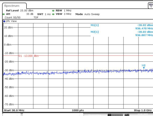
Band14-5MHz-QPSK-23330-25RB#0-Range1:30~1000MHz
