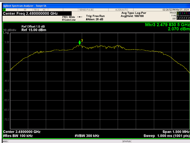
\pi/4 -DQPSK_2480_30~25000
