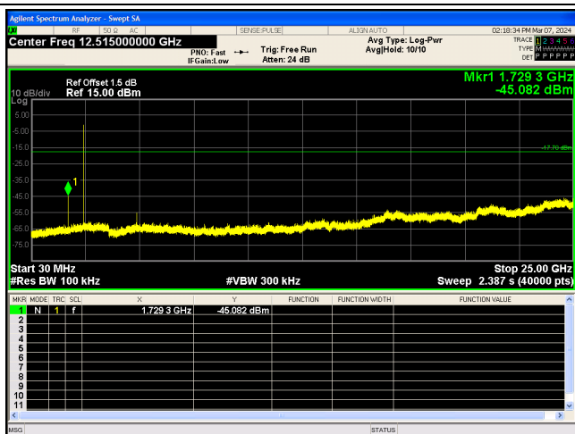
\pi/4 -DQPSK_2480_0~Reference
