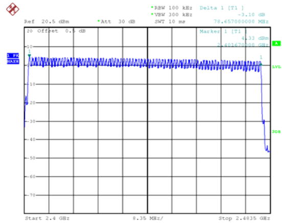
Modulation: \pi/4 DQPSK
