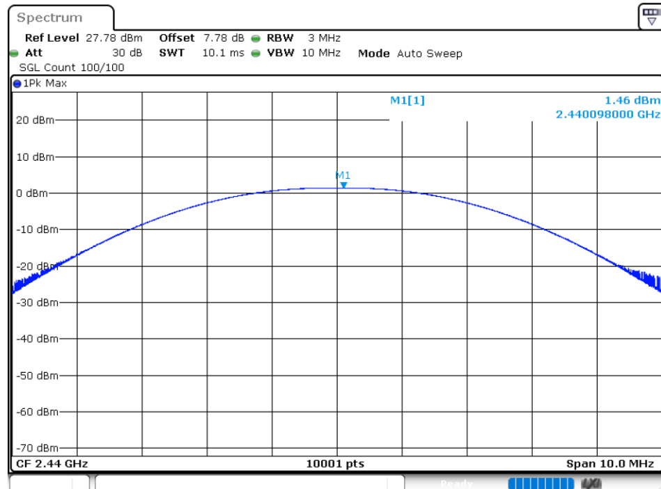
Power NVNT BLE 2440MHz Ant1
