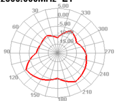
2500.000MHz E1
