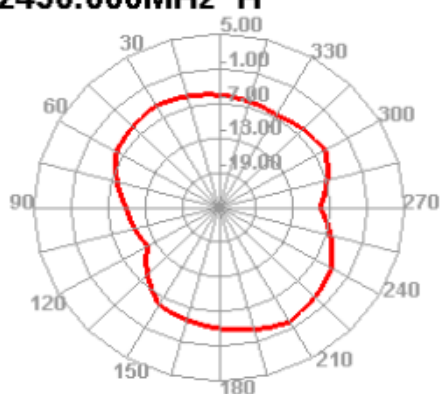
2450.000MHz H
