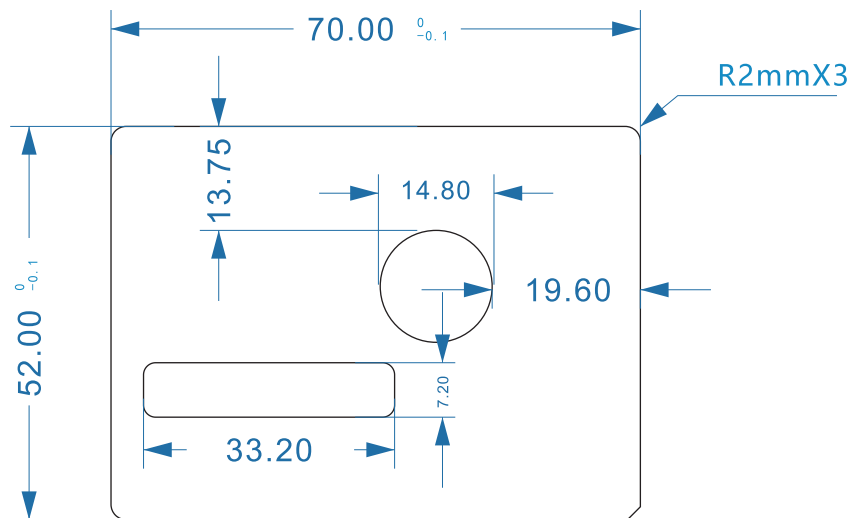
(尺寸图)
