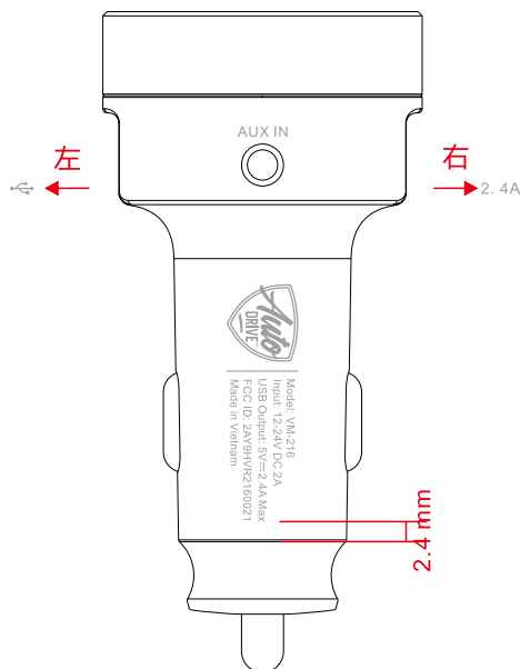
正视图
