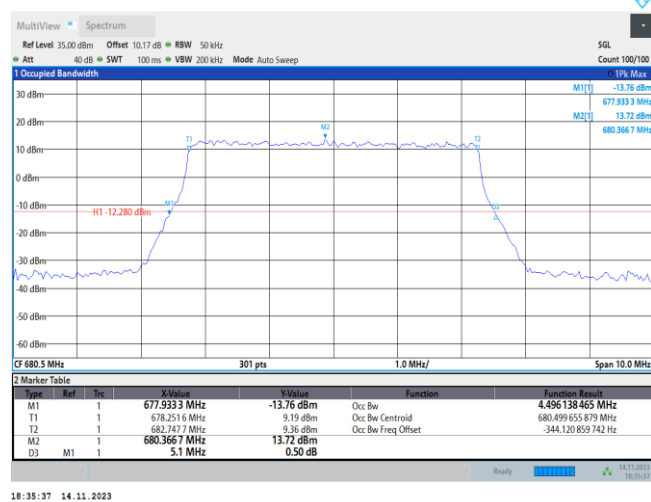
Band71-5MHz-QPSK-133297-25RB#0
